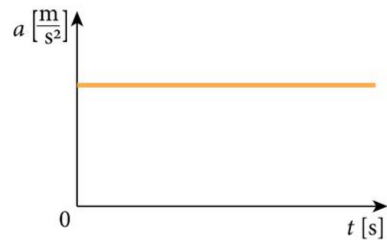
Wykres zależności przyspieszenia od czasu dla ruchu jednostajnie przyspieszonego.
