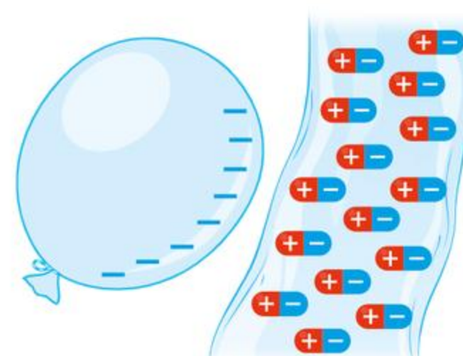
Balonik i stróżka wody.
