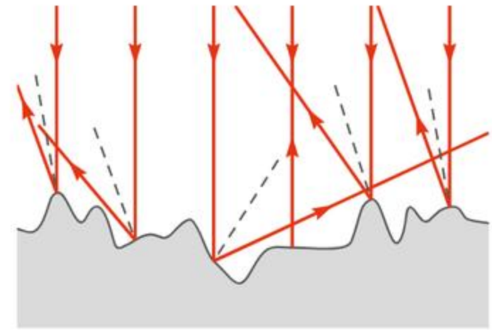
Schemat rozproszenia światła padającego na nierówną (szorstką) powierzchnię.
