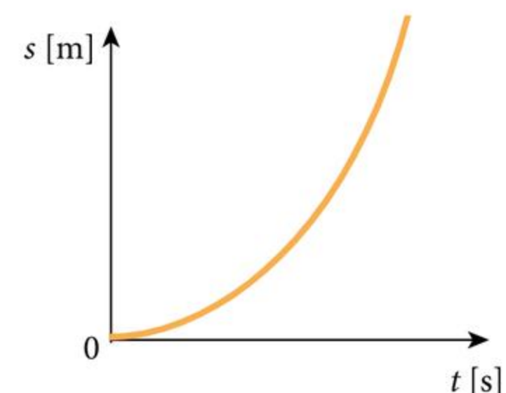
Wykres zależności drogi od czasu dla ruchu jednostajnie przyspieszonego, gdy prędkość początkowa jest równa zero.
