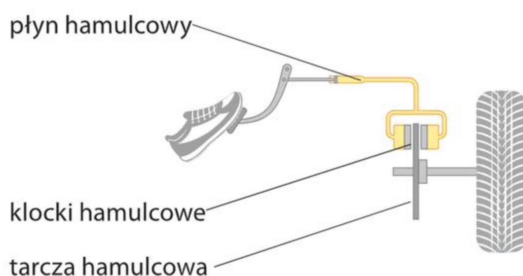
Schemat zasady działania hamulca hydraulicznego.
