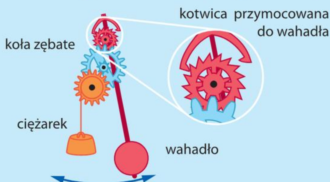
Uproszczony mechanizm działania zegara wahadłowego.
