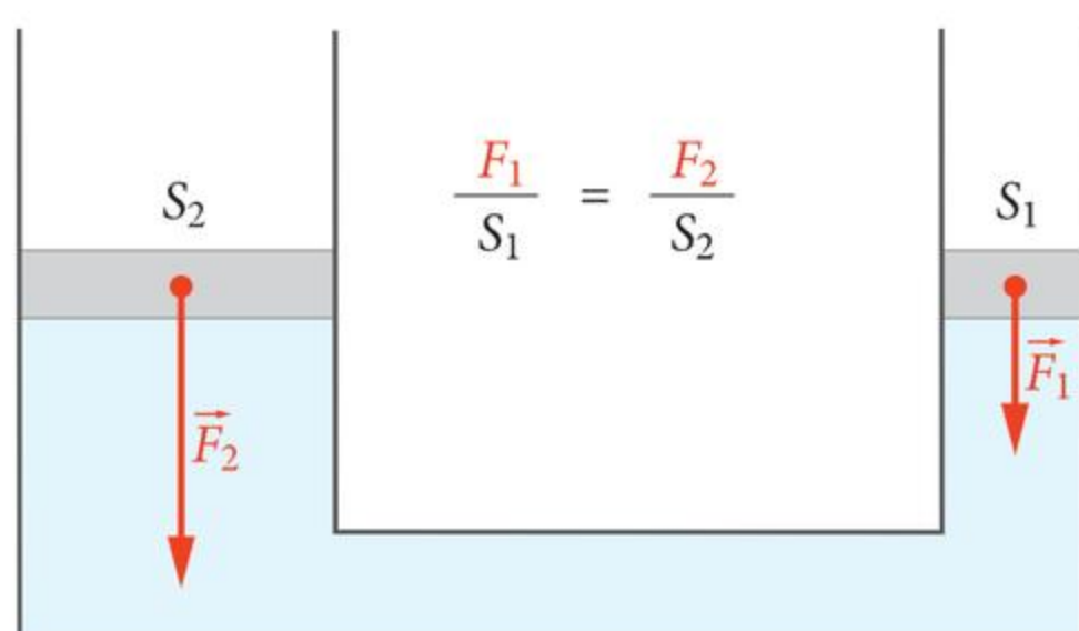
Schemat prasy hydraulicznej.
