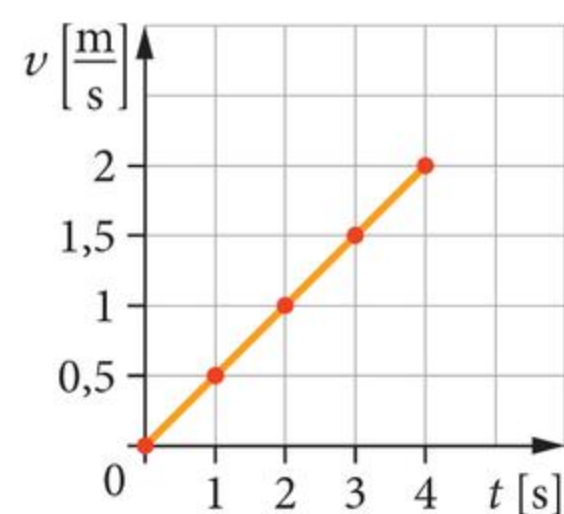
Wykres zależności prędkości od czasu dla pociągu.
