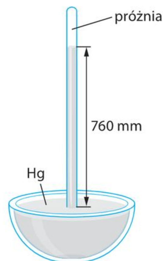
Schemat doświadczenia Torricellego.
