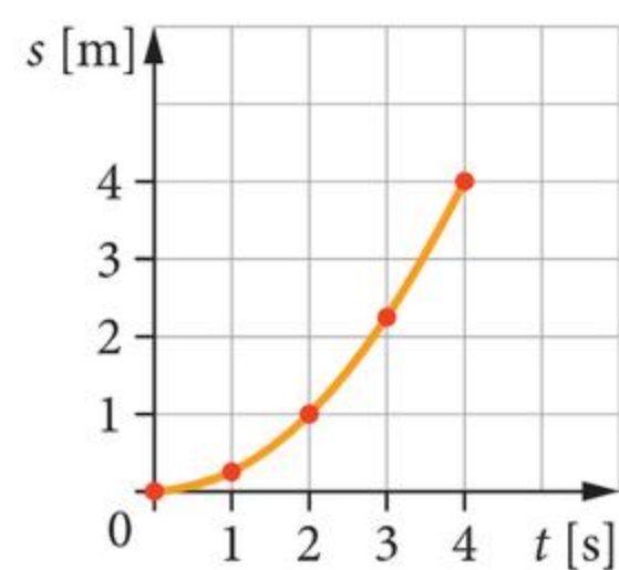
Wykres zależności drogi od czasu dla pociągu poruszającego się z przyspieszeniem 0,5 \frac{\text{m}}{\text{s}^2} .
