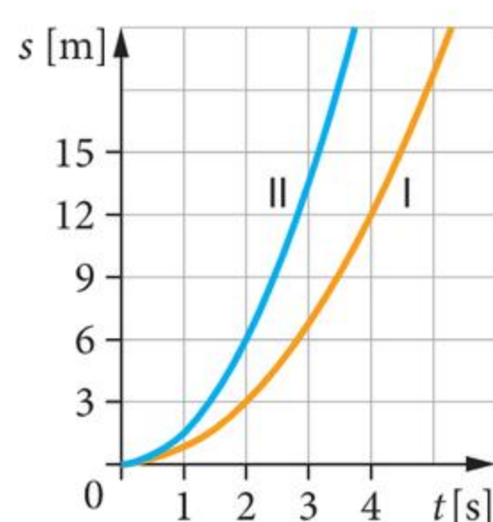
Wykres zależności drogi od czasu w ruchu jednostajnie przyspieszonym ( v_p = 0 \frac{\text{m}}{\text{s}} ).
