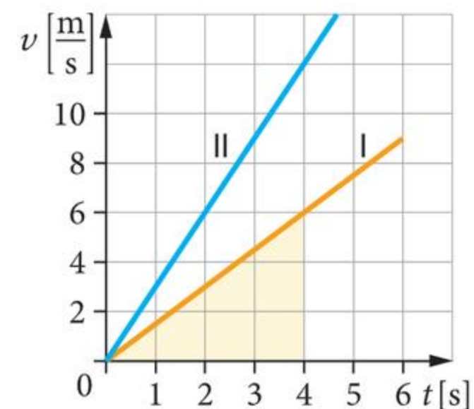
Wykres zależności prędkości od czasu w ruchu jednostajnie przyspieszonym ( v_p = 0 \frac{\text{m}}{\text{s}} ).
