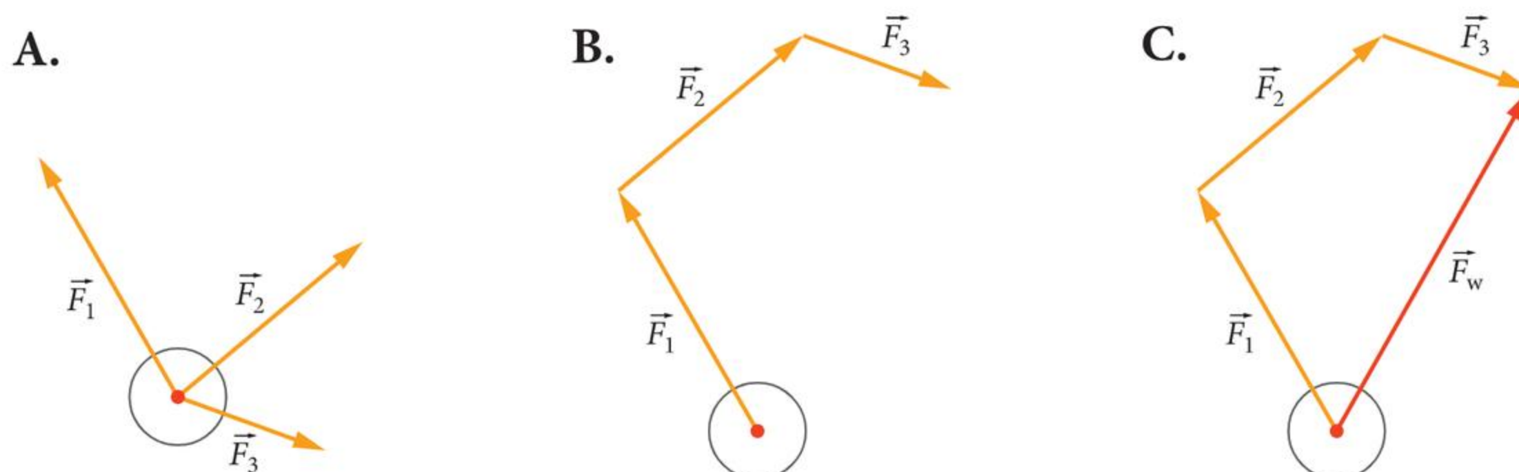
Etapy wyznaczania siły wypadkowej kilku sił składowych metodą łańcucha wektorów.
