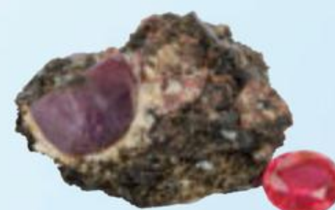
twardość 9 rubin
