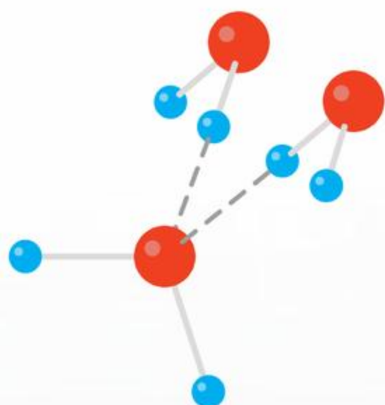
Wiązania wodorowe (zaznaczone linią przerywaną)
