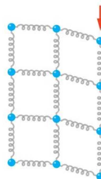
Drgania atomów i cząsteczek w ciele stałym rozchodzą się podobnie jak drgania kulek połączonych sprężynkami.
