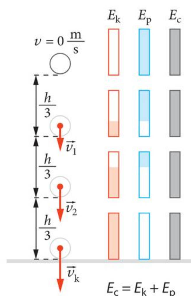
Przemiany energii podczas swobodnego spadania ciała z wysokości h .
