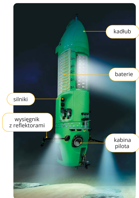
Rys. 12.1. Batyskaf J. Camerona z zaznaczonymi najważniejszymi elementami
