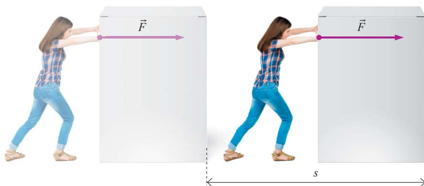
Rys. 26.1. Siła powodująca przesunięcie ciała wykonuje pracę mechaniczną.
