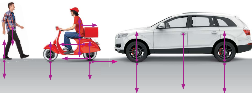
Rys. 4.7. Siły wokół nas
