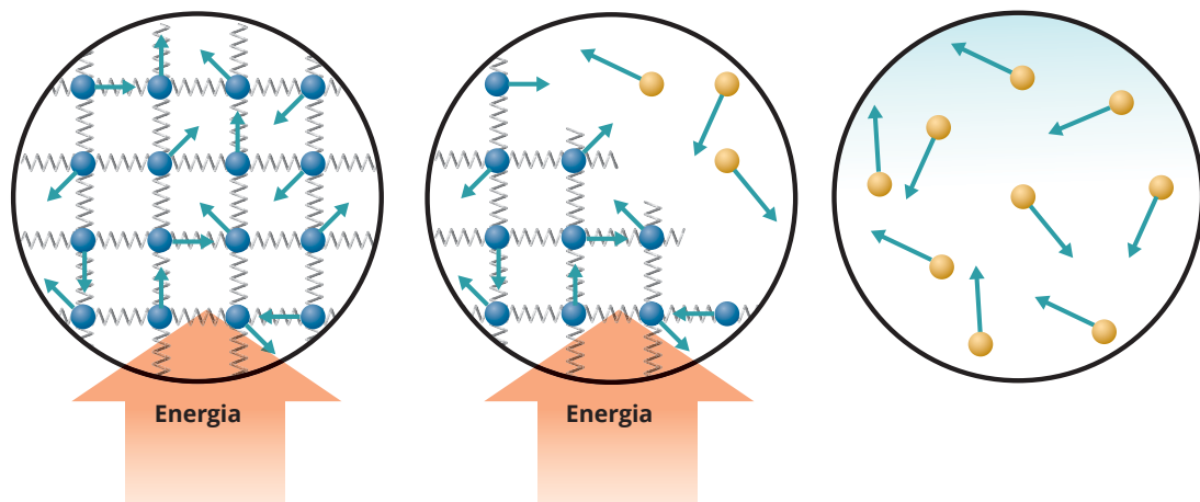
Rys. 36.6. Topnienie, czyli przejście ze stanu stałego w cieki, przedstawione w modelu kinetyczno-molekularnym
