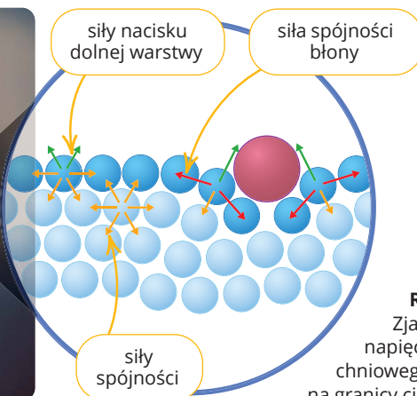
Rys. 7.2. Krople wody powstają dzięki działaniu sił spójności.
