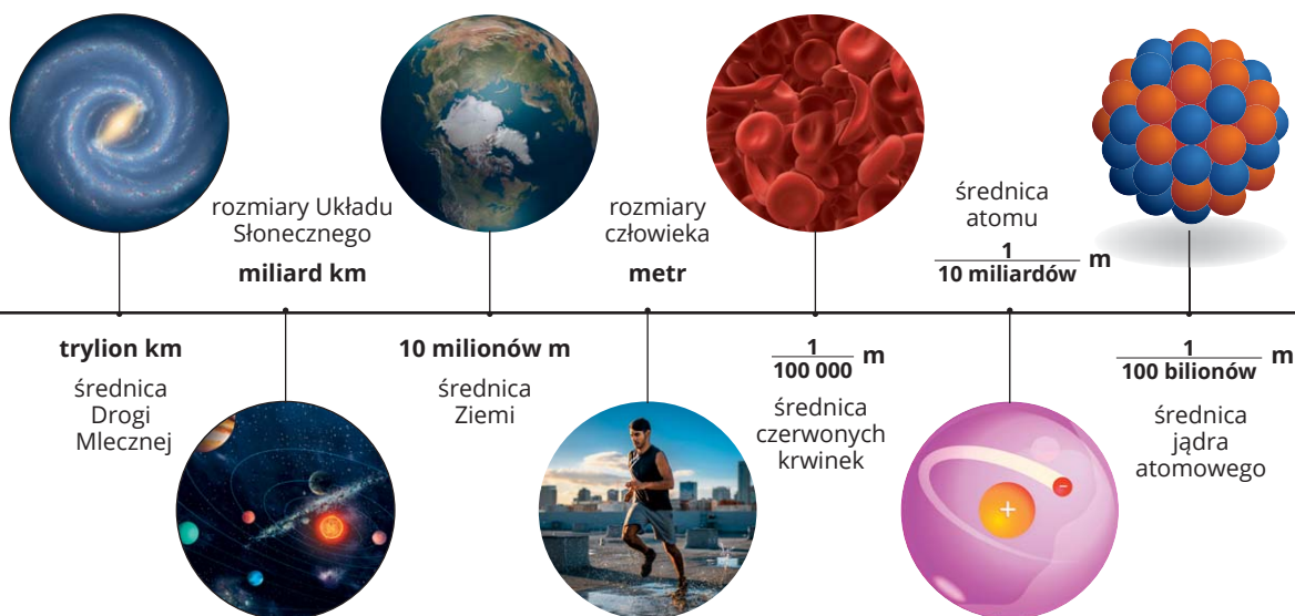
Rys. 2.1. Przykłady obiektów o różnych rozmiarach (podany rząd wielkości, a nie dokładne rozmiary)
