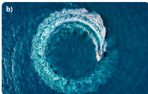
Rys. 14.4. Tor ruchu łodzi motorowej: prostoliniowy (a) i krzywoliniowy (b)
