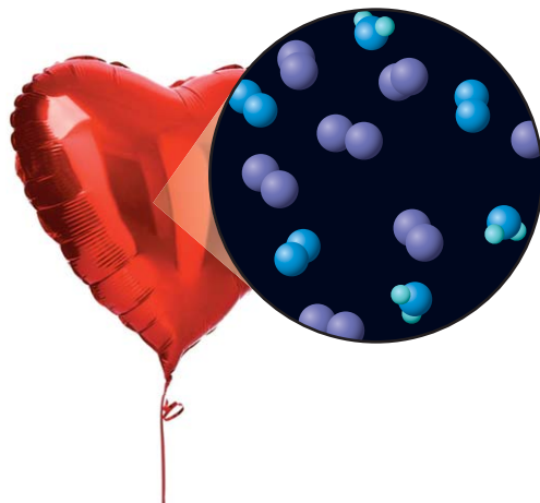
Rys. 2.3. Gaz wewnątrz balonika wypełnia całą dostępną objętość.
