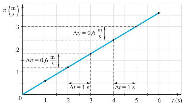
Rys. 24.2. W ruchu jednostajnie przyspieszonym w tych samych odstępach czasu prędkość rośnie o tyle samo.
