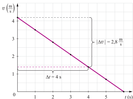
Rys. 24.4. Z wykresu zależności prędkości od czasu można obliczyć przyspieszenie.
