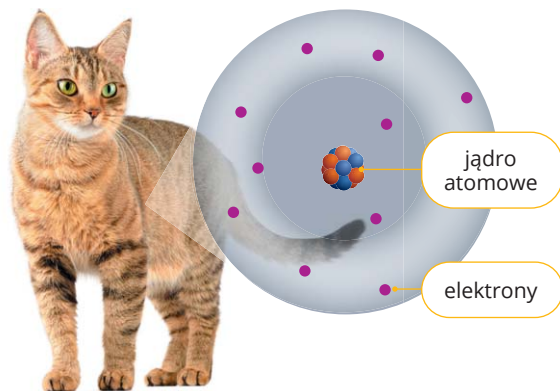
Rys. 2.2. Materia wokół nas składa się z atomów. Atom zbudowany jest z bardzo małego jądra oraz krążących wokół niego jeszcze mniejszych elektronów.
