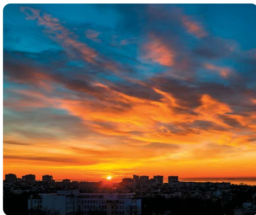
Rys. 1.2. Obserwacja wschodu słońca
