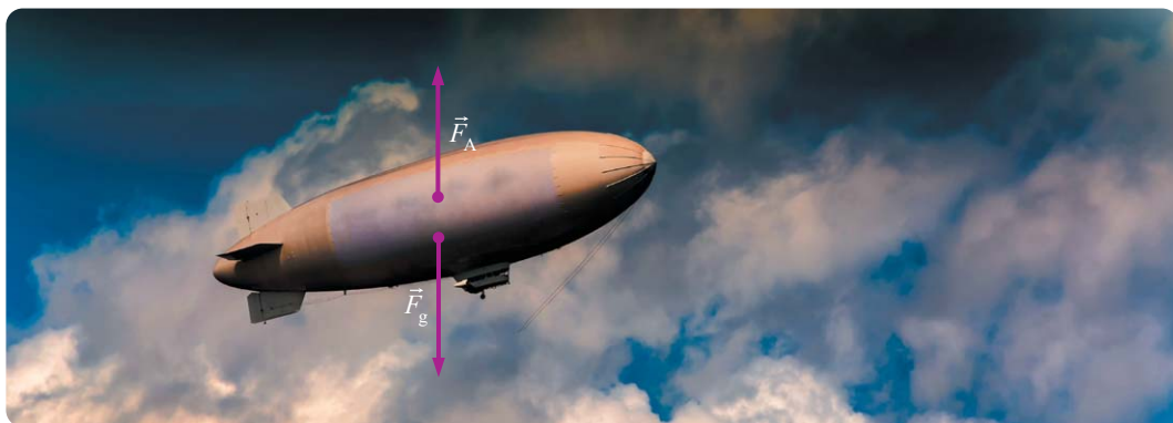
Rys. 13.3. Na sterowiec poruszający się w powietrzu także działa siła wyporu.
