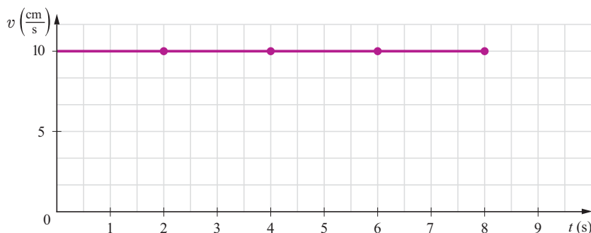
Rys. 19.5. Wykres zależności prędkości od czasu w ruchu jednostajnym
