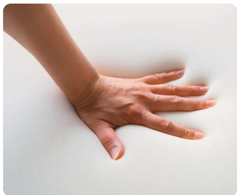
Rys. 3.2. Ręka i materac oddziałują ze sobą sprężystości.
