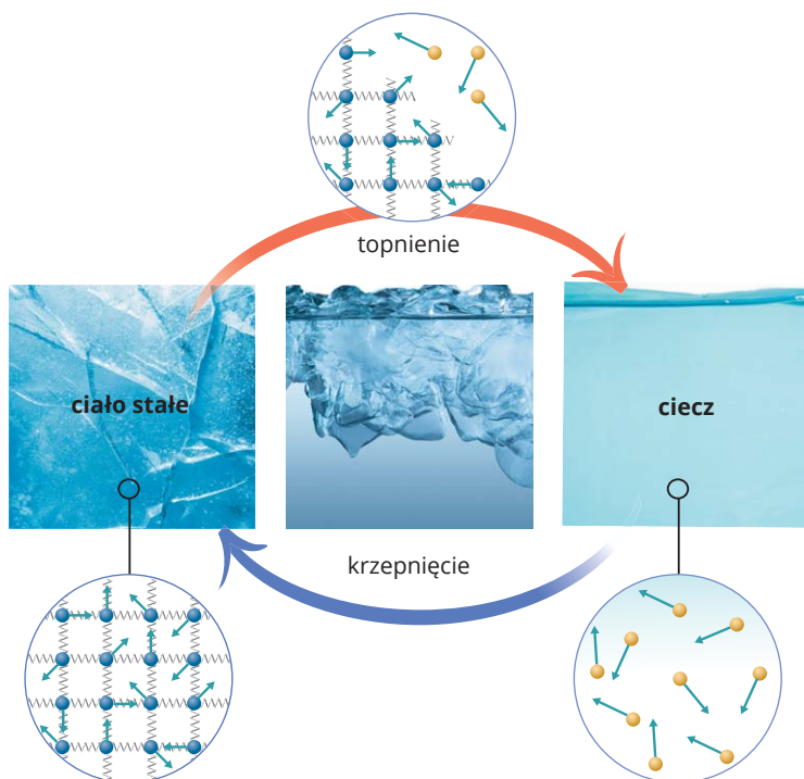
Rys. 33.3. Podczas topnienia i krzepnięcia zmienia się uporządkowanie cząsteczek substancji.
