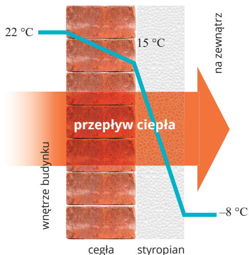
Rys. 35.1. Przepływ ciepła przez ścianę pokrytą izolatorem
