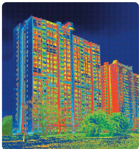
Rys. 35.2. Obraz z kamery termowizyjnej budynków z lepszą (budynek po lewej) i gorszą (budynek po prawej) izolacją ścian szczytowych
