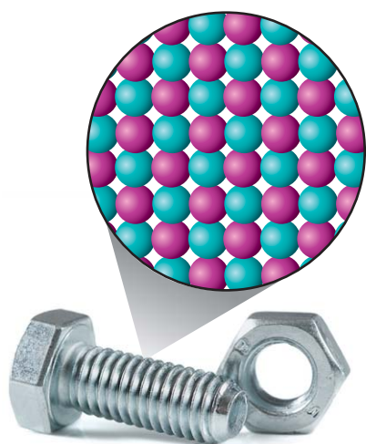
Rys. 2.5. W ciałach krystalicznych cząsteczki tworzą uporządkowaną strukturę.
