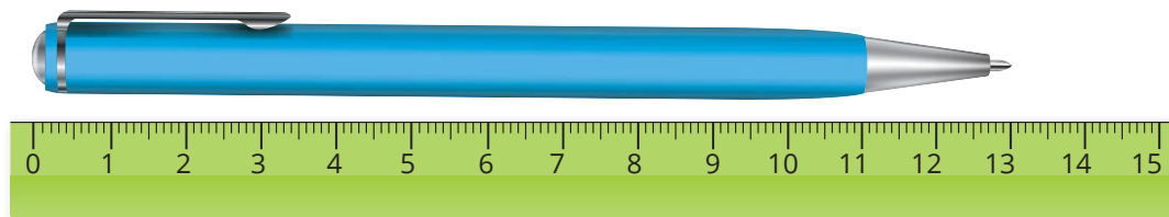
Rys. 1.3. Pomiar długości długopisu za pomocą linijki
