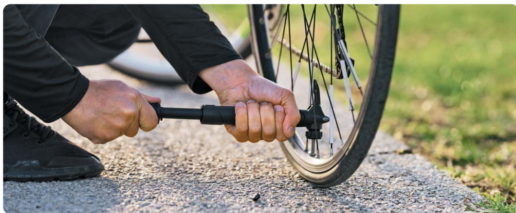
Rys. 32.3. Podczas pompowania dętki koła rowerowego zwiększa się energia wewnętrzna powietrza w pompce.
