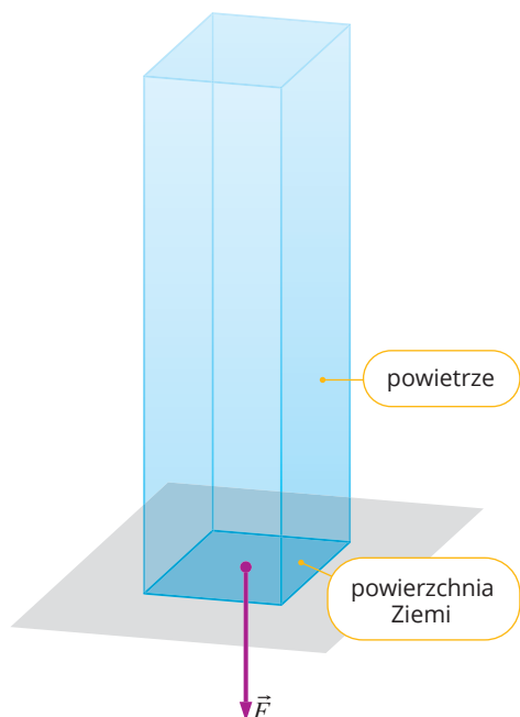
Rys. 10.1. Słup powietrza atmosferycznego działa siłą nacisku na powierzchnię Ziemi.
