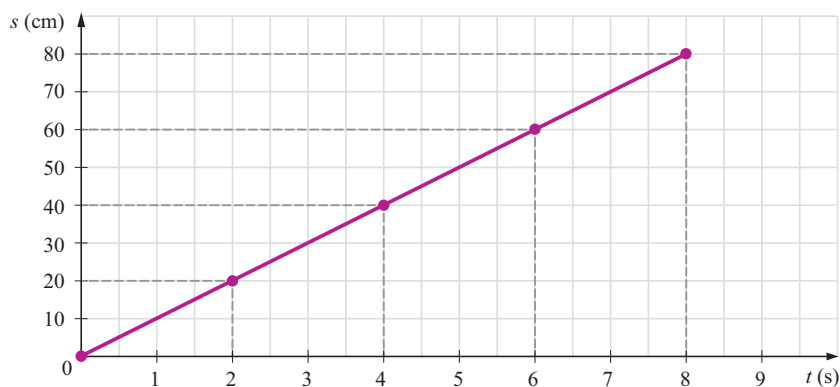
Rys. 19.4. Półprosta przechodząca przez punkty tworzy liniowy wykres zależności drogi od czasu.
