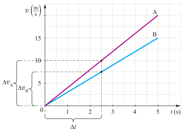
Rys. 24.3. Wykres zależności prędkości od czasu dla motocykli A i B poruszających się z różnymi przyspieszeniami
