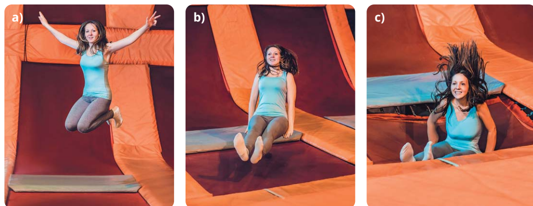
Rys. 27.1. Trzy rodzaje energii mechanicznej: energia potencjalna grawitacji – dziewczyna na pewnej wysokości nad trampoliną (a), energia kinetyczna – dziewczyna w ruchu (b), energia potencjalna sprężystości – odkształcona trampolina (c)
