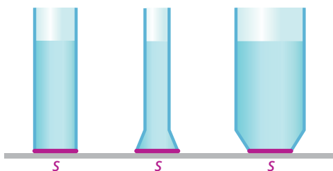
Rys. 2. Siła parcia na dno tych naczyń jest taka sama, jednakowe jest również ciśnienie przy dnie.
