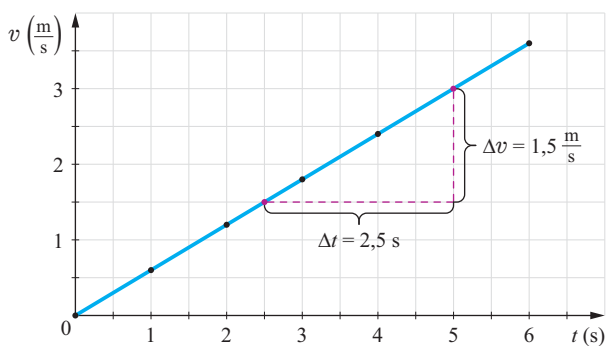
Rys. 24.1. Z wykresu zależności prędkości od czasu można obliczyć przyspieszenie.
