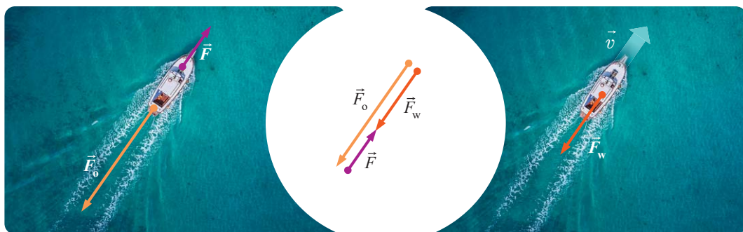
Rys. 23.3. Siła wypadkowa \vec{F}_w zwrócona przeciwnie do prędkości powoduje, że prędkość motorówki maleje.
