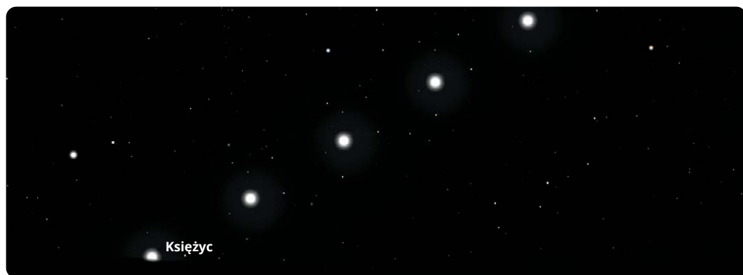
Rys. 14.3. Fotografie Księżyca wykonywane co godzinę i nałożone na siebie
