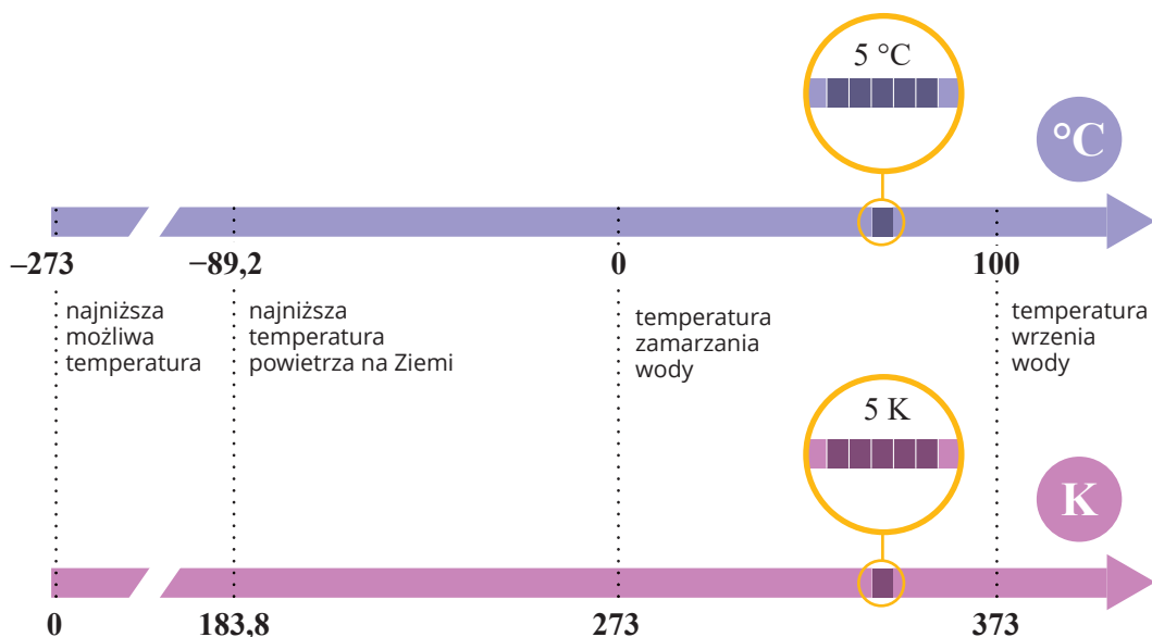
Rys. 31.1. Porównanie temperatur w skalach Celsjusza i Kelvina
