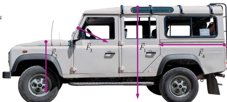
Rys. 10.2. Siły nacisku (parcia) atmosfery działające na różne powierzchnie nadwozia samochodu
