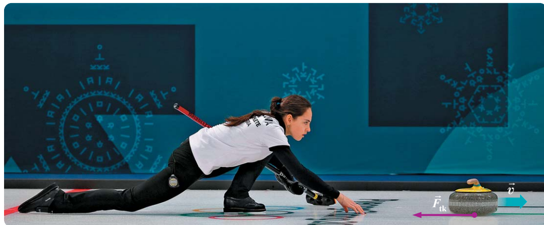
Rys. 22.3. Siła tarcia kinetycznego działająca na poruszający się kamień podczas gry w curling
