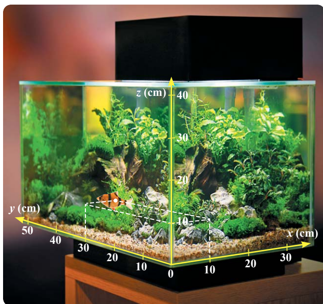
Rys. 15.5. Rybki mają możliwość poruszania się we wszystkich kierunkach. Współrzędne zaznaczonej na zdjęciu rybki to x = 10 cm, y = 30 cm i z = 10 cm.
