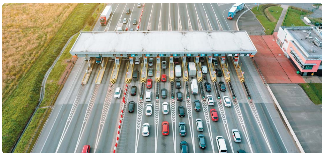
Rys. 16.1. Podczas podróży autostradą poruszamy się zarówno ruchem jednostajnym, jak i zmiennym.
