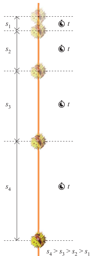
Rys. 16.3. Kasztan poruszający się ruchem zmiennym
