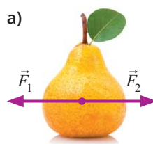
Rys. 6.2. Siły równoważące się (a) oraz siły działające na dwa różne ciała (b)
