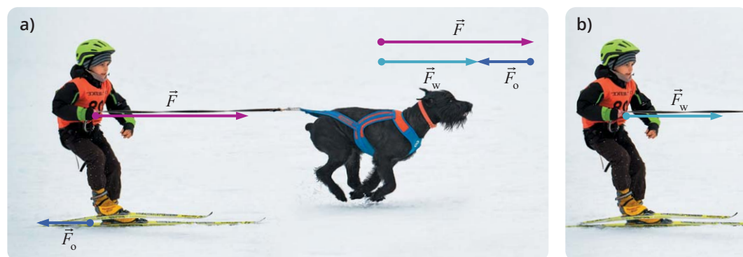
Rys. 23.2. Na narciarza działają dwie siły (a), a ich wypadkowa powoduje wzrost jego prędkości (b).
