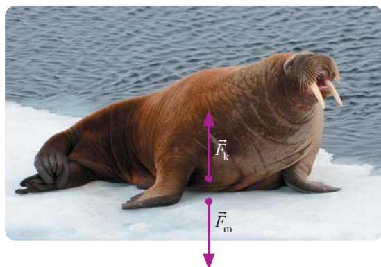
Rys. 4.5. Siła nacisku ciała morsa \vec{F}_m przyłożona jest do powierzchni kry, a siła nacisku kry \vec{F}_k przyłożona jest do powierzchni ciała morsa.
