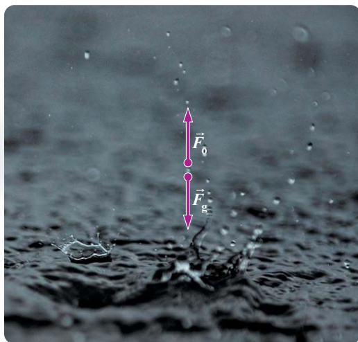
Rys. 18.2. Ruch jednostajny kropli deszczu
