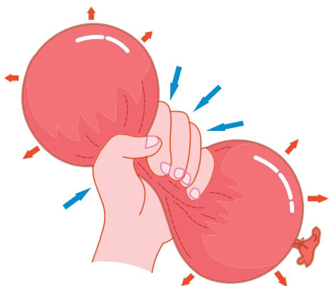
Rys. 12.3. Dodatkowe ciśnienie wywierane na balon rozchodzi się równomiernie w całej jego objętości.
