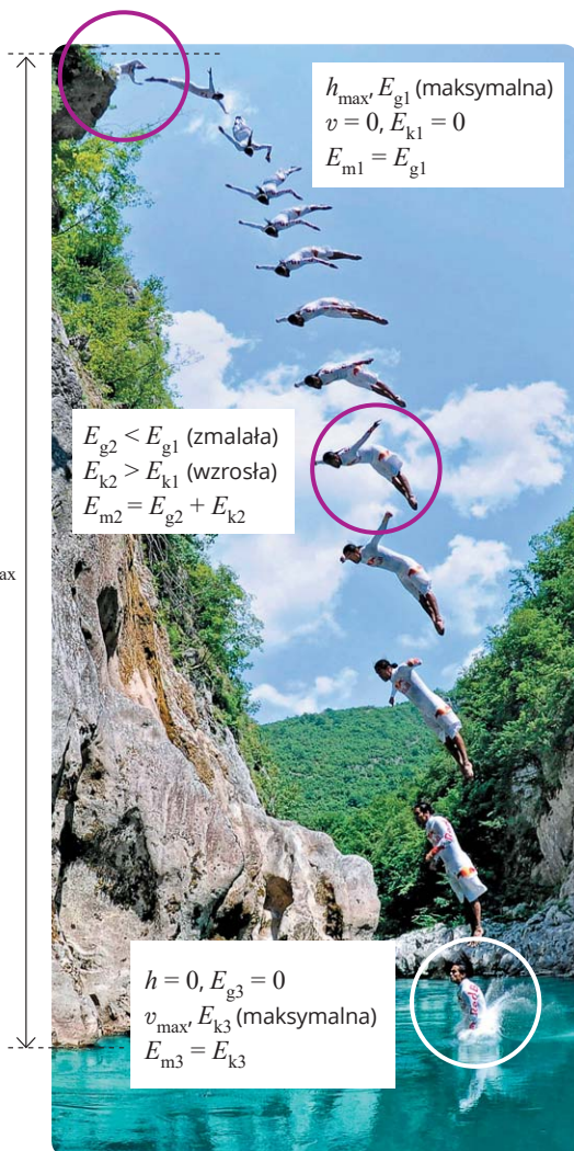
Rys. 29.3. Podczas spadania energia grawitacji zamienia się w energię kinetyczną.
