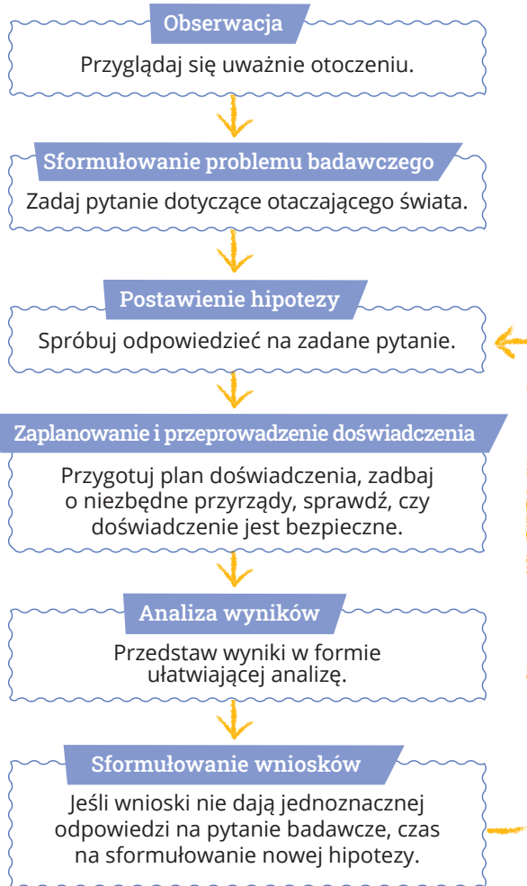
Rys. 1.1. Etapy metody naukowej
