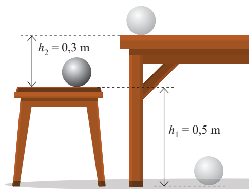
Rys. 27.3. Energia grawitacji ciała zależy od wysokości mierzonej względem wybranego poziomu odniesienia.
