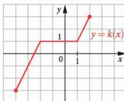
Funkcja k jest ciągła w \langle -4; 2 \rangle .
