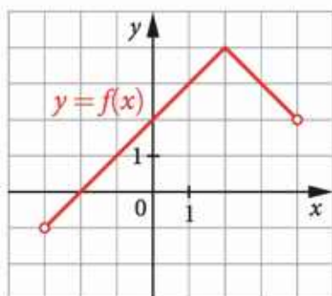
Funkcja f jest ciągła w (-3; 4) .
