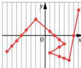
To nie jest wykres funkcji.
