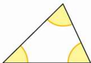
trójkąt ostrokątny wszystkie kąty ostre
