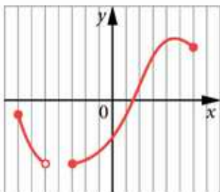
To jest wykres funkcji.
