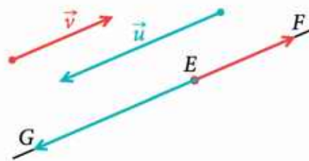
wektory o przeciwnych zwrotach
