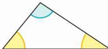
trójkąt rozwartokątny jeden kąt rozwarty
