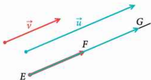
wektory o zgodnych zwrotach
