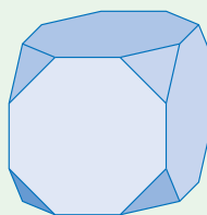
sześcián ścięty
