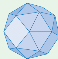
sześcián przycięty
