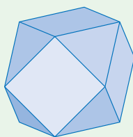
sześćcio-ośmiościan
