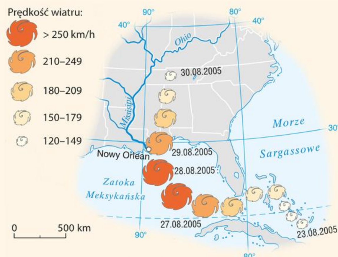
Kierunek przemieszczania się huraganu Katrina.
