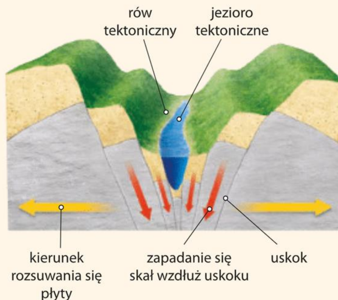
Powstawanie rowów tektonicznych.
