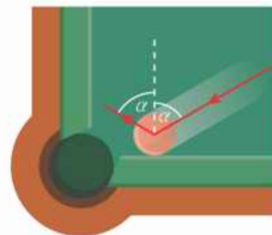
▲ Prawo odbicia dla kul bilardowych
