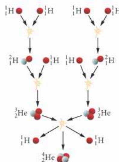
▲ Uproszczony schemat syntezy wodoru w hel
