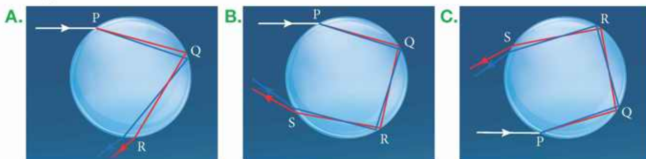
▲ Powstawanie drugiej (zewewnętrznej) tęczy
