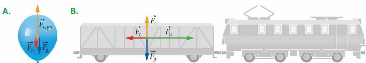
▲ Siły działające na: A. balonik z helem, B. wagon kolejowy
