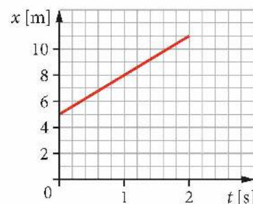
▲ Wykres zależności x(t) dla x_0 = 5 \text{ m} , v = 3 \frac{\text{m}}{\text{s}}
