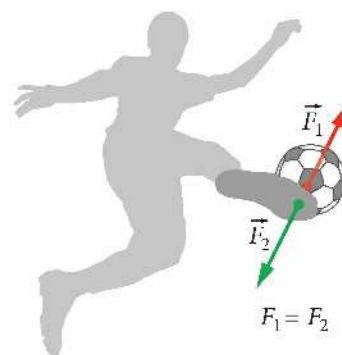
▲ Oddziaływanie stopy i piłki jest wzajemne, obie siły mają równe wartości
