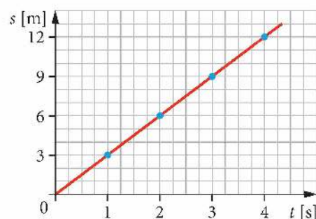
▲ Wykresy zależności: v(t) , s(t) dla v = 3 \frac{\text{m}}{\text{s}}
