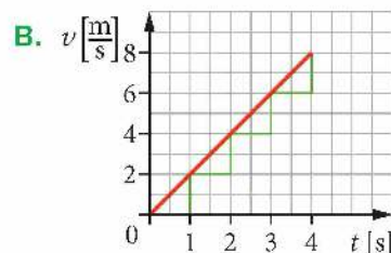
▲ Wykres zależności prędkości od czasu v(t)
