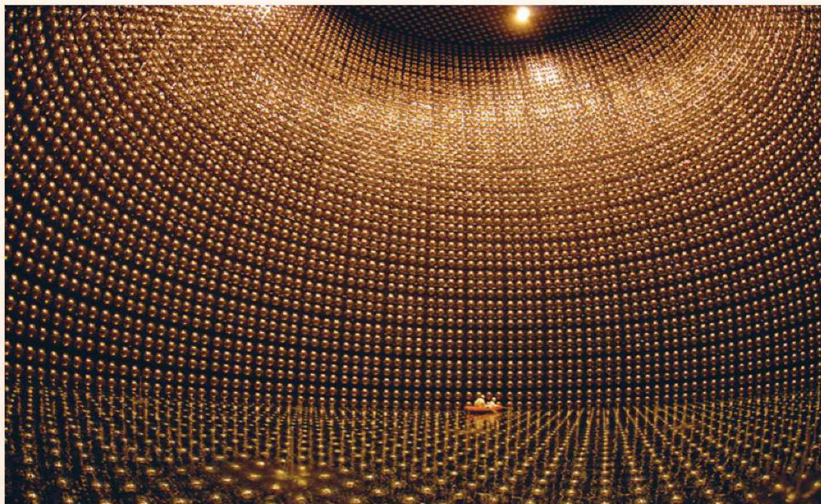
▲ Detektor neutrin Super-Kamiokande zawiera aż 50 000 ton wody. Naokoło niej znajdują się czujniki światła powstającego w następstwie oddziaływania neutrin w wodzie. Na zdjęciu widzisz także pracowników obsługi w pontonie, sprawdzających czujniki w trakcie napełniania detektora wodą
