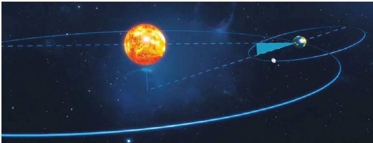
▲ Nachylenie orbity Księżyca względem orbity Ziemi
