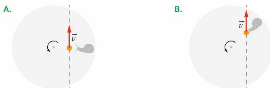
▲ Piłeczka na tarczy z punktu widzenia układu inercyjnego
