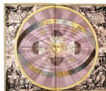
▲ Model heliocentryczny Mikołaja Kopernika
