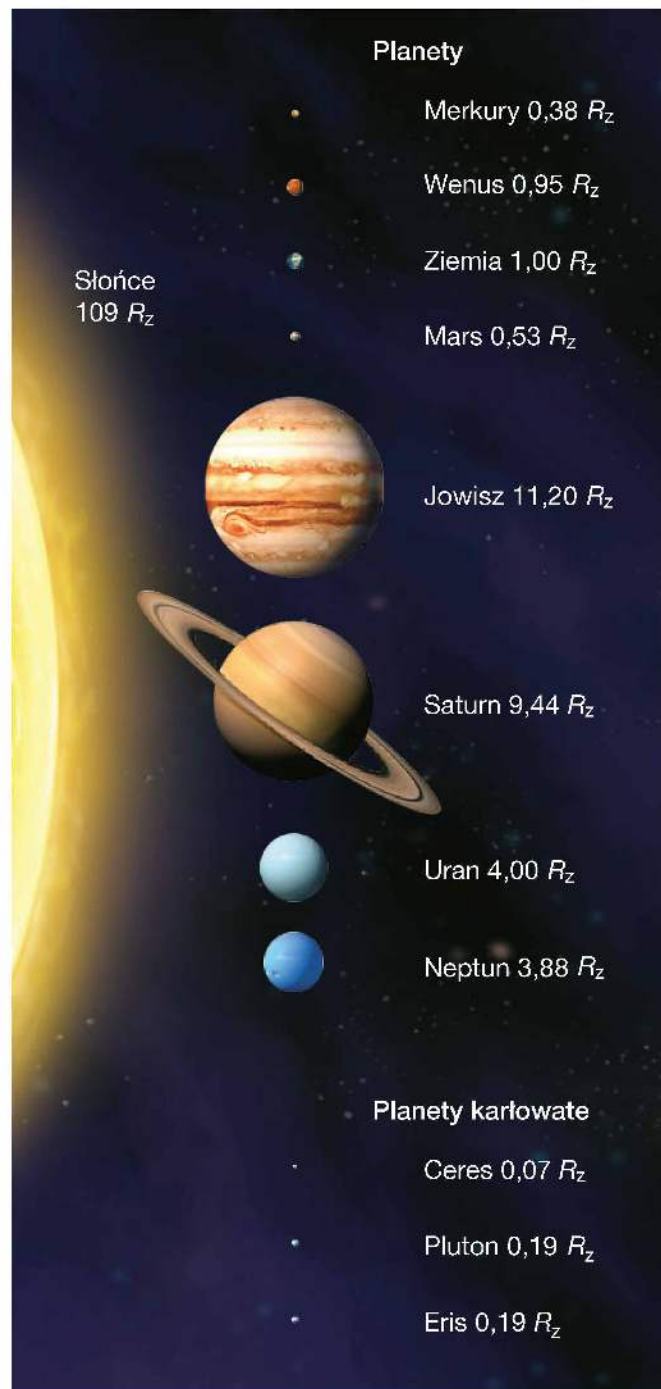
▲ Porównanie promieni: Słońca, planet Układu Słonecznego oraz trzech jego planet karłowatych ( R_Z – promień Ziemi)
