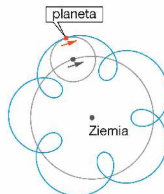
▲ Skomplikowany tor planety poruszającej się wokół Ziemi
