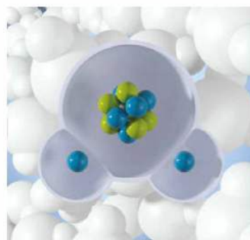
▲ Cząsteczka wody
