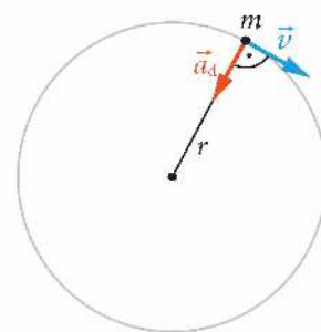
▲ Wektory prędkości i przyspieszenia w ruchu jednostajnym po okręgu
