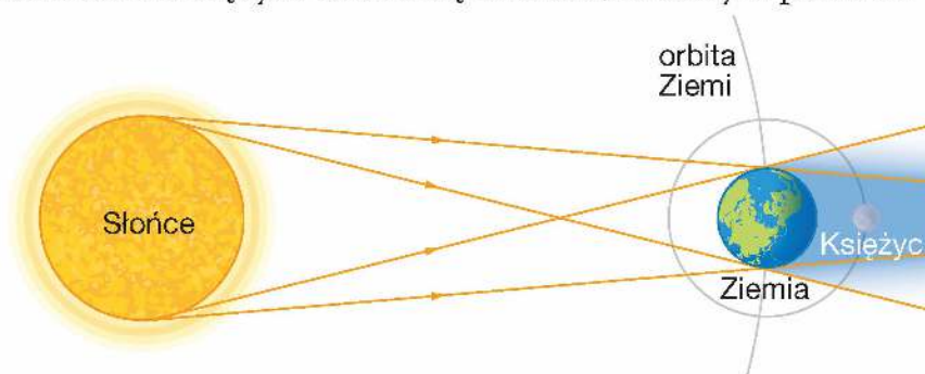
▲ Ustawienie Słońca, Ziemi i Księżyca podczas zaćmienia Księżyca
