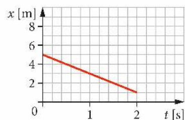
▲ Wykres zależności x(t) dla ciała poruszającego się w przeciwną stronę niż wskazuje strzałka osi
