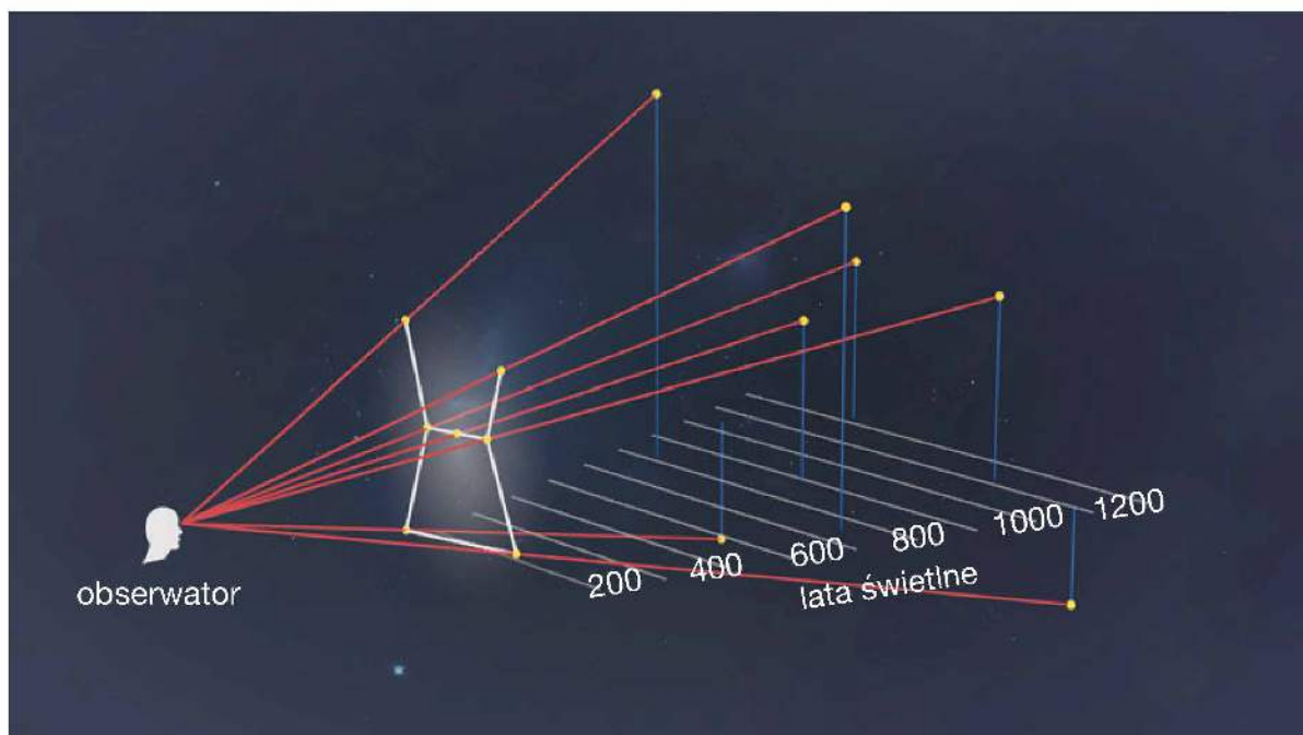
▲ Gwiazdy, które widzimy na niebie jako bliskie, mogą znajdować się w kosmosie daleko od siebie
