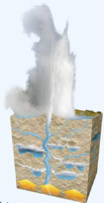
2 Gejzer.
