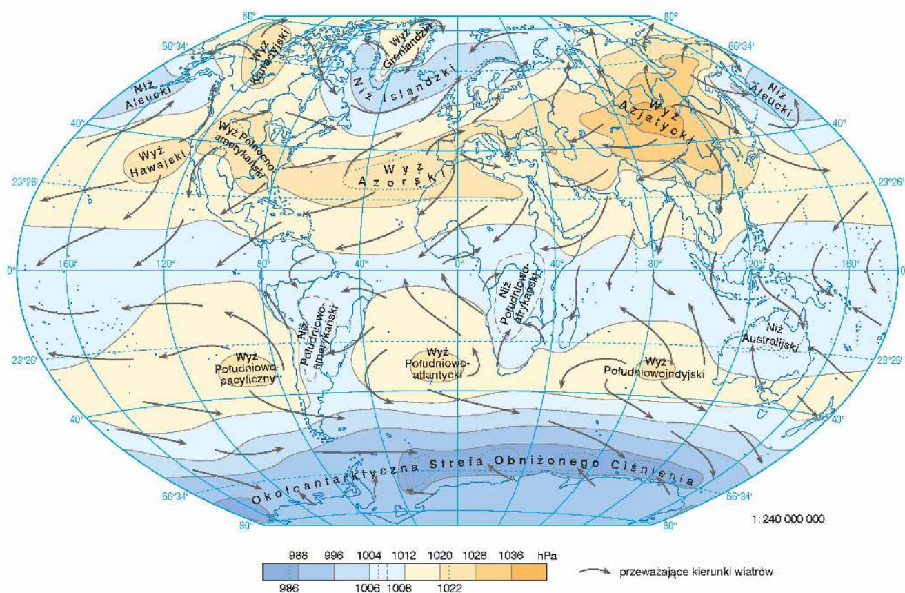
Rozkład ciśnienia barycznego w styczniu wraz z przeważającymi wiatrami
