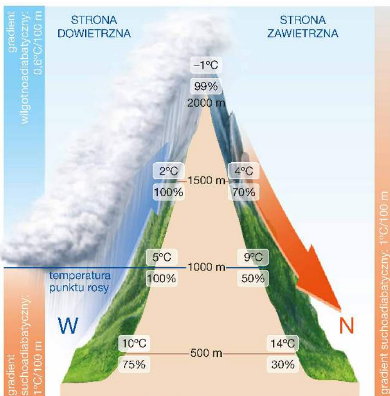
Powstawanie fenu.
