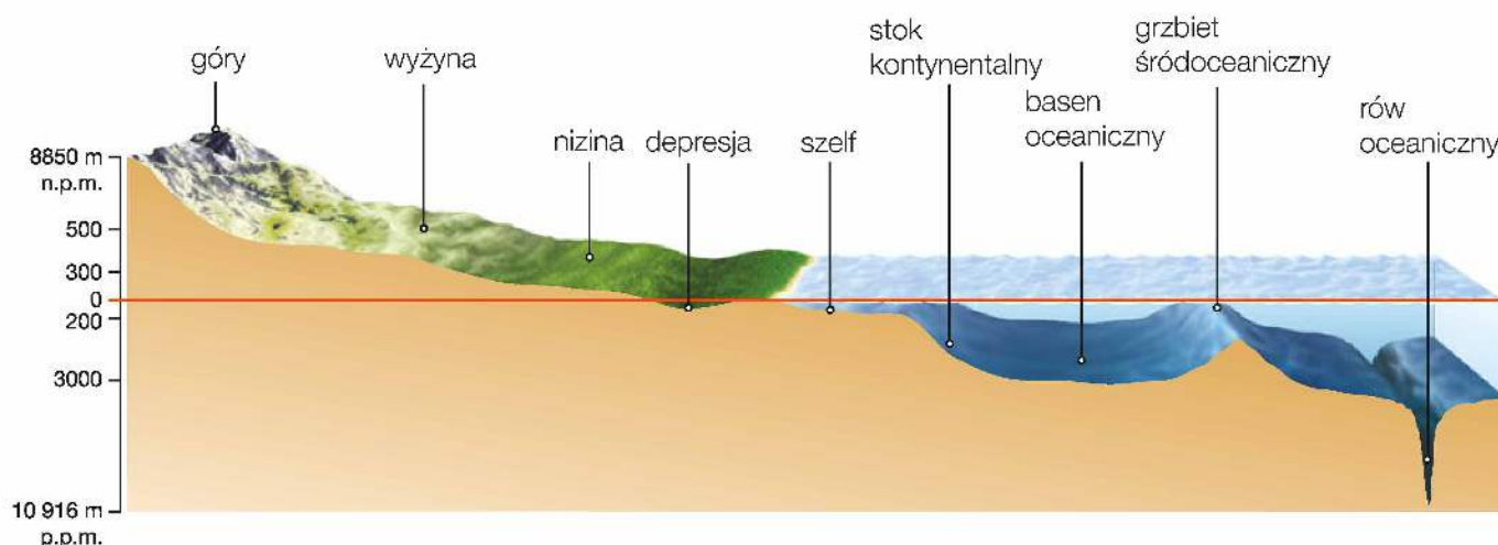
Wielkie formy ukształtowania lądów i dna oceanicznego.
