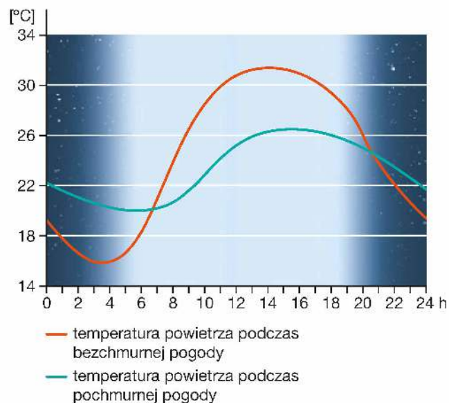
Dobowy przebieg temperatury powietrza.
