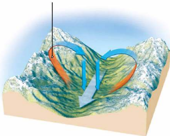
Wiatr dolinny.
