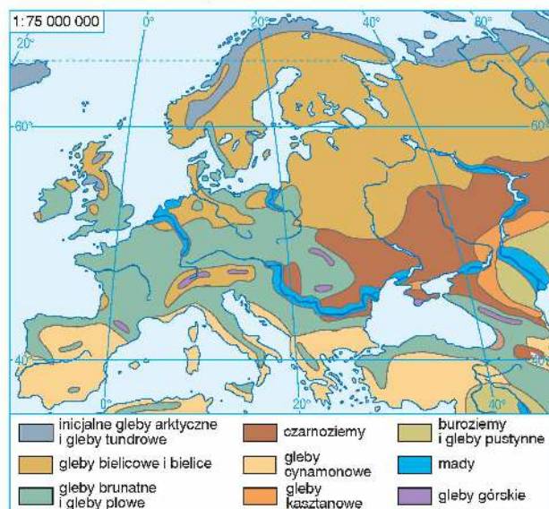
Rozmieszczenie gleb w Europie
