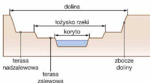
Elementy doliny rzecznej.
