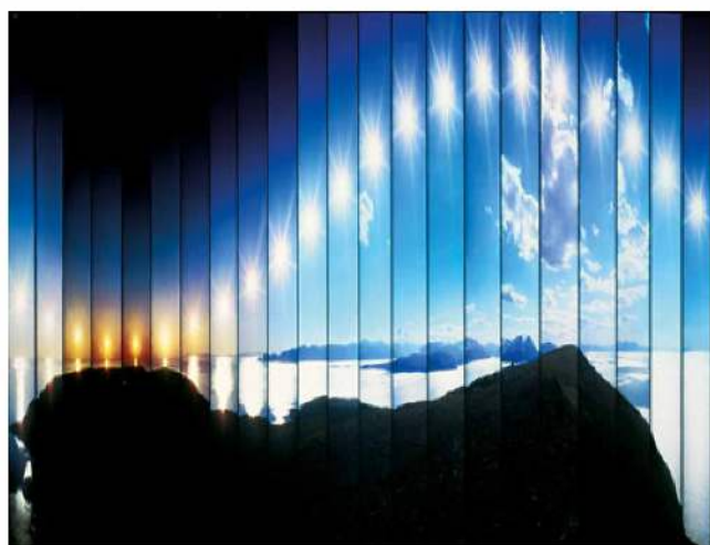
Fotografie przedstawiające położenie Słońca wykonano w godzinnych odstępach w dniach 21 i 22 lipca na norweskiej wyspie Loppa.
