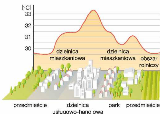
Miejska wyspa ciepła.
