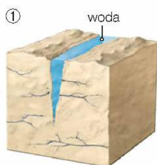
Woda wnika w istniejące szczeliny skalne.
