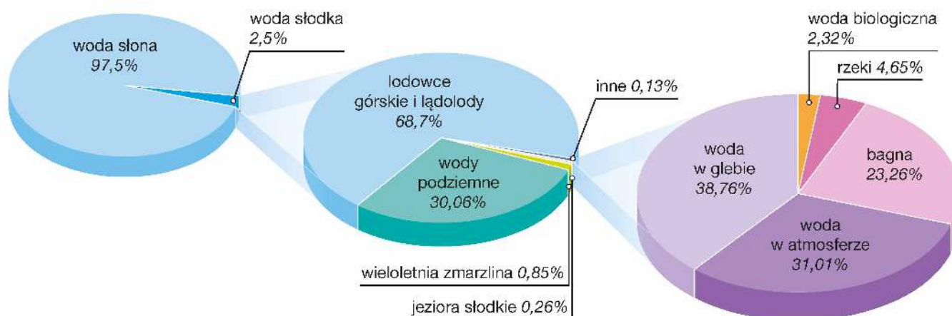
Zasoby wodne Ziemi (procent objętości).
