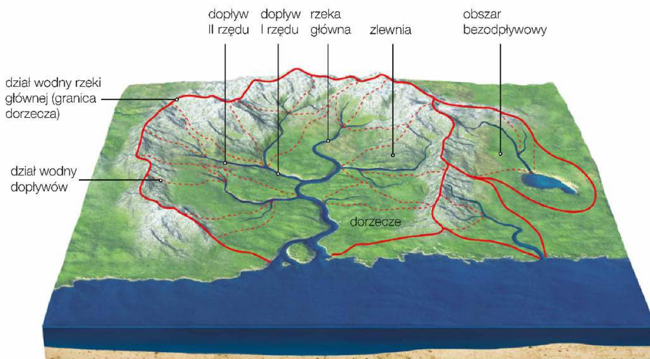
System rzeczny wraz z dorzeczem.
