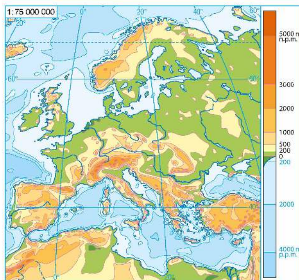
Mapa hipsometryczna Europy
