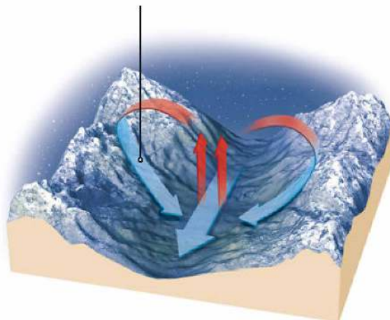
Wiatr górski.
