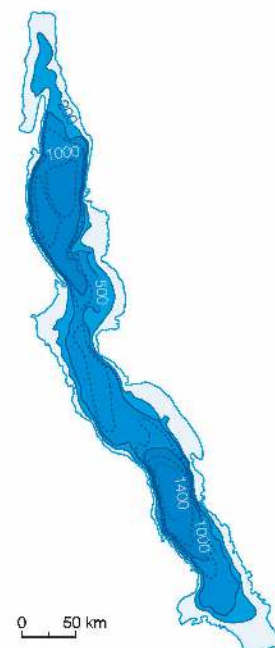
Tanganika
