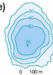
Czarny Staw pod Rysami
