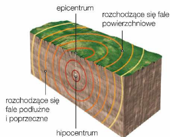
Rozchodzenie się fal sejsmicznych.
