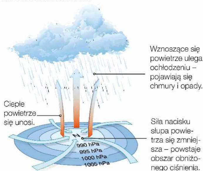
Niż baryczny.
