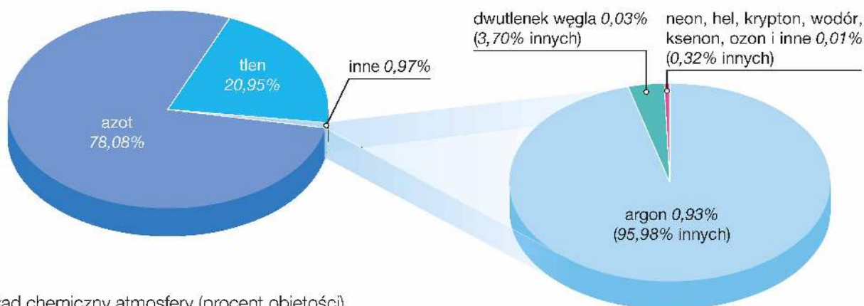
Skład chemiczny atmosfery (procent objętości).
