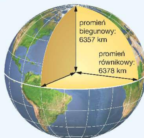
1 Spłaszczenie biegunowe.
