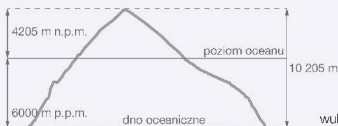
Profil wulkanu Mauna Kea pokazany od dna oceanicznego do najwyższego wierzchołka.
