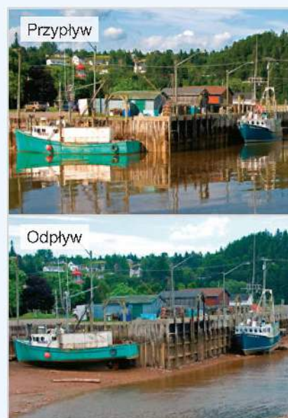
2 Pływy.
