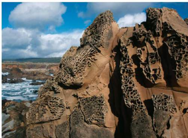
Na skutek wietrzenia chemicznego mogą powstawać w skałach zagłębienia przypominające plastry miodu – tafoni. Występują one na przykład na wybrzeżu Kalifornii.
