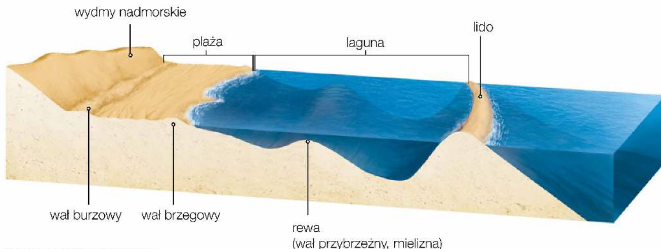
Budowa wybrzeża niskiego.
