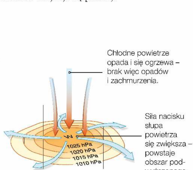
Wyż baryczny.
