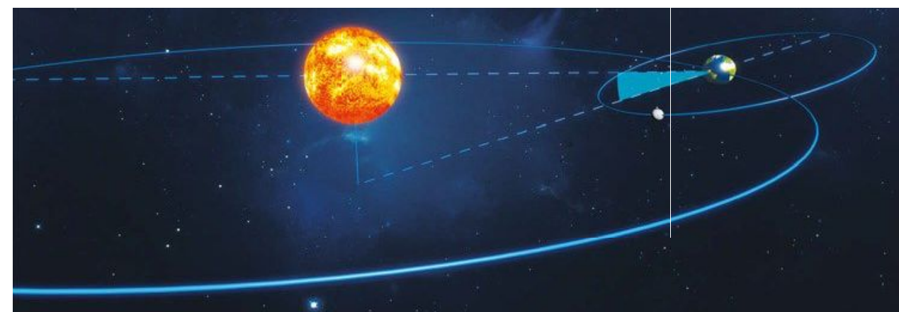
▲ Nachylenie orbity Księżyca względem orbity Ziemi
