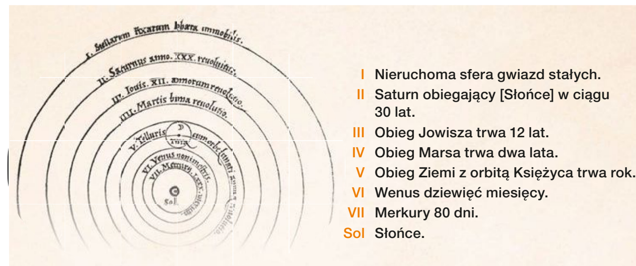
▲ Rycina z dzieła Mikołaja Kopernika O obrotach . Przy orbitach kolejnych planet podano ich okres obiegu (tłumaczenie znajduje się obok ilustracji)
