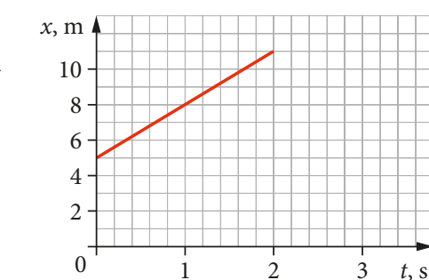
▲ Wykres zależności x(t) dla x_0 = 5 \text{ m} , v = 3 \frac{\text{m}}{\text{s}}
