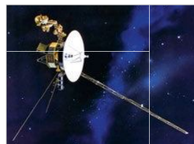
▲ Wystrzelona w 1977 r. sonda Voyager 1 oddaliła się od Ziemi o zaledwie 24 mld km, czyli niecałą dobę świetlną, a już teraz przyciąganie przez Słońce powoduje zmniejszenie jej prędkości zaledwie o 0,04% rocznie. W kosmosie można znaleźć obszary odległe o miliony lat świetlnych od najbliższej gwiazdy
