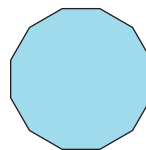
dwunastokąt foremny
