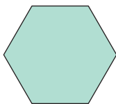
sześciokąt foremny
