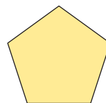
pięciokąt foremny
