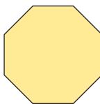
ośmiokąt foremny
