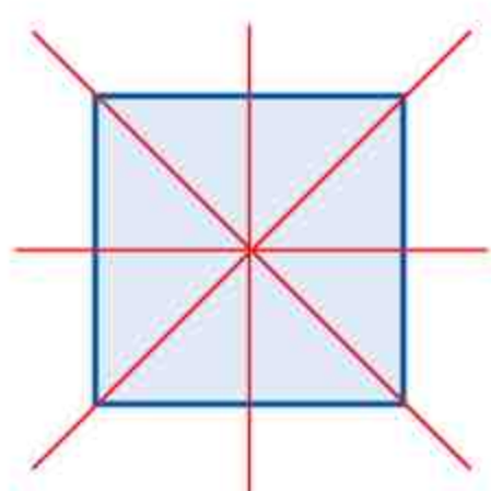
Kwadrat ma 4 osie symetrii.
