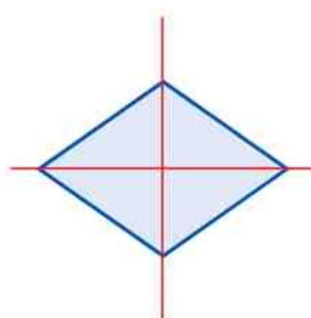
Romb ma 2 osie symetrii.
