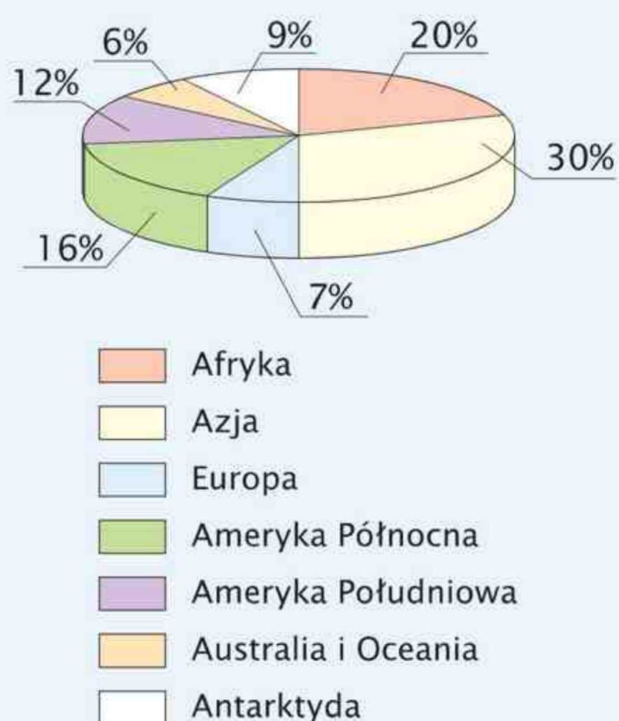
Powierzchnia lądów na Ziemi
