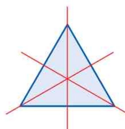
Trójkąt równoboczny ma 3 osie symetrii.
