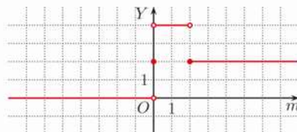
Wykres funkcji y = g(m)
