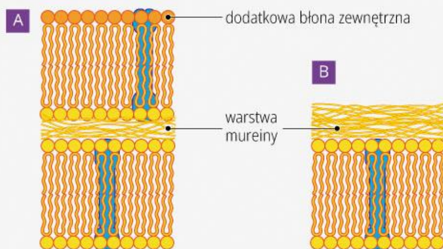
Schemat ściany komórkowej: A. Bakteria Gram-ujemna, B. Bakteria Gram-dodatnia
