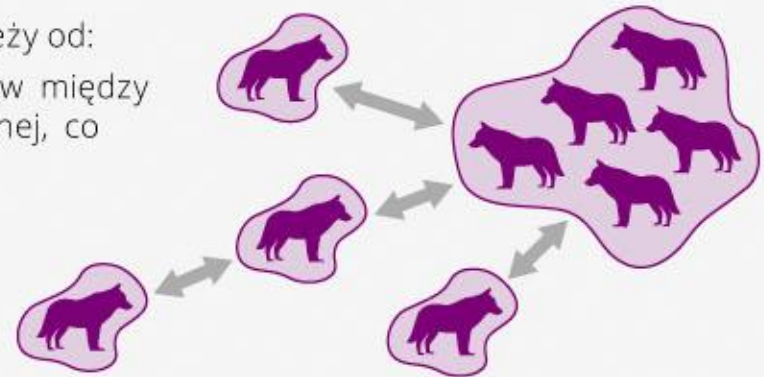
Dynamika liczebności hipotetycznej metapopulacji
