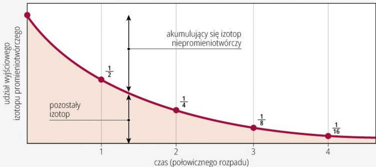
Datowanie izotopowe i czas połowicznego rozpadu
