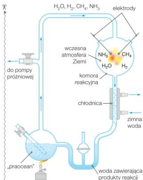
Aparat skonstruowany przez Millera i Ureya.
