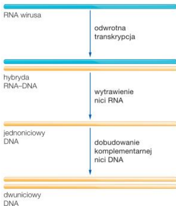
Etapy odwrotnej transkrypcji.
