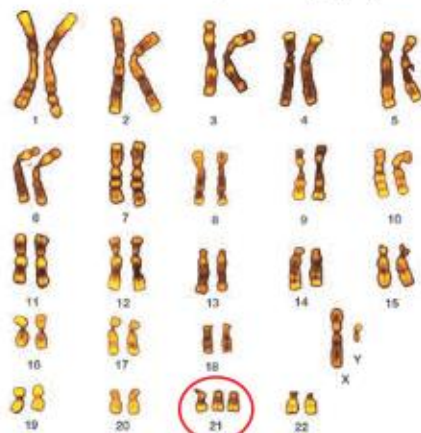
Kariogram osoby z zespołem Downa. Kariotyp zawiera trzy chromosomy 21.
