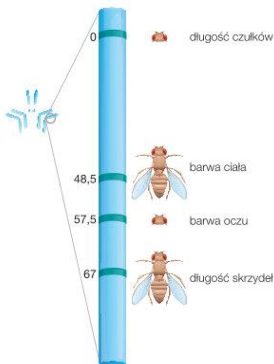
Sposób rozmieszczenia alleli wybranych genów na chromosomie drugim muszki owocowej. Jednostki mapowe (liczby naniesione na rysunku) obliczono z dokładnością do jednego miejsca po przecinku.
