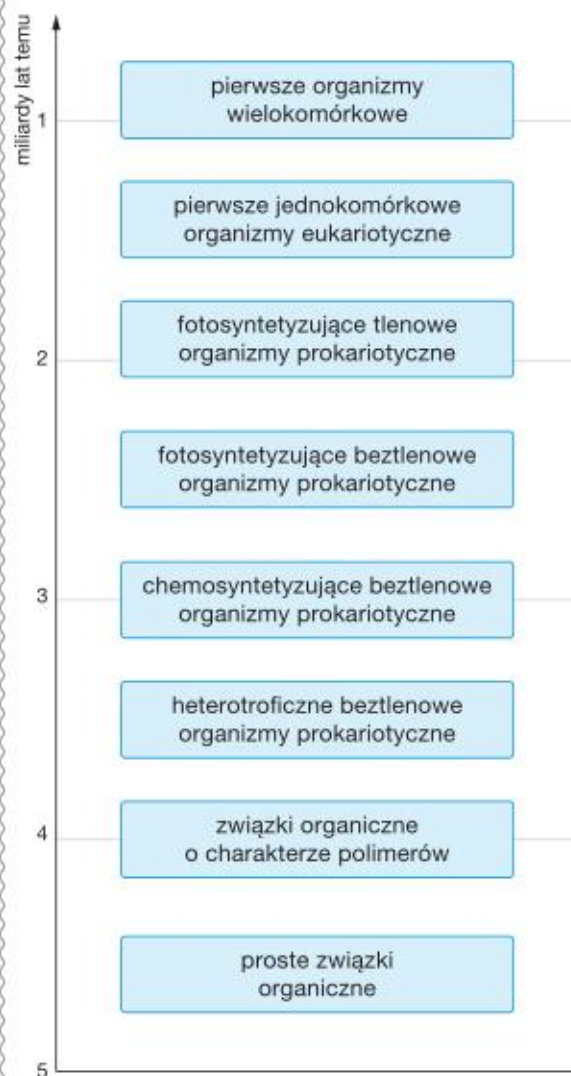
Etapy rozwoju życia na Ziemi.
