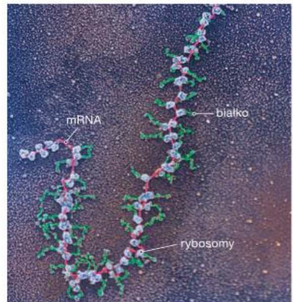
Translacja w komórce eukariotycznej (obraz spod TEM).
