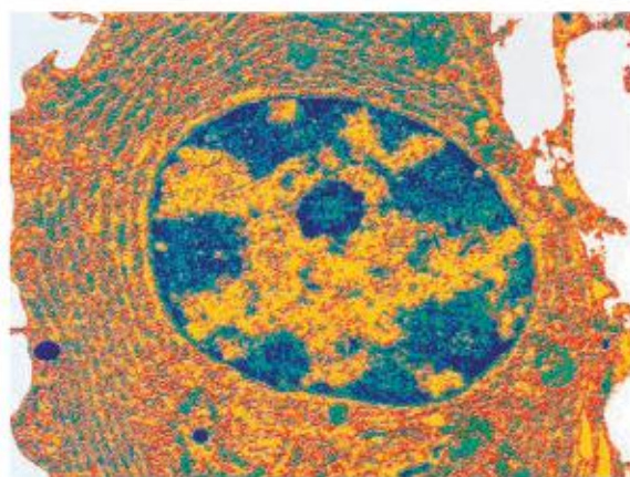
Struktura chromatyń w jądrze komórkowym (obraz spod TEM). Heterochromatyna znajduje się zwykle pod otoczką jądrową i wokół jąderka (kolor niebieski), natomiast euchromatyna jest swobodnie rozproszona w pozostałej przestrzeni jądra komórkowego (kolor żółty).
