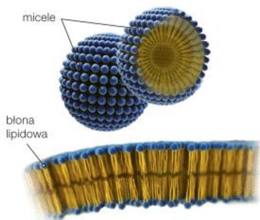
Budowa miceli i błon lipidowych.
