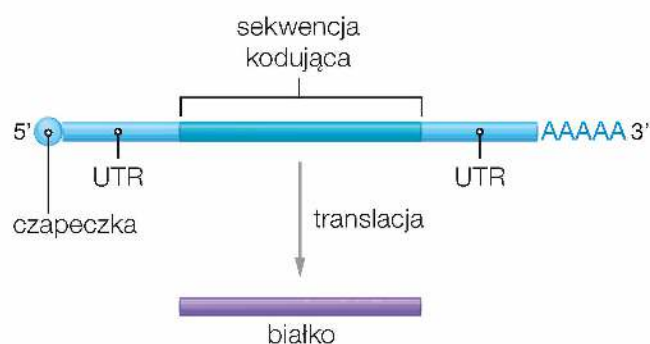
Budowa mRNA u organizmów eukariotycznych.
