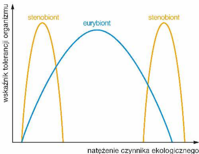
Porównanie zakresu tolerancji ekologicznej eurybiontów i stenobiontów.
