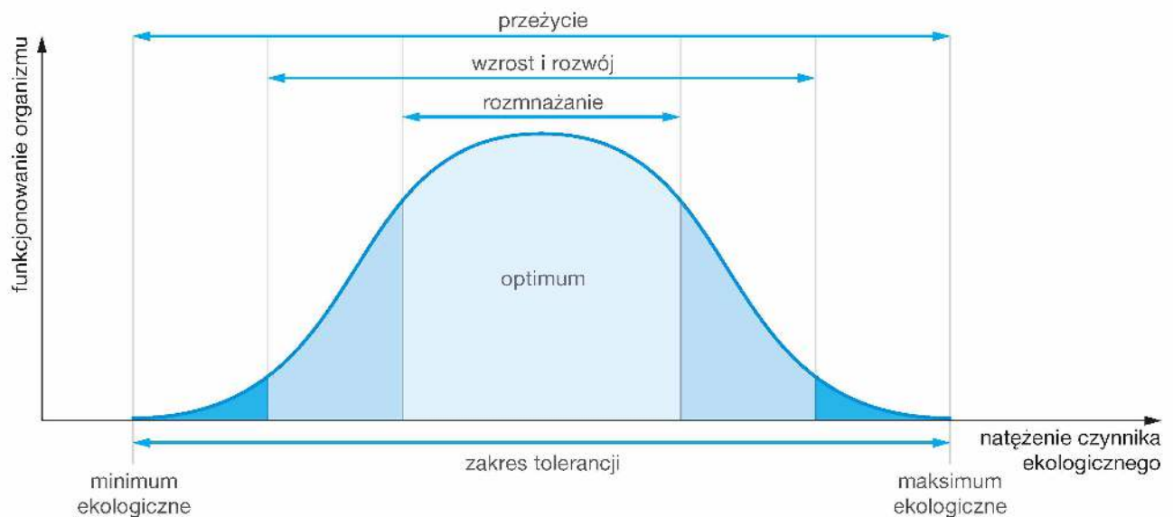
Zakres tolerancji organizmu na natężenie czynnika ekologicznego.
