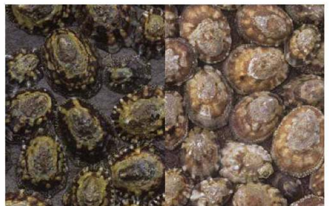
Ciemno i jasno ubarwione osobniki Acmea digitalis wykazują największą przeżywalność.
