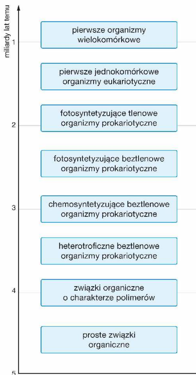
Etapy rozwoju życia na Ziemi.
