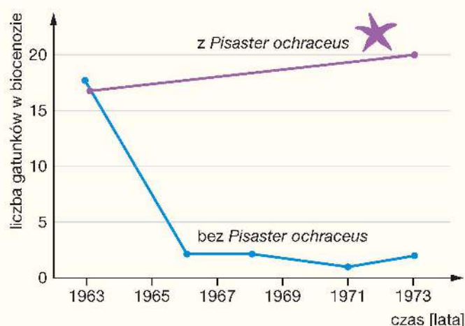
Wpływ rozgwiezdy Pisaster ochraceus na bogactwo gatunkowe badanej biocenozy.
