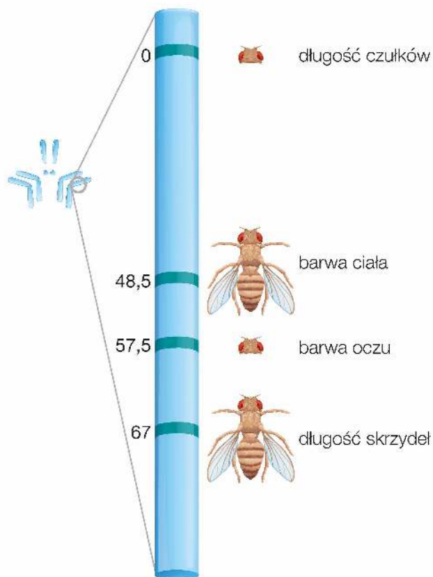
Sposób rozmieszczenia alleli wybranych genów na chromosomie drugiej muszki owocowej. Jednostki mapowe (liczby naniesione na rysunku) obliczono z dokładnością do jednego miejsca po przecinku.
