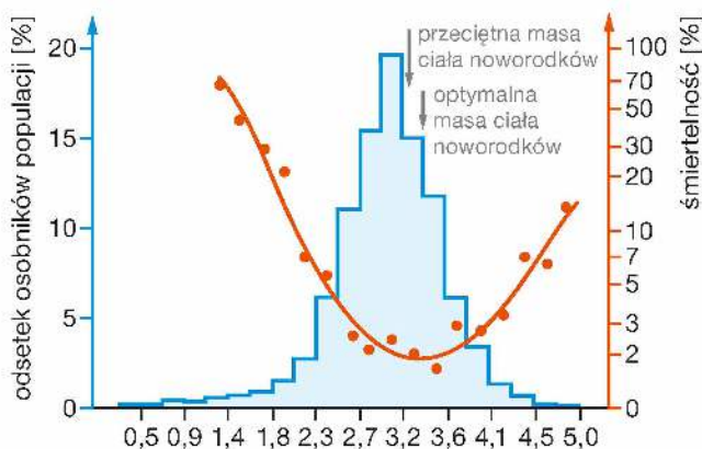
Rozkład masy ciała noworodków w populacji.
