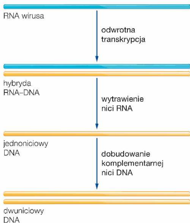
Etapy odwrotnej transkrypcji.
