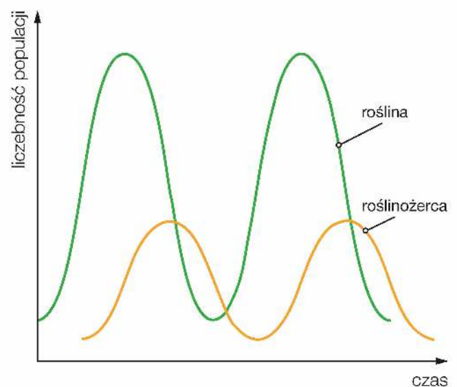
Wykres regulacji liczebności w układzie roślinożerca-roślina.
