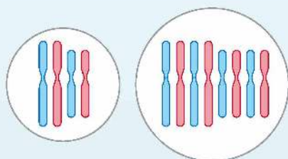
Komórka diploidalna ( 2n ).
