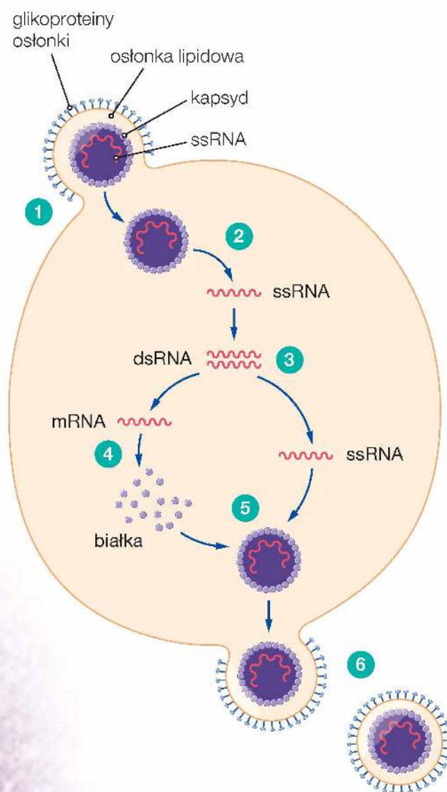
Uproszczony cykl infekcyjny koronawirusa.
