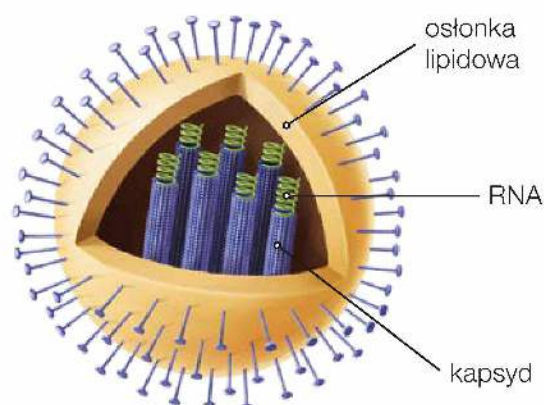
Struktura wirusa grypy.
