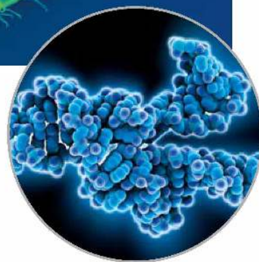
Model budowy rybozimu.
