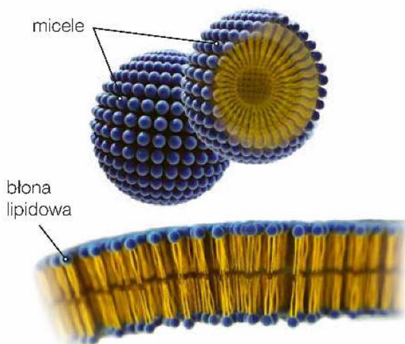
Budowa miceli i błon lipidowych.
