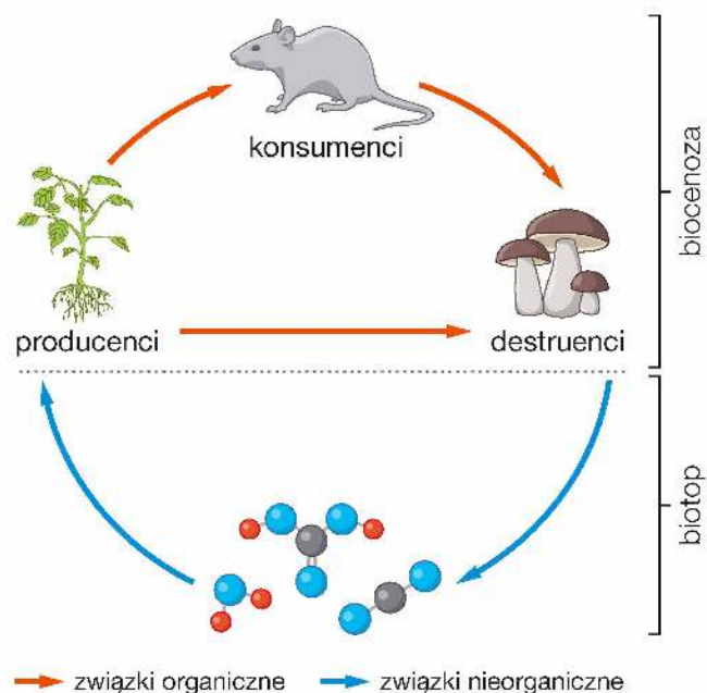
Schemat obiegu materii w ekosystemie.
