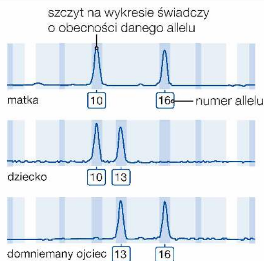
Przykładowy wynik badania ojcostwa.
