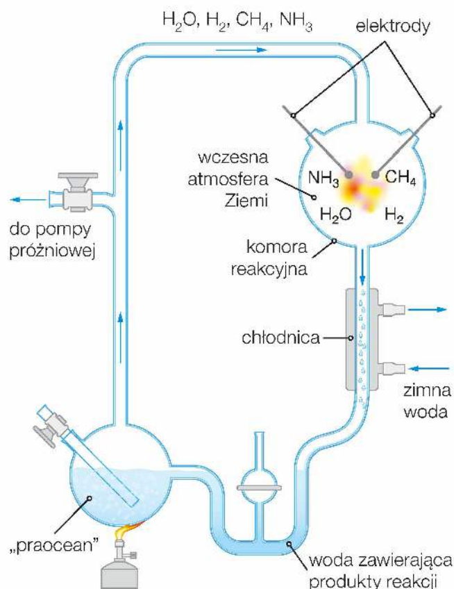
Aparat skonstruowany przez Millera i Ureya.
