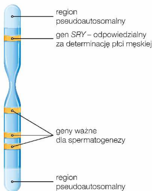
Lokalizacja niektórych genów na chromosomie Y.
