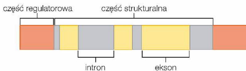
Budowa genu nieciągłego.
