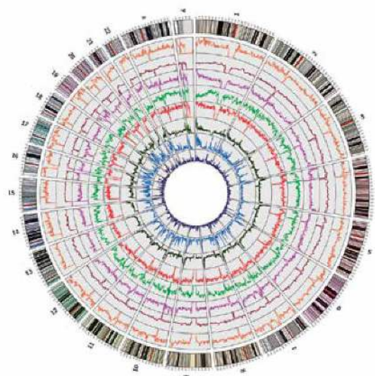
Mapa genetyczna człowieka.
