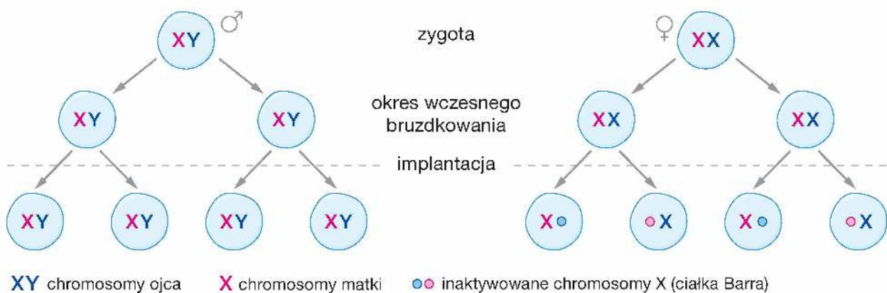
Schemat losowej inaktywacji chromosomu X.
