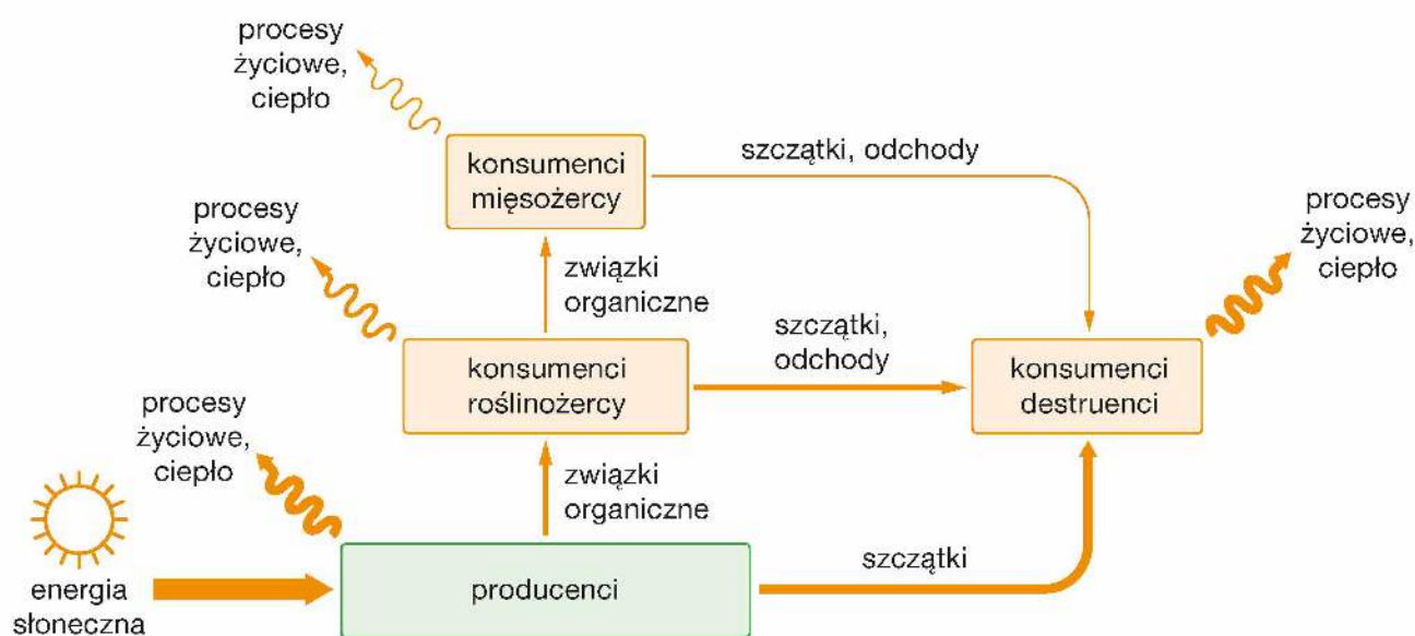
Schemat przepływu energii przez ekosystem.
