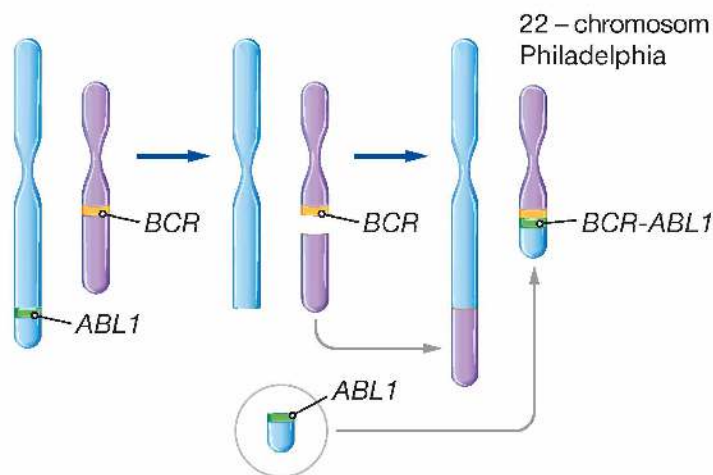
Powstawanie chromosomu Philadelphia.
