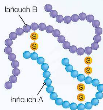
Cząsteczka ludzkiej insuliny.
