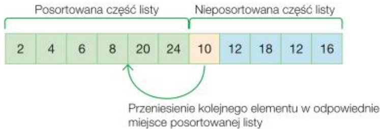
Rys. 8.10. Umieszczenie liczby 10 na częściowo uporządkowanej liście
