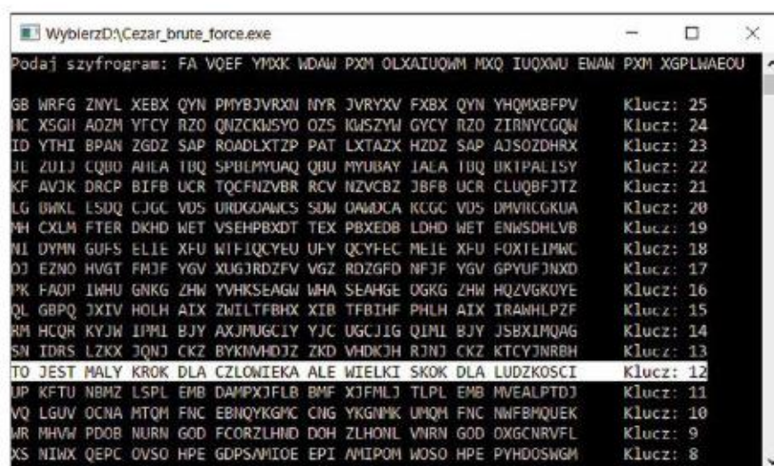
Rys. 2.10. Zastosowanie ataku siłowego do łamania szyfru Cezara
