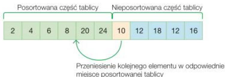
Rys. 3.10. Umieszczenie liczby 10 w częściowo uporządkowanej tablicy
