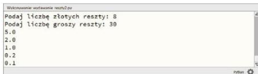
Rys. 9.5. Wywołanie programu Wydawanie reszty 2 dla kwoty 8 zł 30 gr
