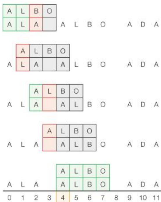
Rys. 1.7. Naiwne wyszukiwanie wzorca w tekście
