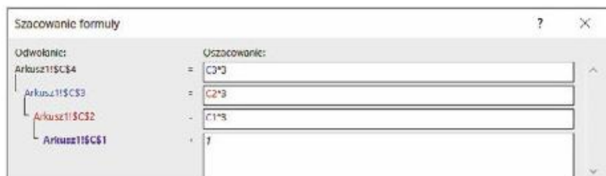
Rys. 10.6. Podgląd wywołań rekurencyjnych w narzędziu Szacuj formułę
