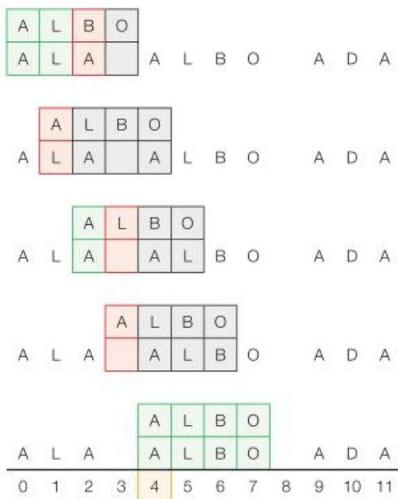
Rys. 6.7. Naiwne wyszukiwanie wzorca w tekście
