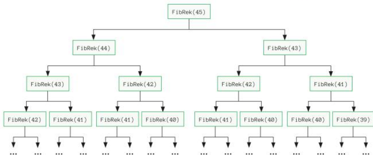
Rys. 5.11. Schemat wywołań rekurencyjnych funkcji FibRek dla n = 45
