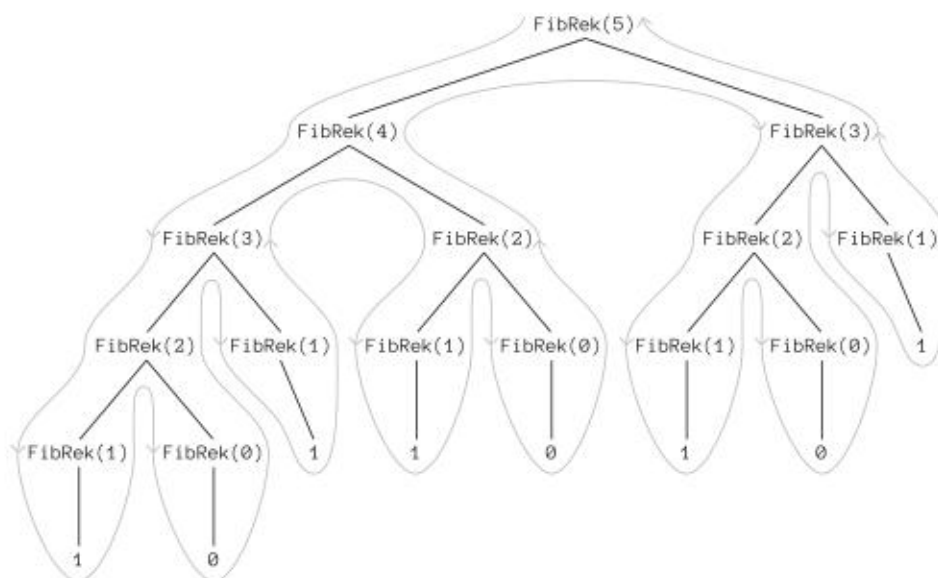
Rys. 5.12. Drzewo wywołań rekurencyjnych funkcji FibRek dla n = 5
