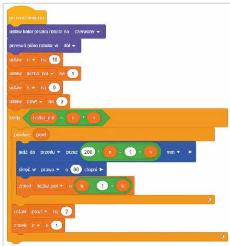
Rys. 11.25. Kod źródłowy programu Wszystkie pola planszy
