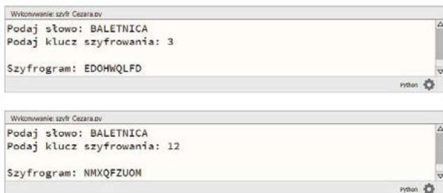
Rys. 7.8. Wywołania programu Szyfr Cezara dla kluczy 3 oraz 12
