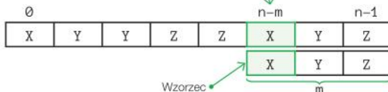
Rys. 6.8. Wyznaczenie indeksu ostatniego znaku tekstu, z którym porównujemy wzorec
