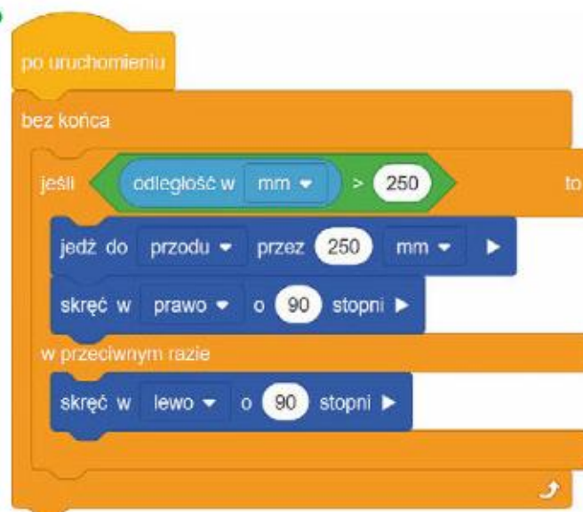
Rys. 11.27. Kod źródłowy programu Wyjście z labiryntu
