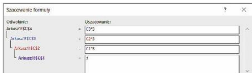
Rys. 5.6. Podgląd wywołań rekurencyjnych w narzędziu Szacuj formułę
