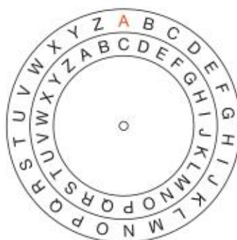
Rys. 2.7. Szyfrowanie liter szyfrem Cezara za pomocą obracających się tarcz
