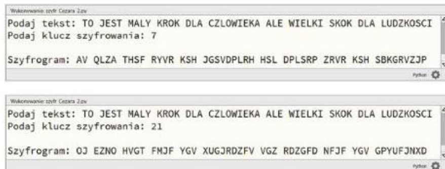
Rys. 7.9. Wywołania programu Szyfr Cezara 2
