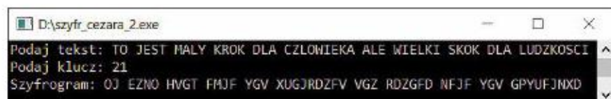
Rys. 2.9. Wywołanie programu szyfr_cezara_2.exe
