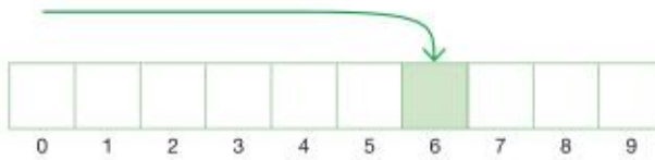
Rys. 3.4. Dostęp bezpośredni
