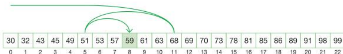
Rys. 8.6. Wyszukiwanie binarne
