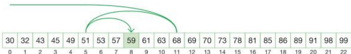
Rys. 3.6. Wyszukiwanie binarne
