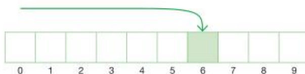
Rys. 8.4. Dostęp bezpośredni
