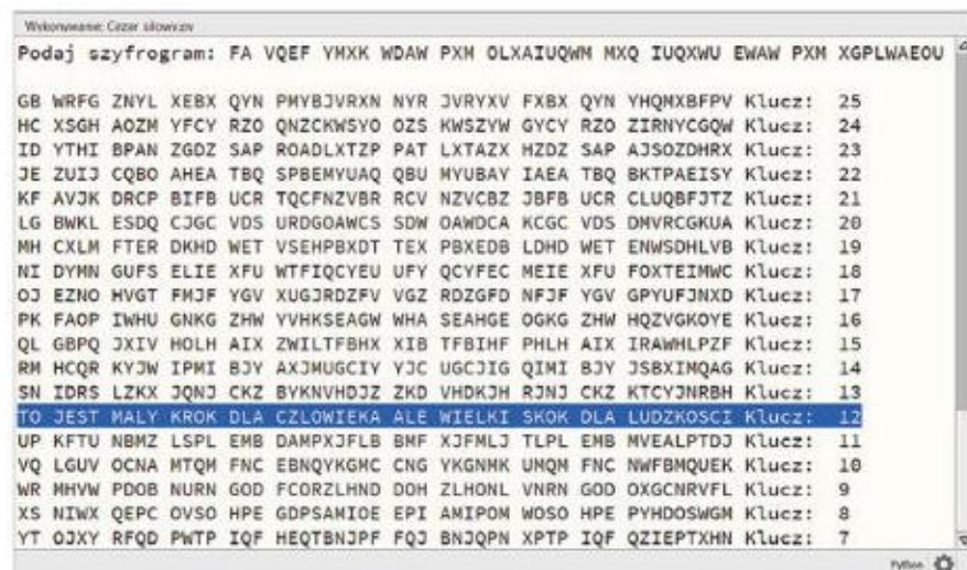
Rys. 7.10. Zastosowanie ataku siłowego do łamania szyfru Cezara
