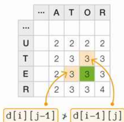
Rys. 19.14. Wybór pola przy wyznaczaniu wspólnego podciągu – analiza dwóch przypadków
