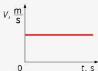
Wykres wartości prędkości od czasu w ruchu jednostajnym prostoliniowym
