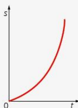
Wykres drogi od czasu trwania ruchu w ruchu jednostajnie przyspieszonym prostoliniowym
