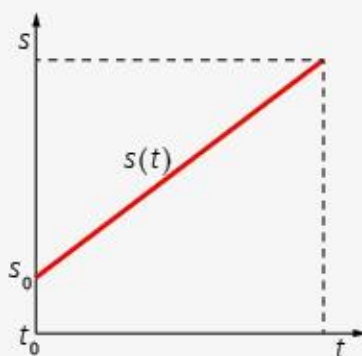
Wykres zależności przemieszczenia od czasu w ruchu jednostajnym prostoliniowym
