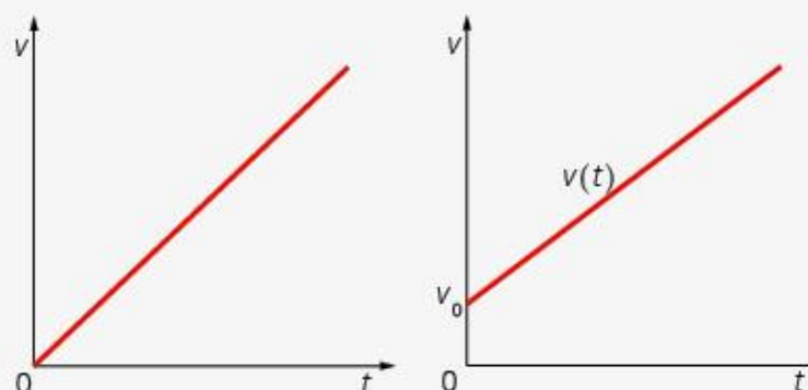
Wykresy przedstawiające zależność szybkości od czasu, gdy v_0 = 0 i v_0 > 0
