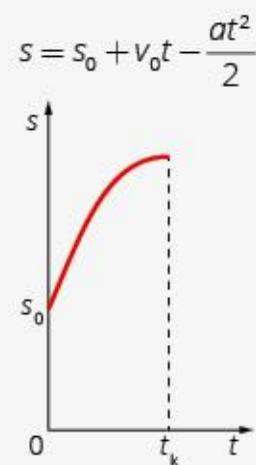
Wykresy przedstawiające zależność drogi od czasu, gdy s_0 = 0 i s_0 > 0
