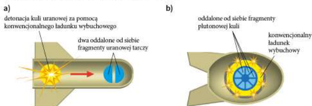
Rys. 24.8 Schemat bomby: działającej jak dział (a), implozyjnej (b)
