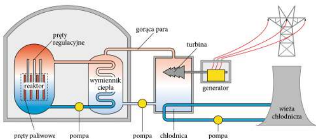
Rys. 24.3 Schemat elektrowni jądrowej
