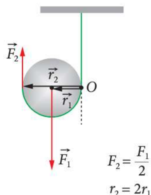
Rys. 5.5 Schemat krążka ruchomego
