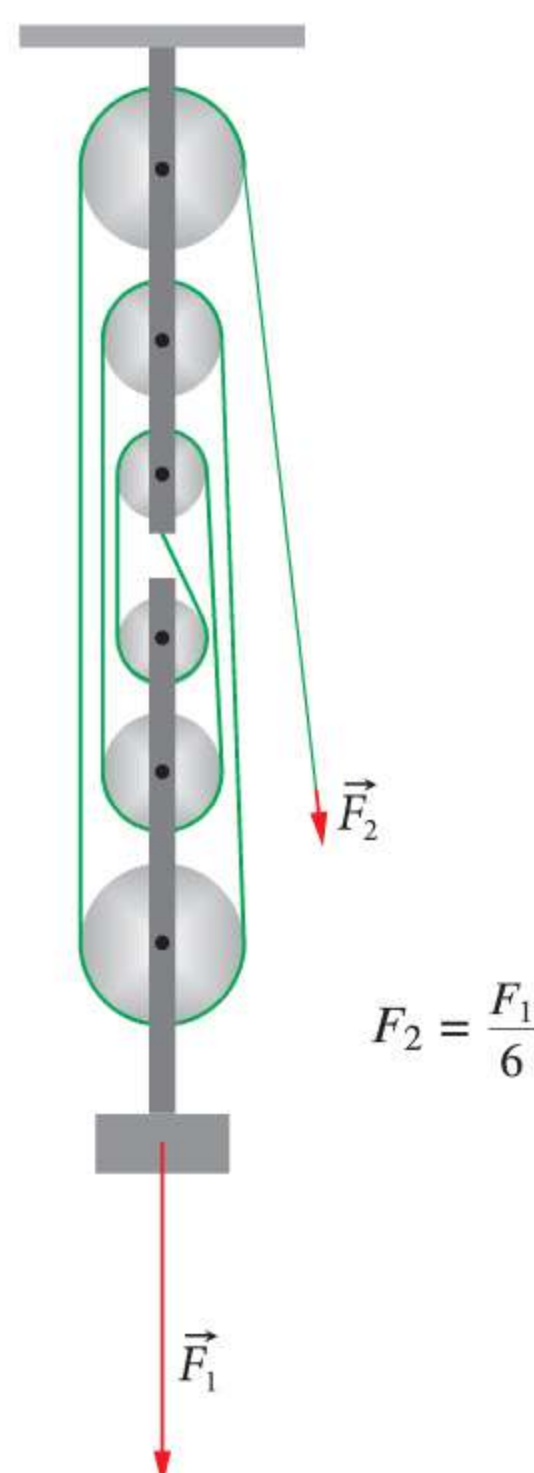
Rys. 5.7 Schemat wielokrążka
