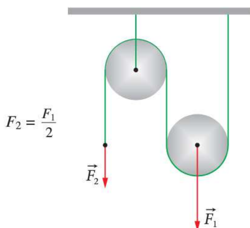
Rys. 5.6 Schemat układu krążków nieruchomego i ruchomego
