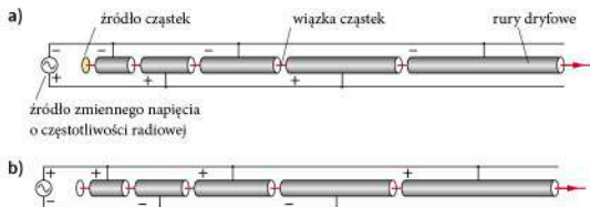
Rys. 52.4 Schemat budowy akceleratora liniowego
