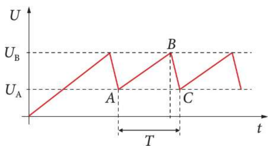
Rys. 52.2 Napięcie w generatorze podstawy czasu
