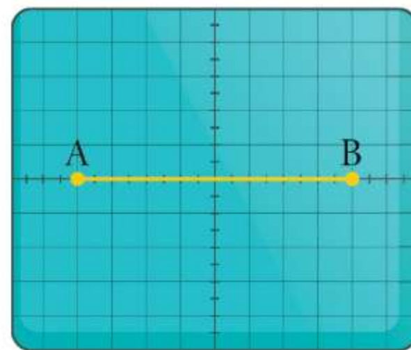
Rys. 52.3 Obraz plamki na ekranie
