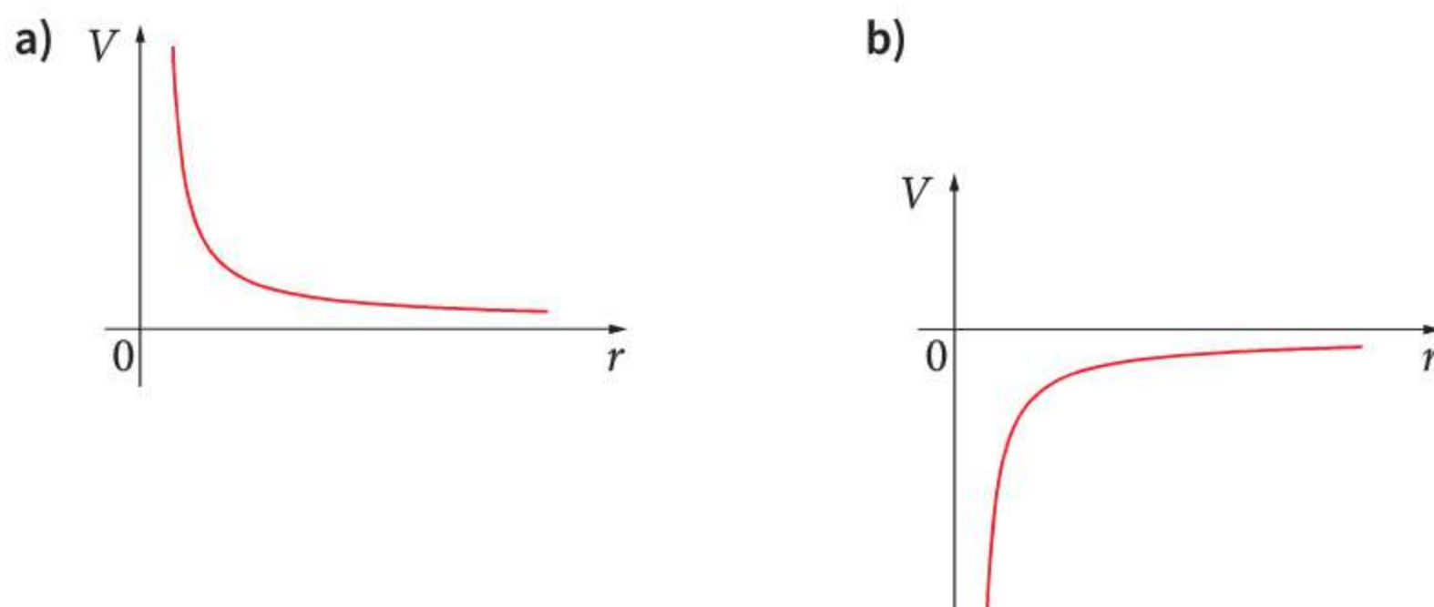
Rys. 47.2 Wykresy V(r) dla pola centralnego, gdy: Q > 0 (a), Q < 0 (b)
