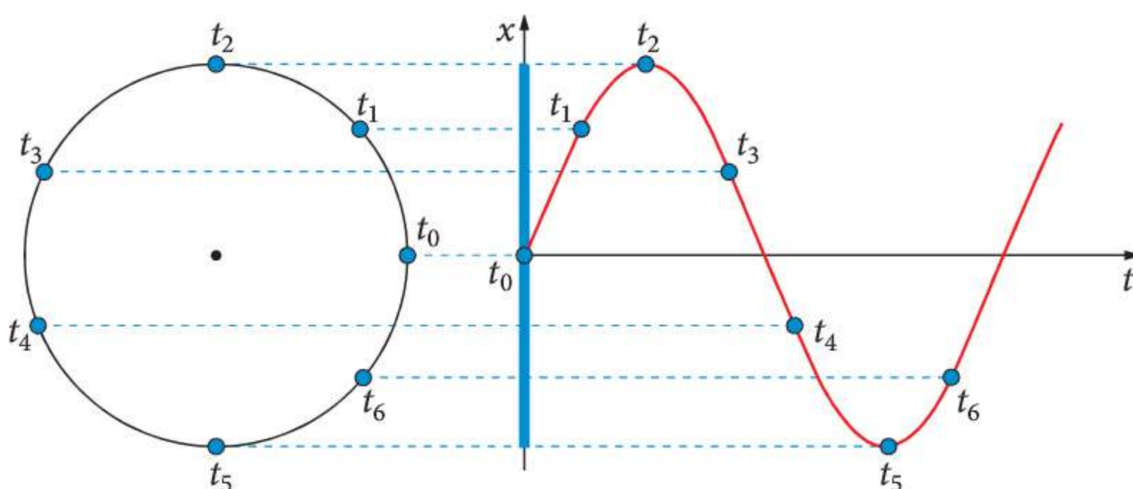
Rys. 24.2 Wykres zależności położenia cienia od czasu
