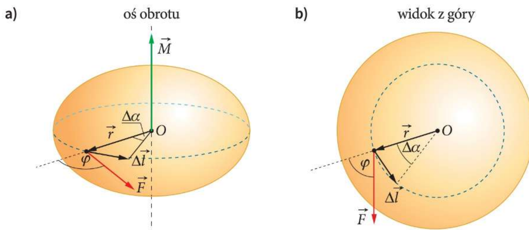
Rys. 4.7 Ilustracja wyprowadzenia wzoru na pracę momentu siły
