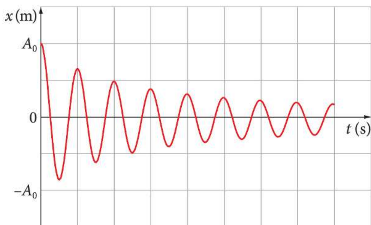
Rys. 27.3 Wykres x(t) dla ruchu drgającego tłumionego
