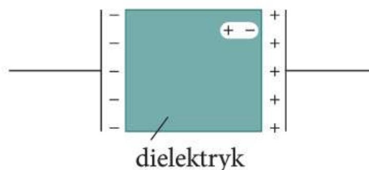
Rys. 50.4 Polaryzacja atomu dielektryka w polu elektrostatycznym
