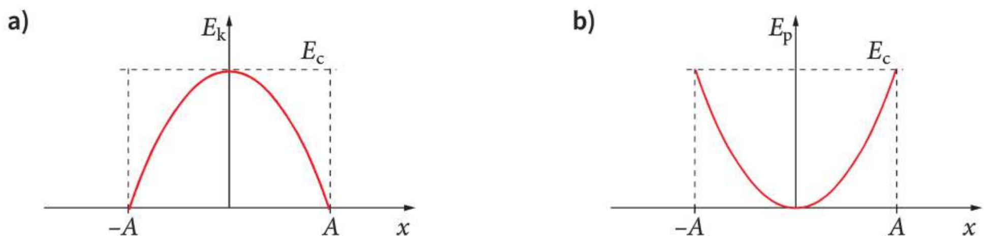
Rys. 25.3 Wykresy zależności: energii kinetycznej (a) i energii potencjalnej sprężystości (b) od wychylenia
