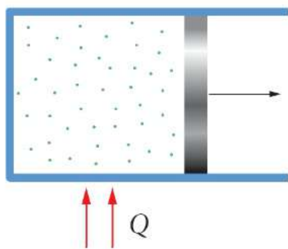
Rys. 37.1 Gaz wypycha tłok, więc wykonuje pracę dodatnią (praca siły zewnętrznej W < 0 )
