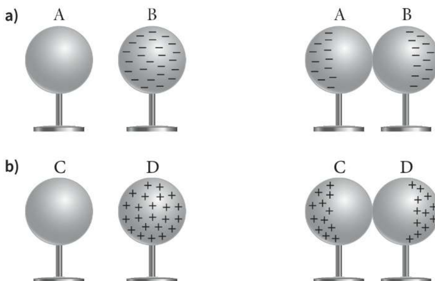
Rys. 43.2 Elektryzowanie przez zetknięcie
