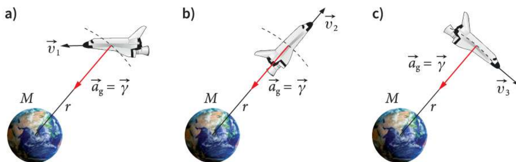
Rys. 12.8 Przyspieszenie grawitacyjne promu kosmicznego a natężenie pola grawitacyjnego
