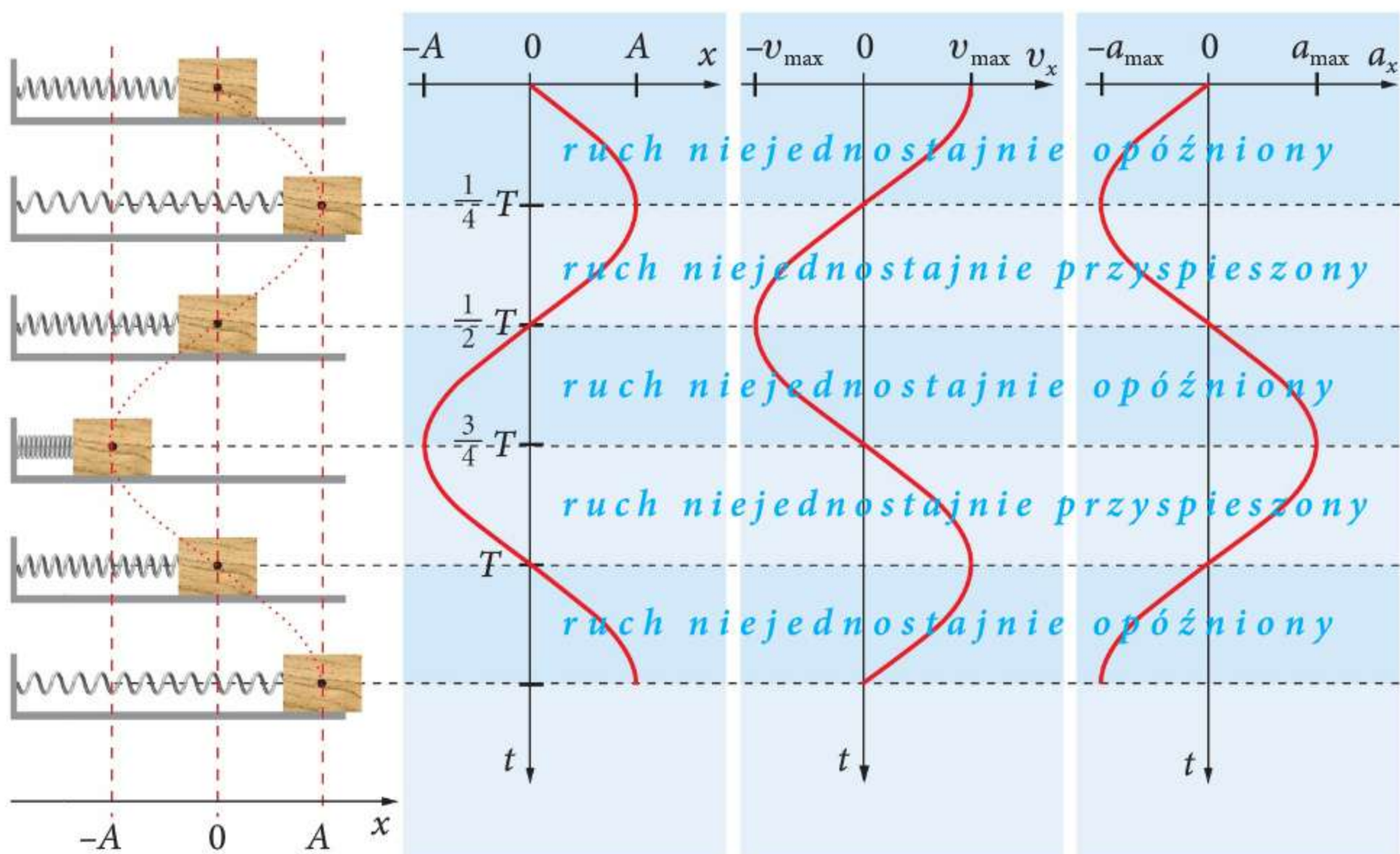
Rys. 24.9 Wykresy zależności: x(t) , v_x(t) i a_x(t) dla ruchu harmonicznego
