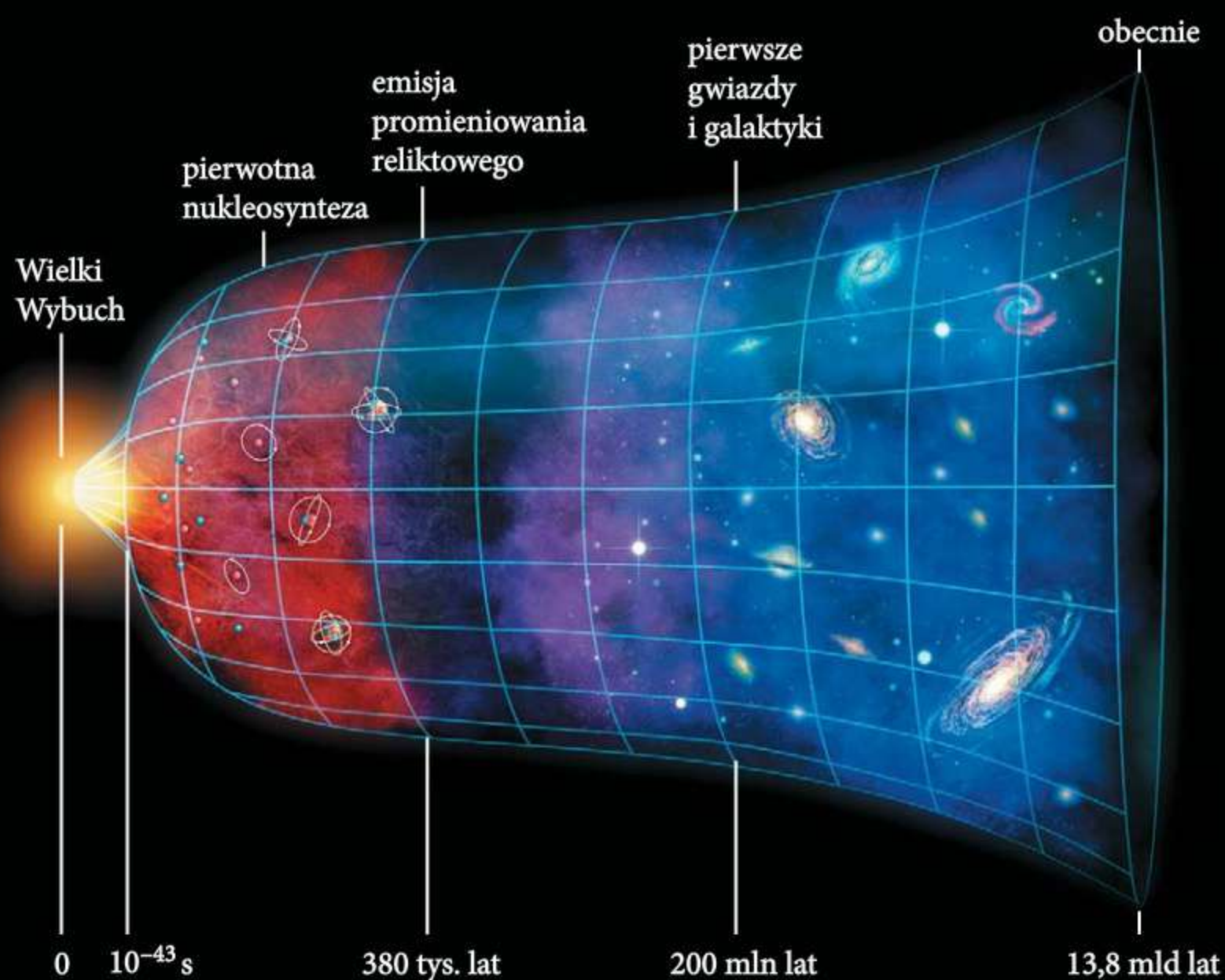
Rys. 21.4 Schematyczne przedstawienie ewolucji Wszechświata
