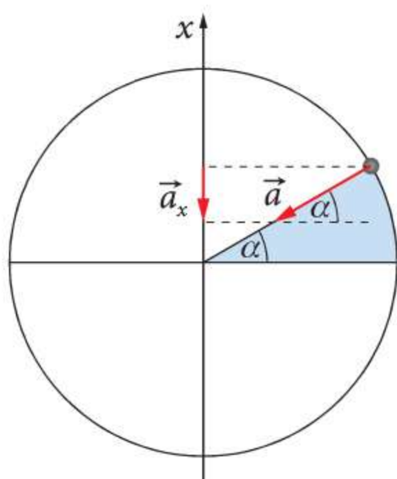
Rys. 24.5 Ilustracja wyprowadzenia zależności a_x(t)
