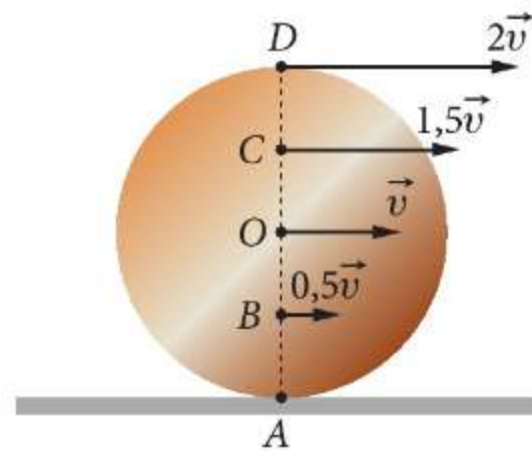
Rys. 8.2 Prędkości wybranych punktów podczas toczenia
