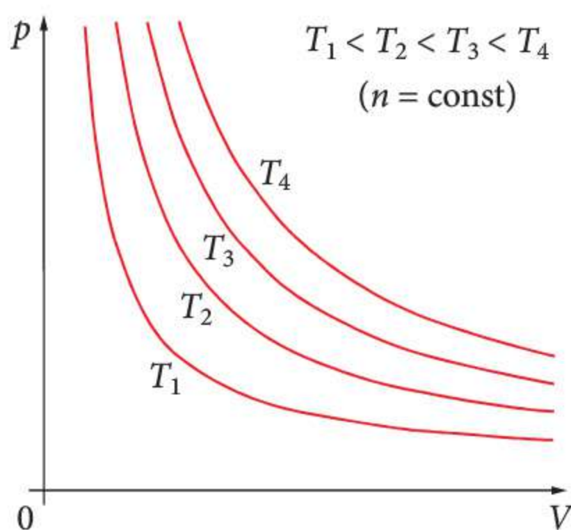
Rys. 31.1 Izotermy gazu doskonałego dla różnych temperatur
