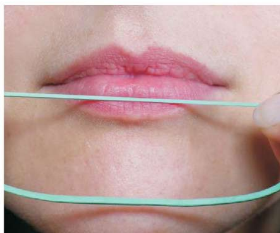
Rys. 22.2 Zamiana energii potencjalnej sprężystości w energię wewnętrzną
