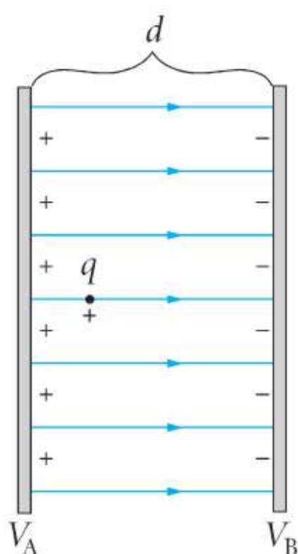
Rys. 49.1 Pole elektrostatyczne w kondensatorze płaskim
