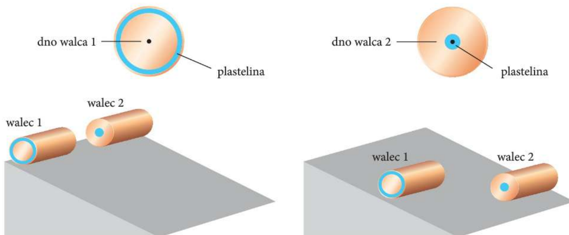
Rys. 3.1 Ruch walców o różnych momentach bezwładności
