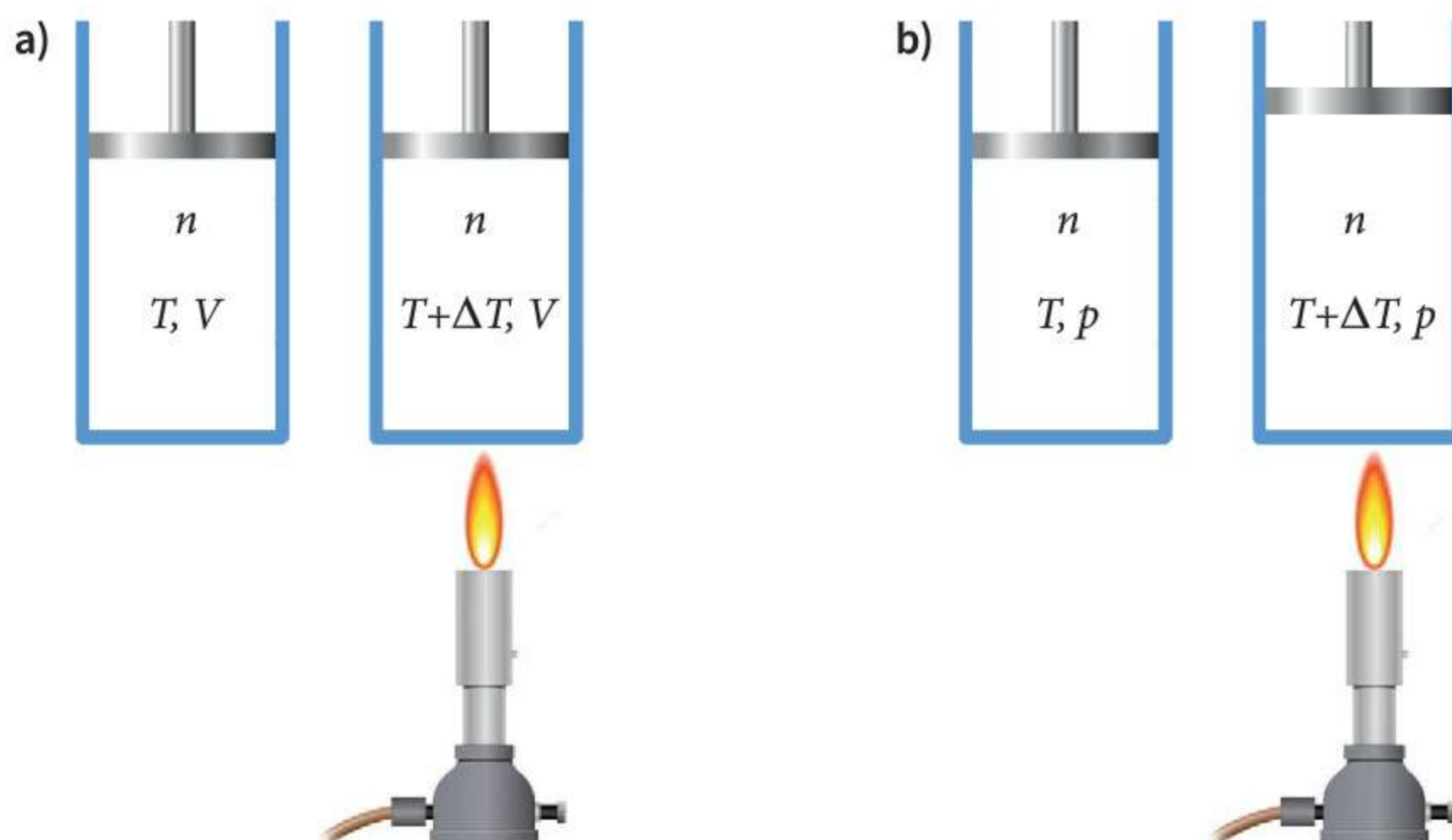
Rys. 35.1 Zwiększanie energii wewnętrznej gazu: w stałej objętości (a), przy stałym ciśnieniu (b)
