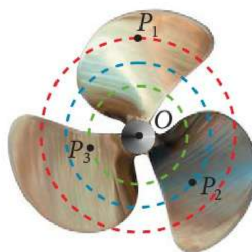
Rys. 2.2 Przykład ruchu obrotowego bryły sztywnej
