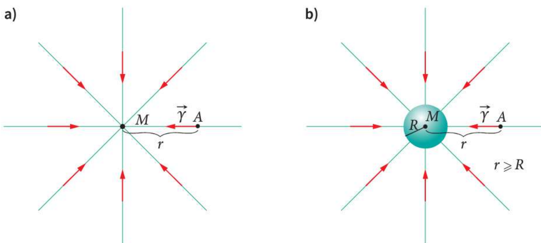
Rys. 12.3 Natężenia obu pól w punkcie A są jednakowe
