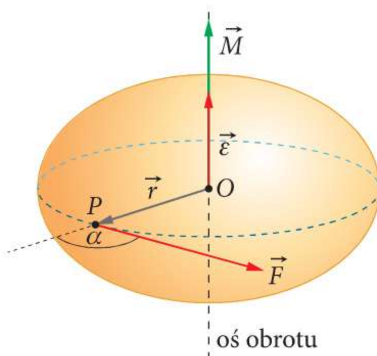
Rys. 4.3 Kierunek i zwrot momentu siły i przyspieszenia kątownego bryły
