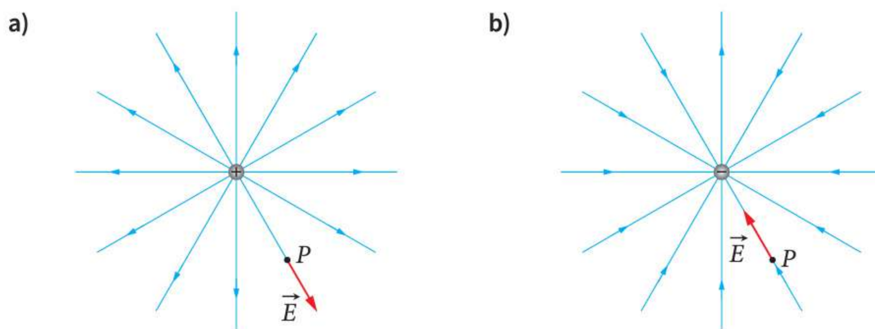
Rys. 44.1 Centralne pola elektrostatyczne utworzone przez: ładunek dodatni (a), ładunek ujemny (b)
