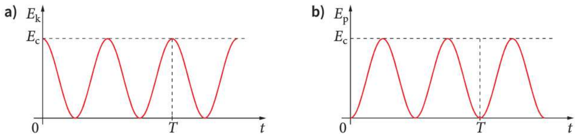
Rys. 25.2 Wykresy zależności: energii kinetycznej (a) i energii potencjalnej sprężystości (b) od czasu
