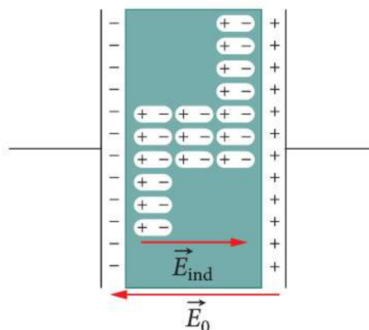
Rys. 50.5 Indukowanie pola wewnątrz dielektryka umieszczonego w polu elektrostatycznym; E_{\text{ind}} \neq E
