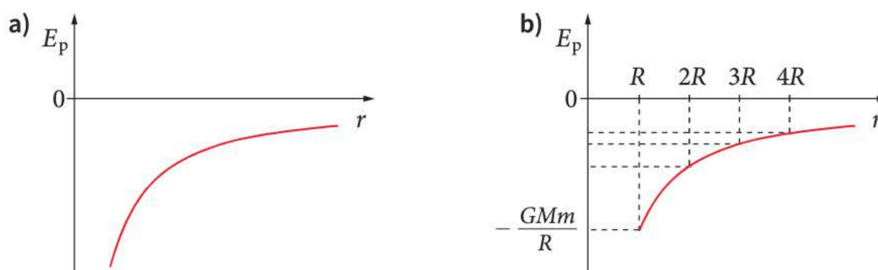
Rys. 14.3 Wykres E_p(r) dla ciała w polu grawitacyjnym: źródła punkowego (a), jednorodnej kuli (b)
