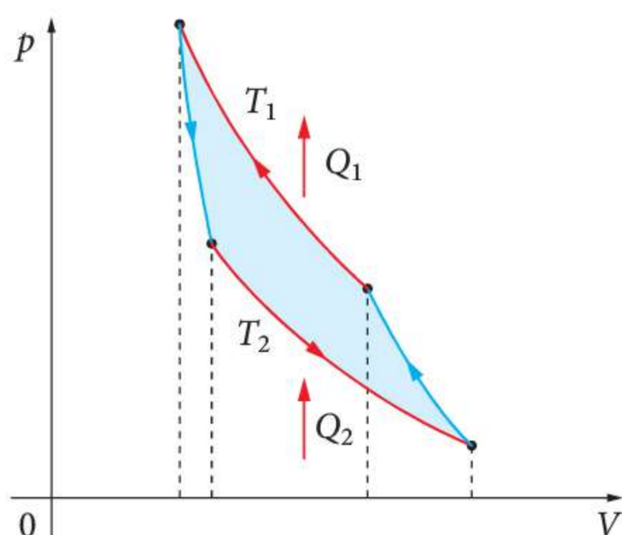
Rys. 37.8 Cykl pracy chłodziarki (odwrotny do cyklu Carnota)
