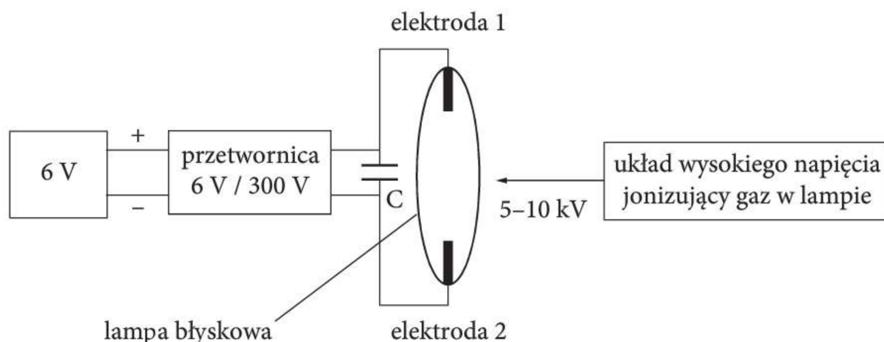
Rys. 51.1 Schemat układu z lampą błyskową
