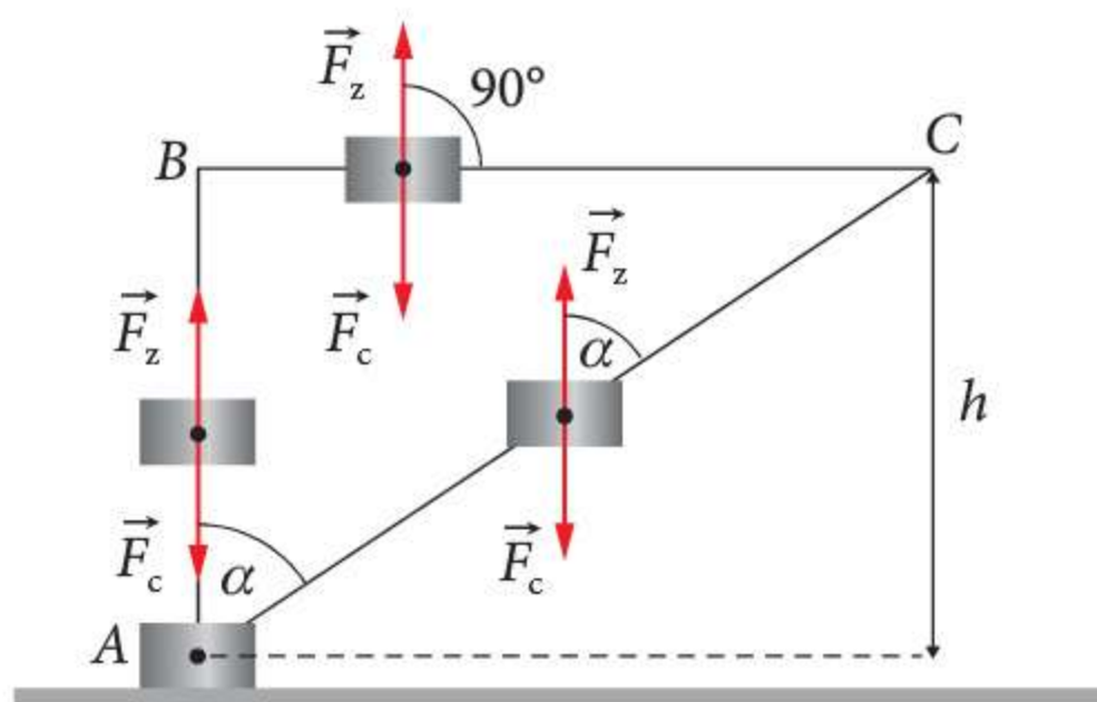
Rys. 13.1 Różne tory ciała przemieszczanego od punktu A do punktu C
