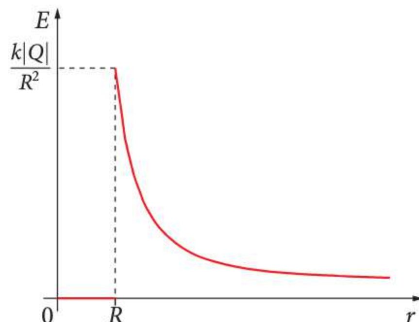
Rys. 45.4 Wykres E(r) dla naładowanej kuli
