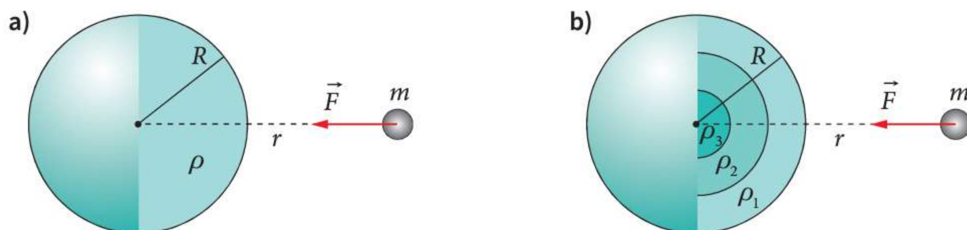
Rys. 10.1 Kule o sferycznym symetrycznym rozkładzie masy: jednorodna (a), składająca się z warstw o różnych gęstościach (b)
