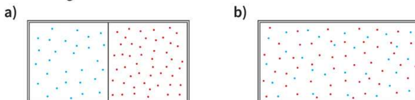
Rys. 38.1 Różne gazy w pojemniku z przegrodą – stan początkowy (a); stan końcowy po usunięciu przegrody (b)
