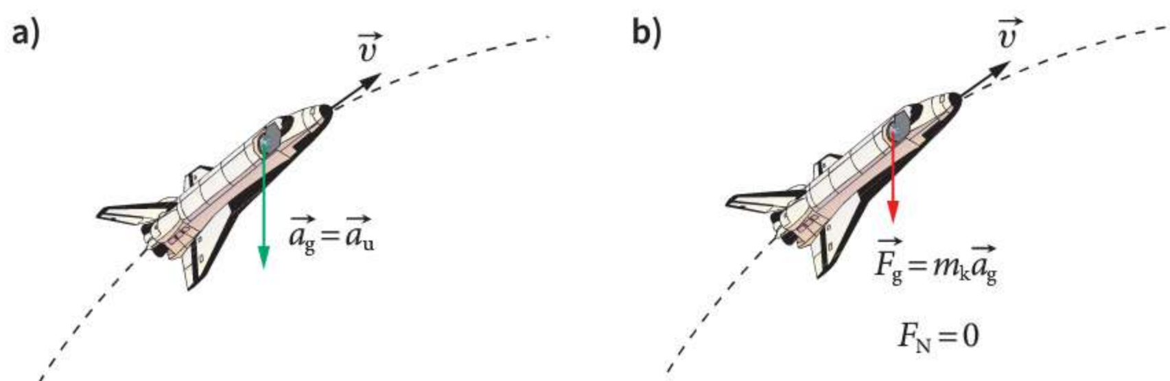
Rys. 17.4 Przyspieszenie kosmonauty w rakiecie poruszającej się bez napędu (a) oraz działająca na niego siła grawitacji (b)
