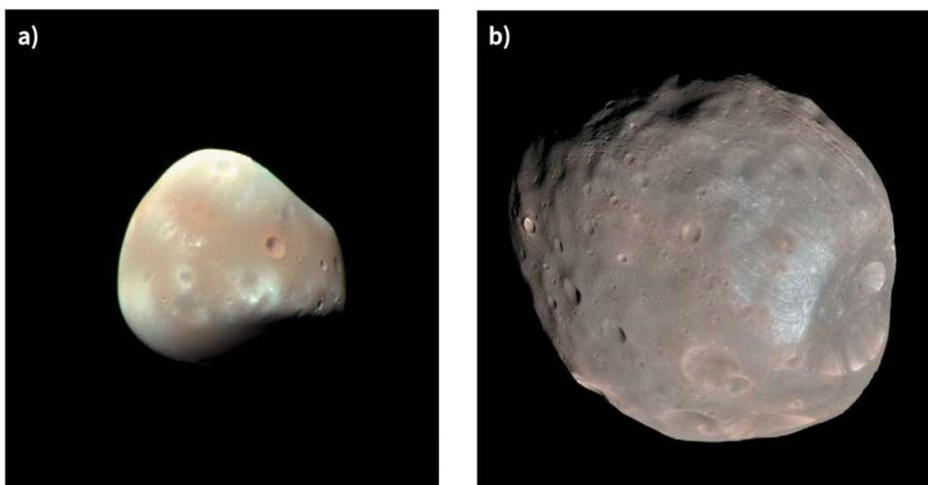
Rys. 18.3 Księżyce Marsa: Deimos (a), Fobos (b)
