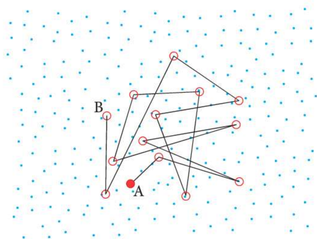
Rys. 38.2 Ruchy Browna
