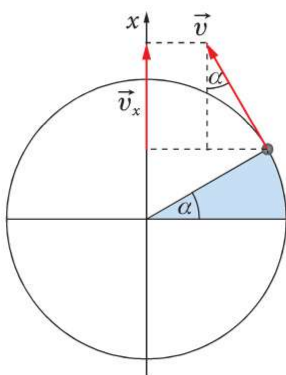
Rys. 24.4 Ilustracja wyprowadzenia zależności v_x(t)
