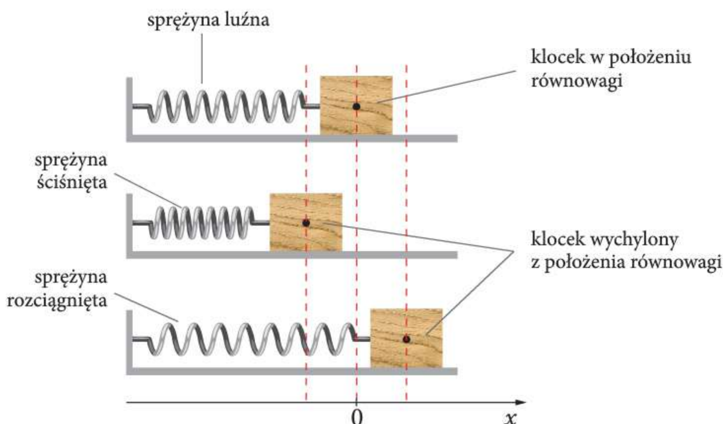
Rys. 23.1 Drgania klocka na śliskiej, poziomej powierzchni
