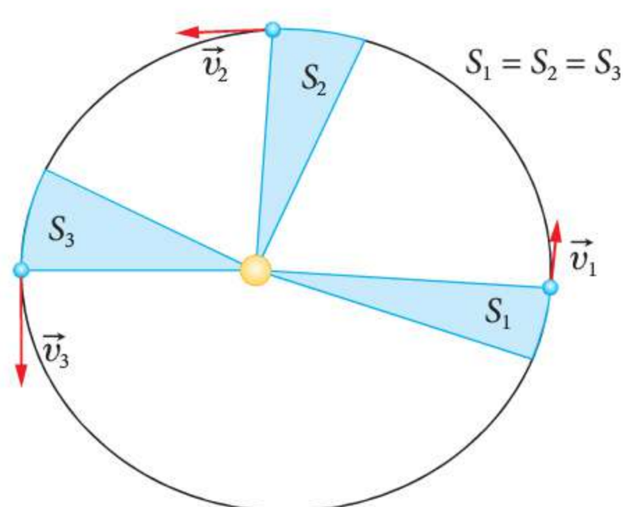
Rys. 9.6 Prędkość planety w różnych punktach toru
