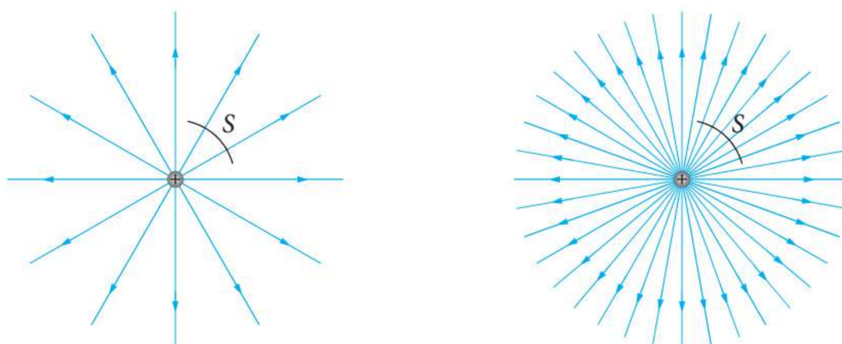
Rys. 44.2 Centralne pola elektrostatyczne o różnych natężeniach
