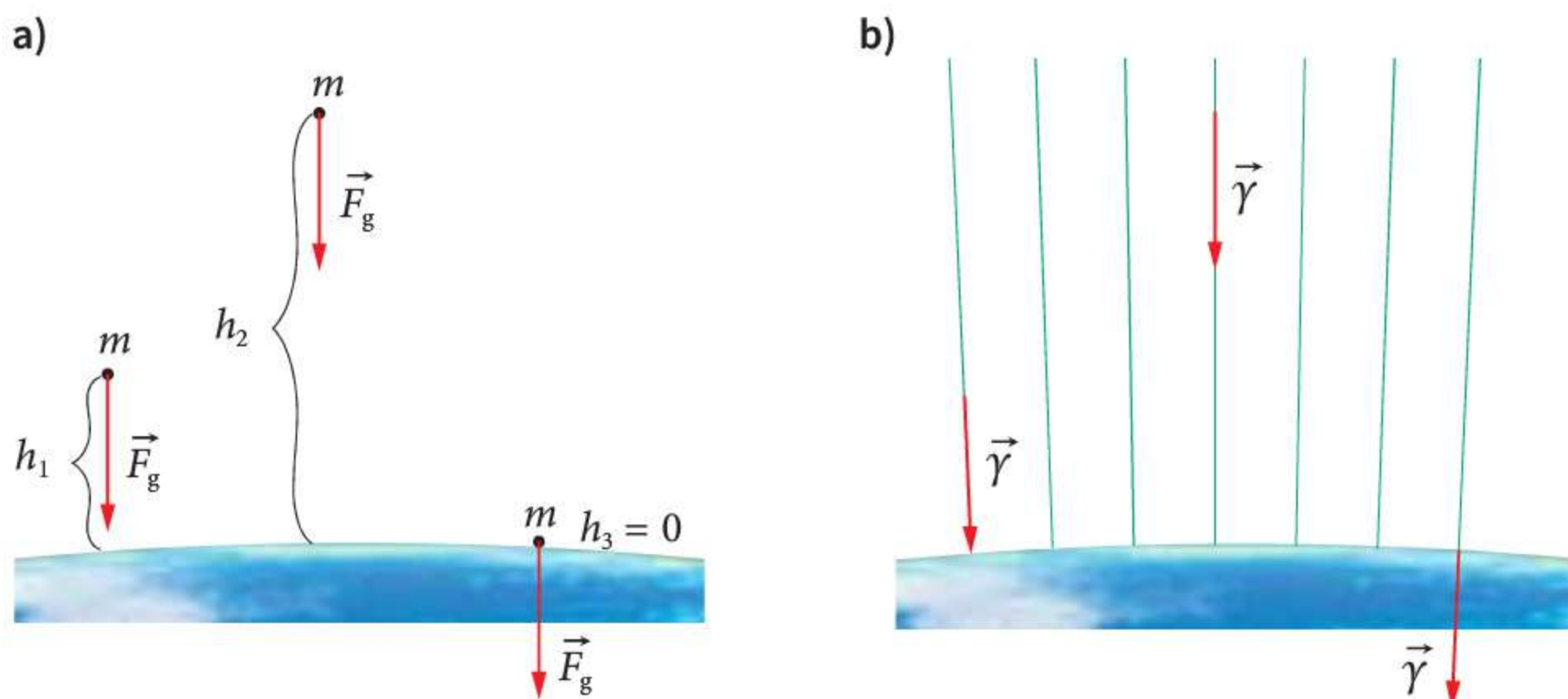
Rys. 12.7 Siły grawitacji (a) oraz natężenie pola grawitacyjnego (b) w pobliżu Ziemi
