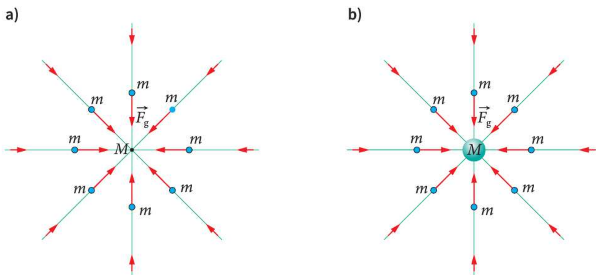
Rys. 12.1 Pola centralne: punktu materialnego (a), jednorodnej kuli (b)
