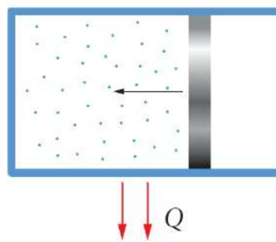
Rys. 37.2 Sprężanie gazu; pracę dodatnią wykonuje siła zewnętrzna ( W > 0 )
