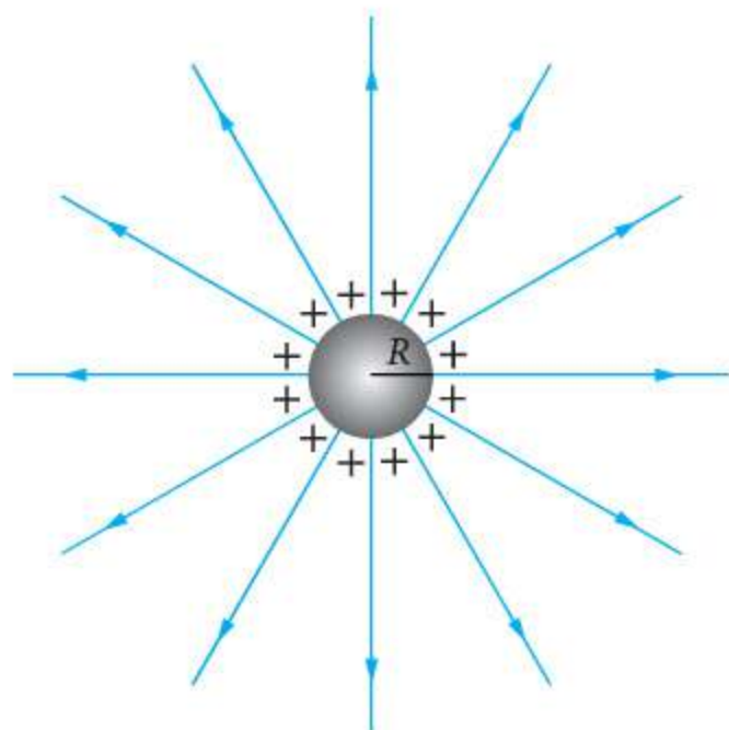
Rys. 45.3 Pole elektrostatyczne na zewnątrz kuli o promieniu R
