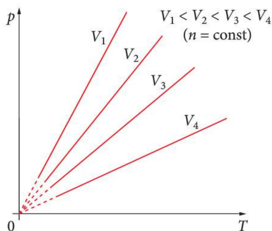
Rys. 31.2 Izochory gazu doskonałego dla różnych objętości
