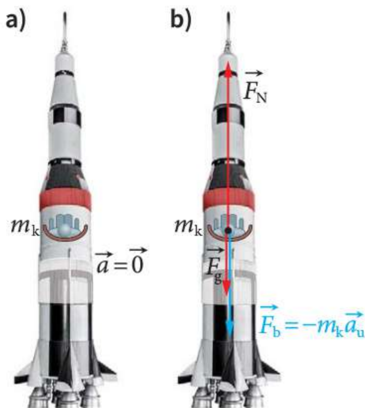
Rys. 17.2 Przyspieszenie kosmonauty w startującej rakiecie (a) oraz działające na niego siły (b) – względem układu nieinercjalnego rakiety
