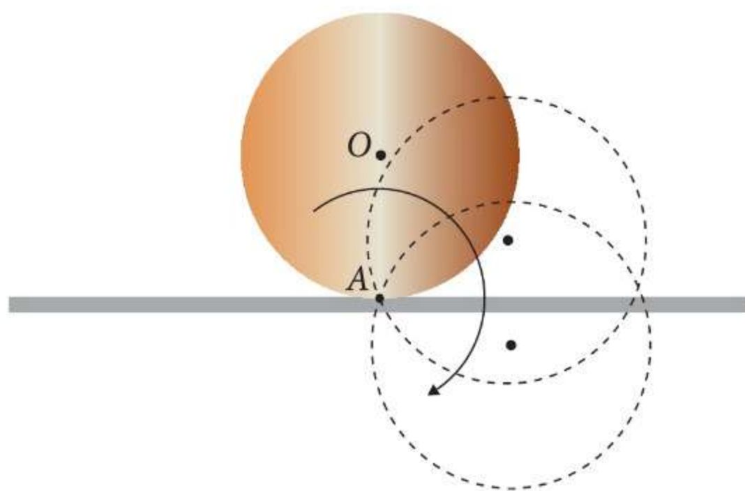
Rys. 8.3 Toczenie jako obrót względem chwilowej osi obrotu
