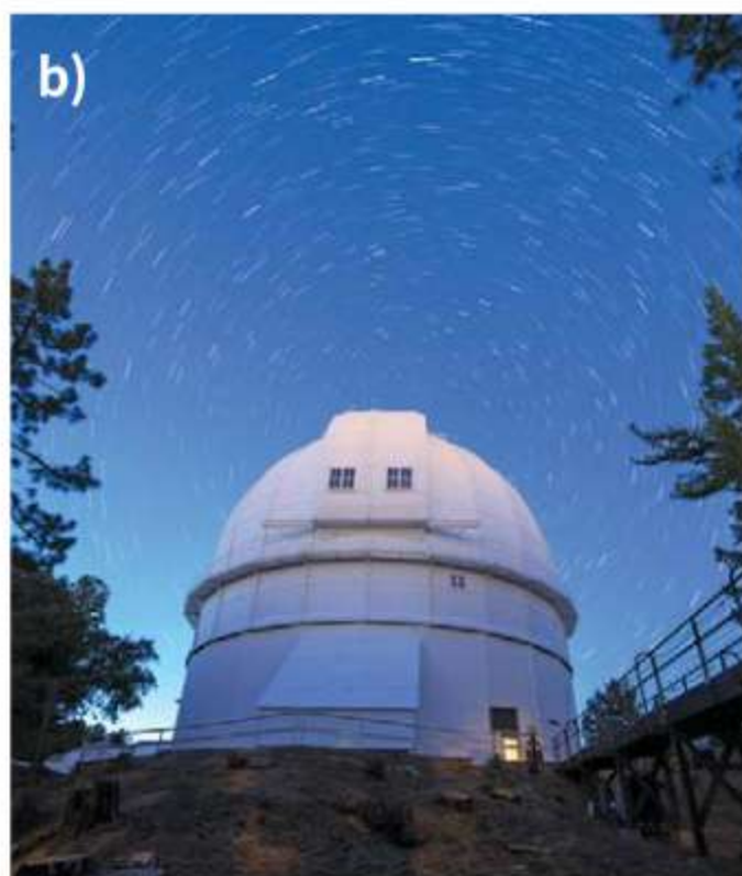
Rys. 21.1 Edwin Hubble (a) oraz obserwatorium, w którym pracował (b)
