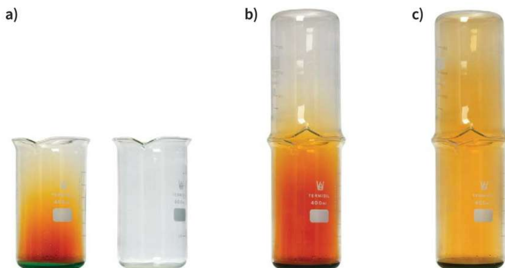
Rys. 28.1 Kolejne etapy dyfuzji w gazie
