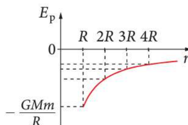
źródłem pola jest ciało kuliste
