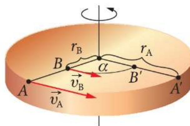
Rys. 2.4 Prędkości wybranych punktów obracającego się walca
