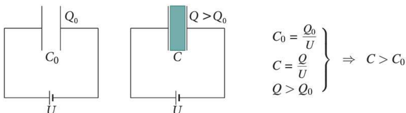
Rys. 50.3 Wpływ dielektryka na pojemność kondensatora połączzonego ze źródłem napięcia
