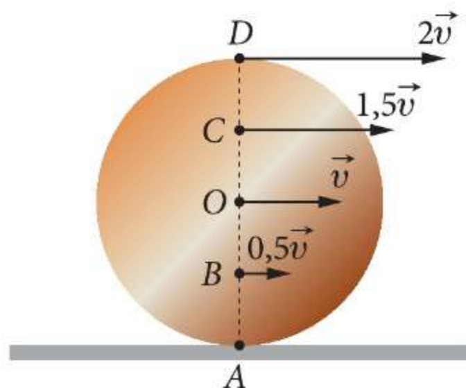
Rys. 8.2 Prędkości wybranych punktów podczas toczenia
