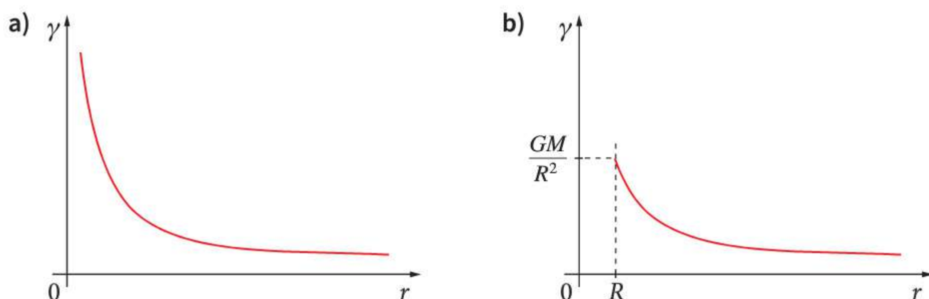
Rys. 12.4 Wykres \gamma(r) : dla źródła punkowego (a), na zewnątrz jednorodnej kuli o masie M i promieniu R (b)
