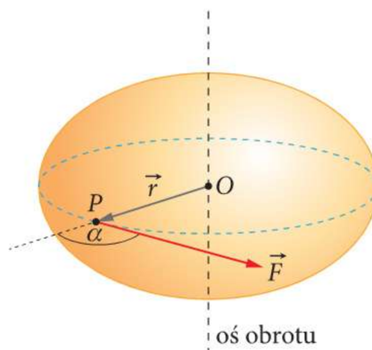
Rys. 4.2 Przykład siły powodującej obrót bryły
