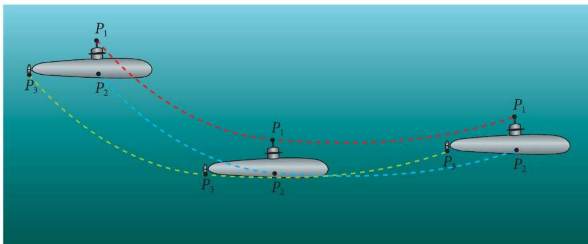
Rys. 2.1 Przykład ruchu postępowego bryły sztywnej
