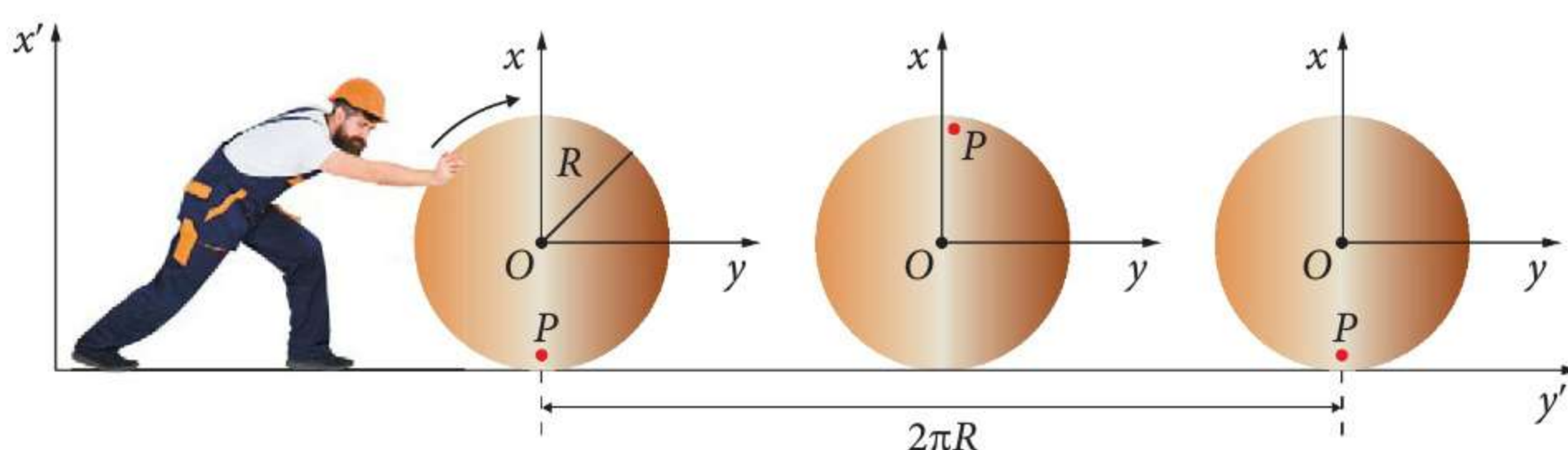
Rys. 2.3 Toczenie bryły obrotowej
