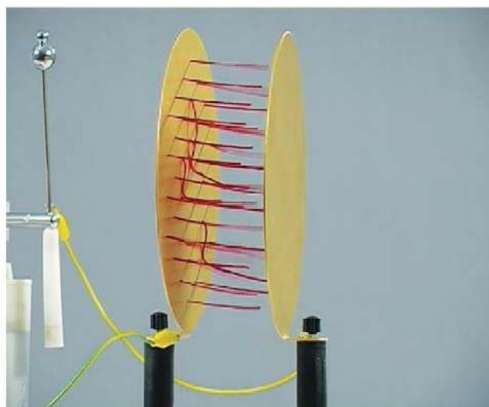
Rys. 44.4 Jednorodne pole elektrostatyczne
