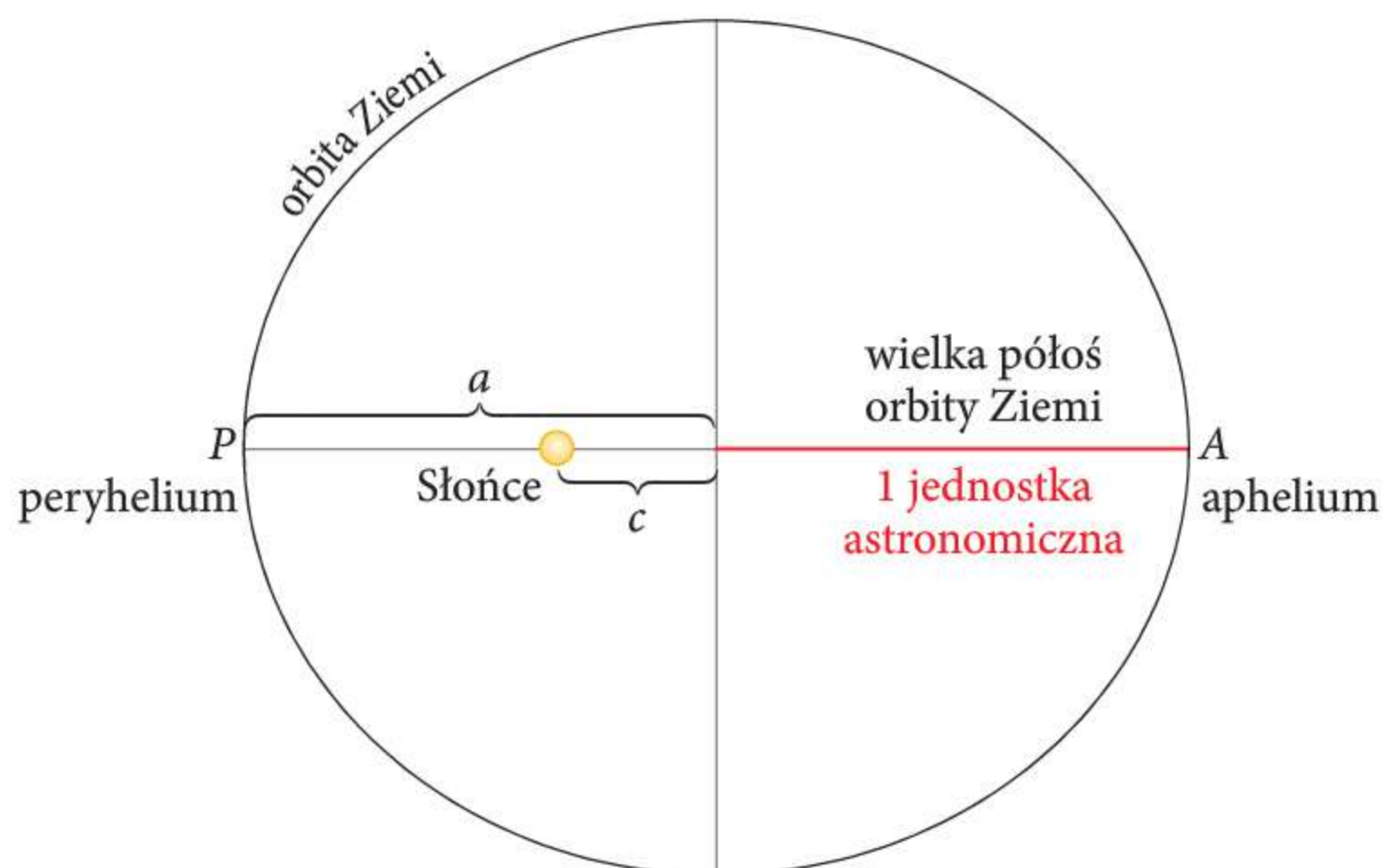
Rys. 19.1 Ilustracja definicji jednostki astronomicznej
