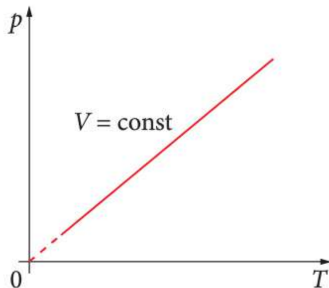
Rys. 40.1 Zależność ciśnienia pary nienasyconej (w stałej objętości) od temperatury
