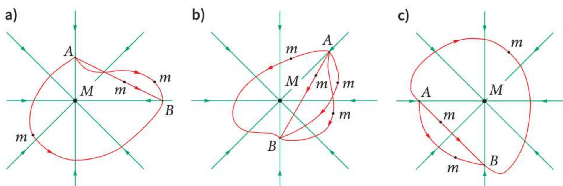
Rys. 14.1 Różne tor 8 ciała przemieszczanego od punktu A do punktu B w polu centralnym: r_B > r_A \Rightarrow \Delta E_p > 0 (a), r_B < r_A \Rightarrow \Delta E_p < 0 (b), r_B = r_A \Rightarrow \Delta E_p = 0 (c)
