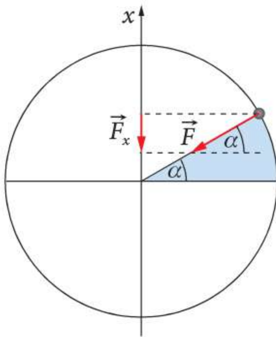
Rys. 24.6 Ilustracja wyprowadzenia zależności F_x(t)
