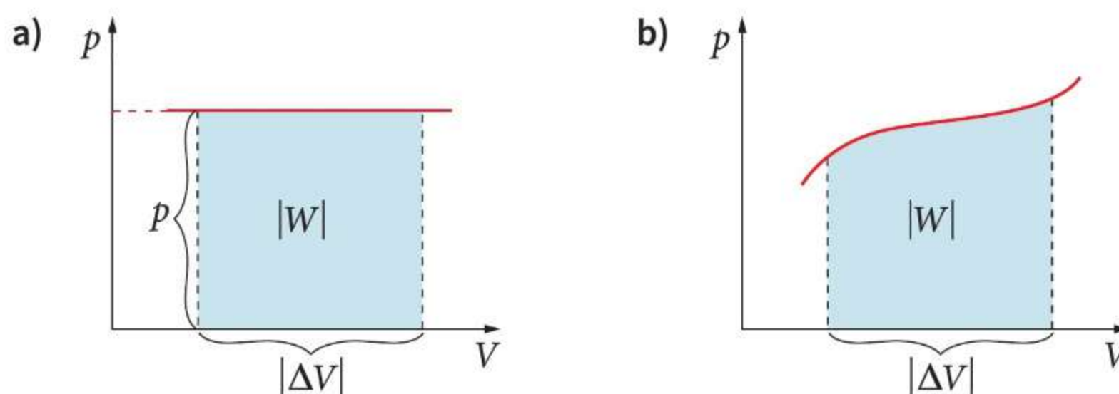
Rys. 33.3 Praca objętościowa: w przemianie izobarycznej (a), w dowolnej przemianie gazu (b)
