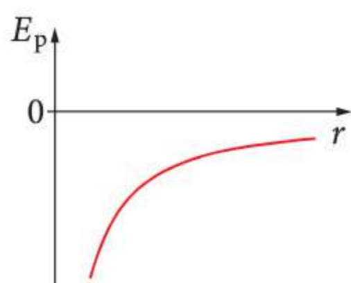
punktowe źródło pola
