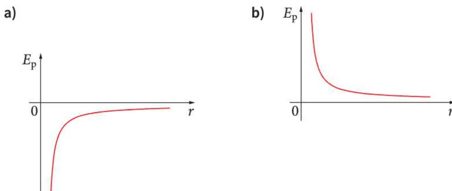
Rys. 47.1 Wykresy E_p(r) dla pola ładunku punkowego, gdy: Qq < 0 (a), Qq > 0 (b)
