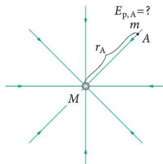
Rys. 14.2 Ilustracja definicji energii potencjalnej ciała w centralnym polu grawitacyjnym
