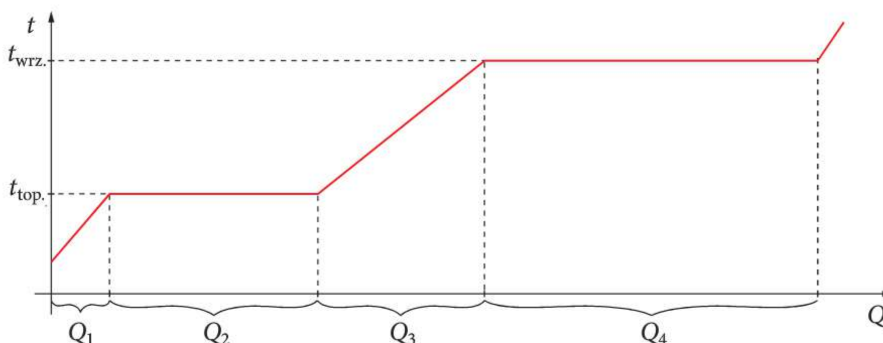
Rys. 39.2 Zależność temperatury substancji od ilości dostarczonego ciepła
