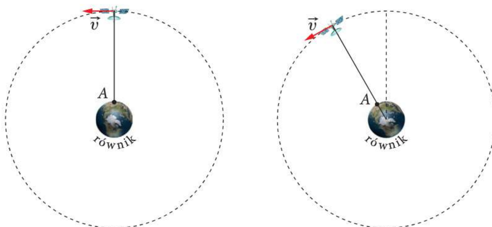
Rys. 11.3 Położenie satelity geostacjonarnego w dwóch różnych chwilach
