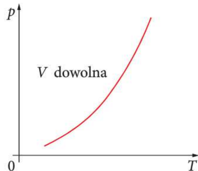
Rys. 40.2 Zależność ciśnienia pary nasyconej od temperatury; objętość dowolna, gdyż ciśnienie pary nasyconej nie zależy od objętości
