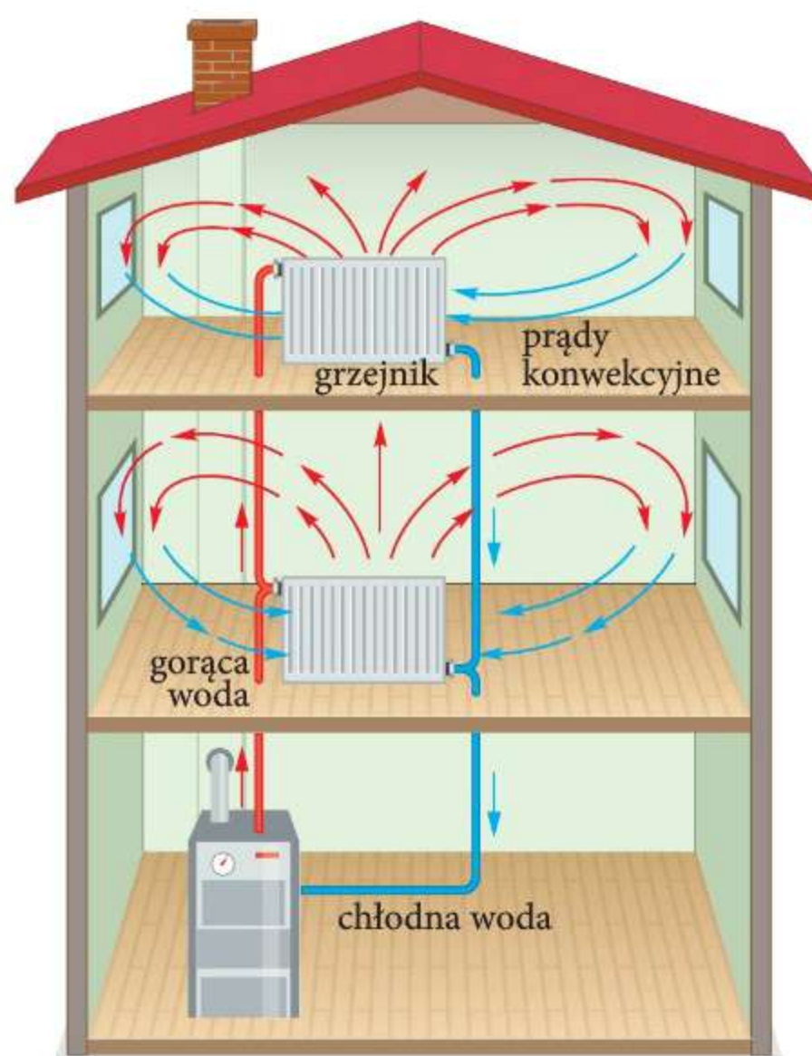
Rys. 42.7 Prądy konwekcyjne w powietrzu wewnątrz ogrzewanego budynku
