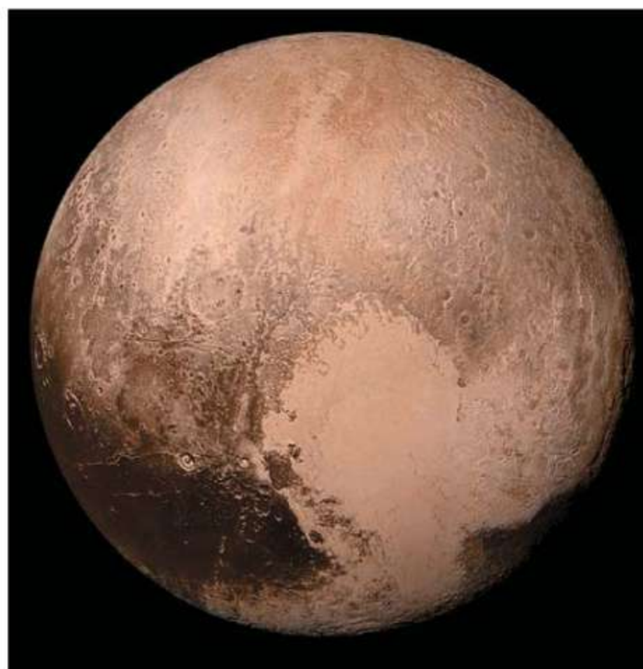
Rys. 18.9 Planeta karłowata Pluton
