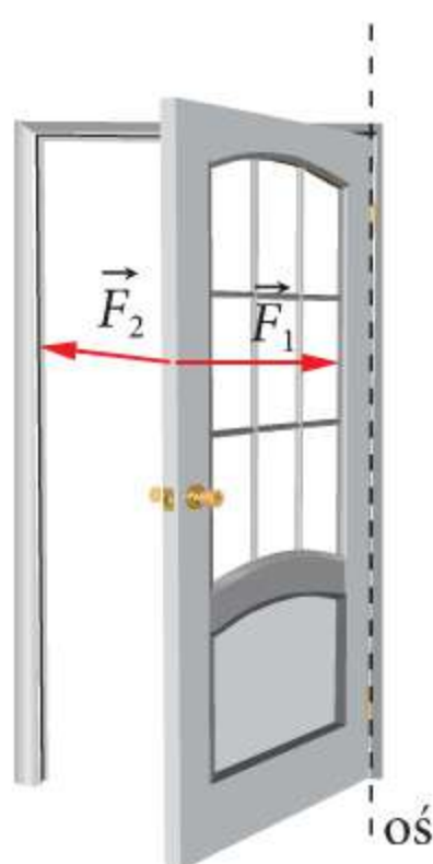
Rys. 4.1 Która z sił spowoduje obrót drzwi?
