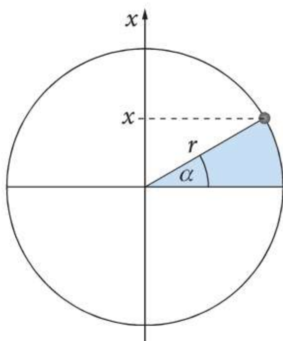
Rys. 24.3 Ilustracja wyprowadzenia zależności x(t)
