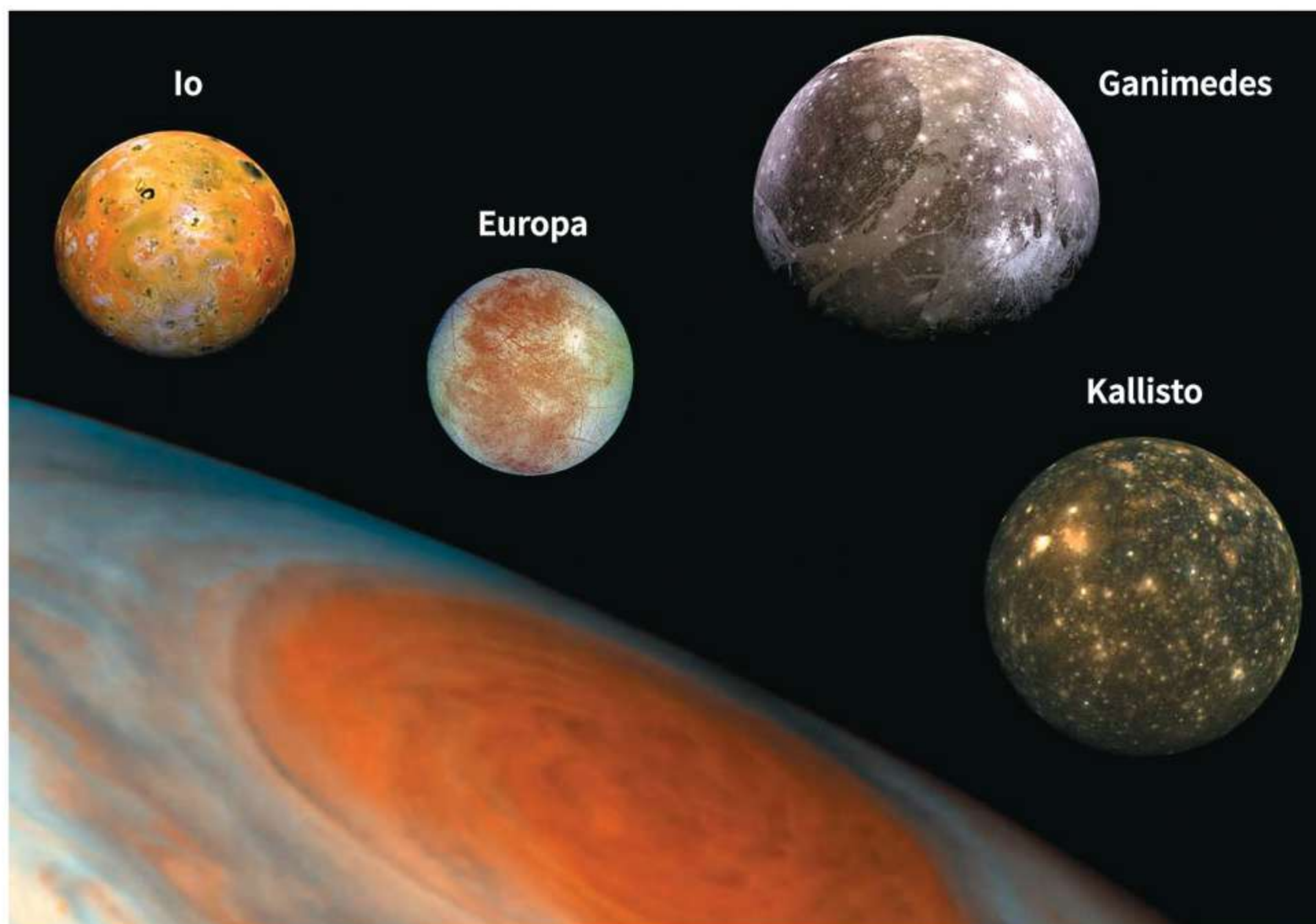
Rys. 18.4 Galileuszowe księżyce Jowisza
