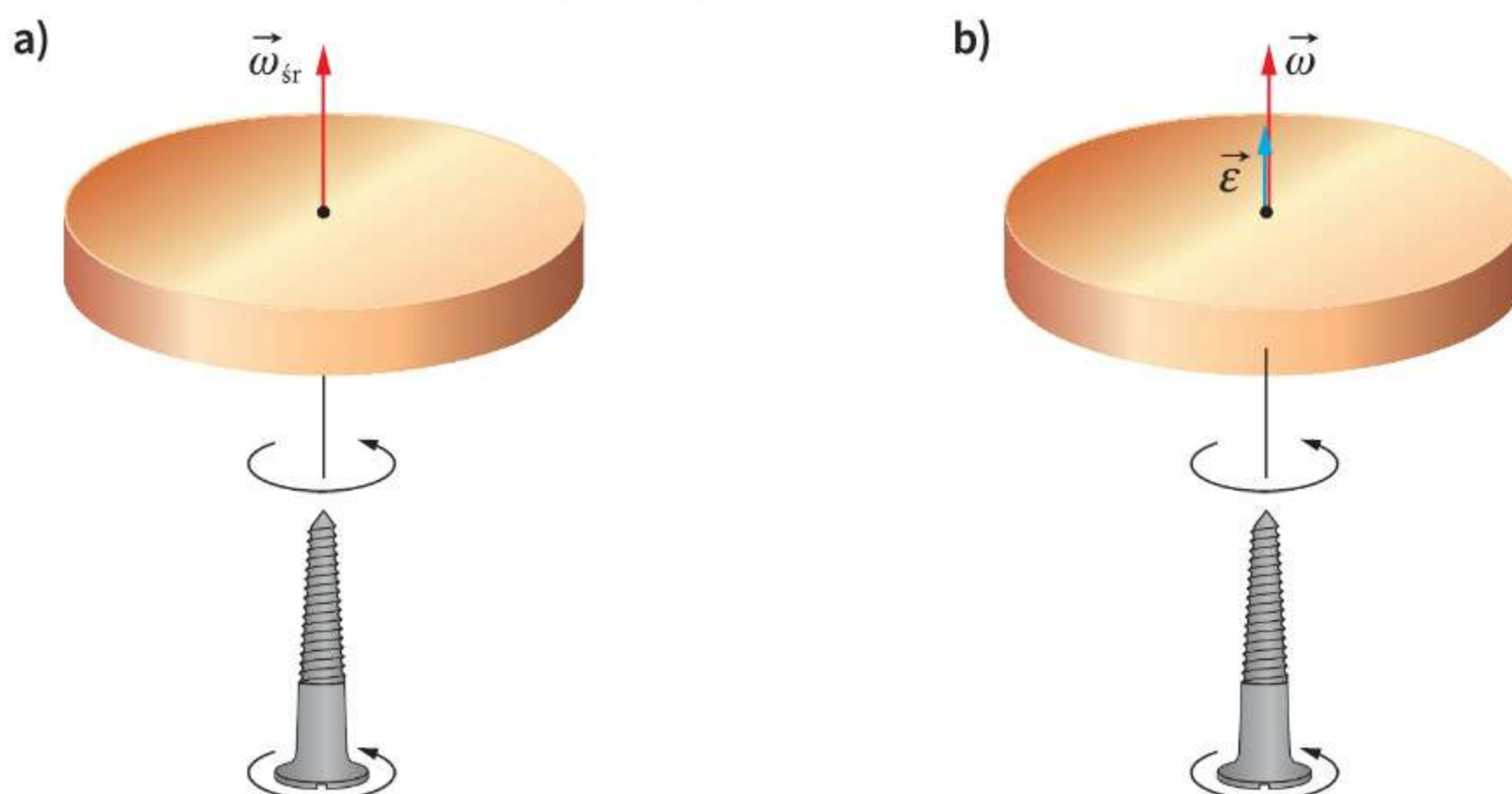
Rys. 2.5 Wyznaczanie zwrotu wektorów: prędkości kątowej średniej (a), prędkości kątowej i przyspieszenia kątowego (b)
