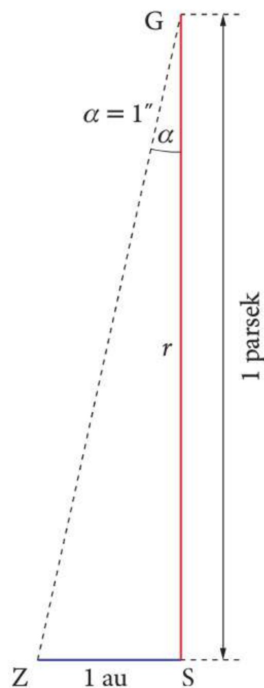
Rys. 19.4 Ilustracja definicji parseka
