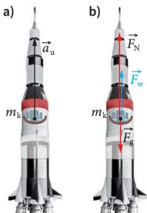
Rys. 17.1 Przyspieszenie kosmonauty w startującej rakiecie (a) oraz działające na niego siły (b) – względem układu inercjalnego Ziemi
