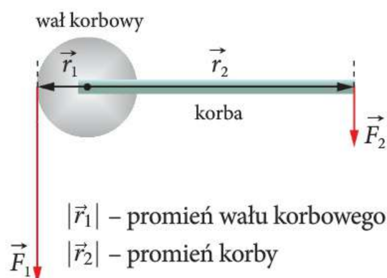
Rys. 5.8 Schemat kołowrotu
