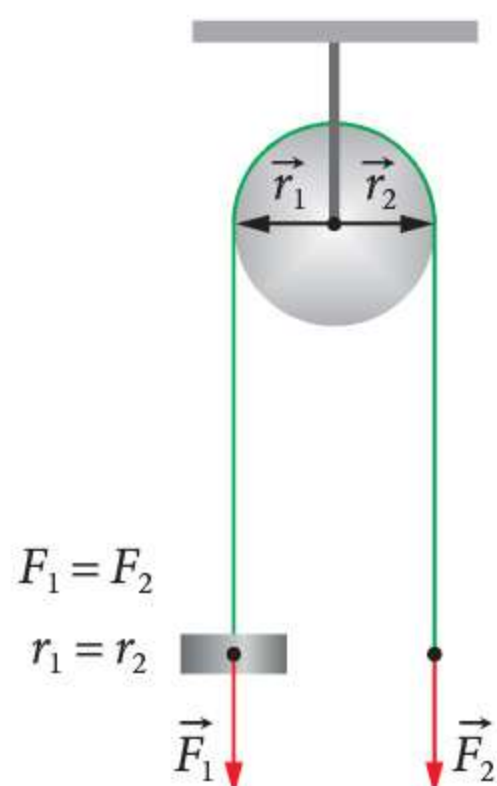
Rys. 5.4 Schemat krążka nieruchomego
