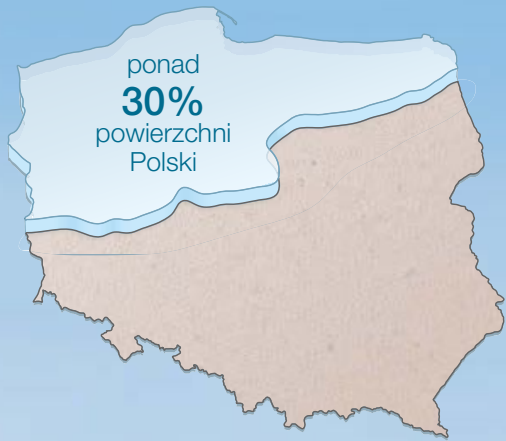
Zasięg zlodowaceń północnopolskich
