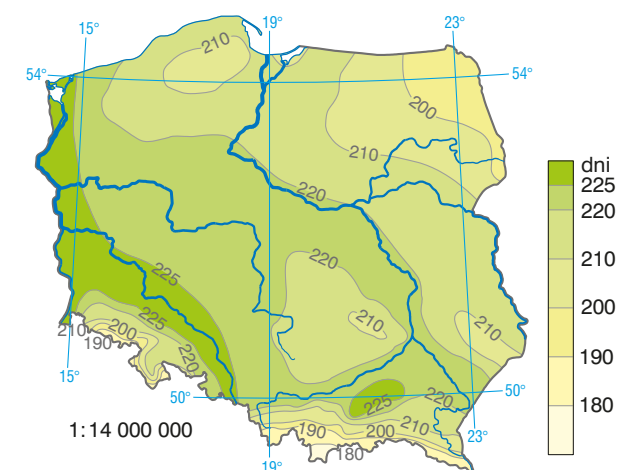
Długość okresu wegetacyjnego w Polsce.
