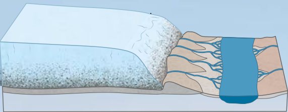
2 Obszar w trakcie zlodowacenia
