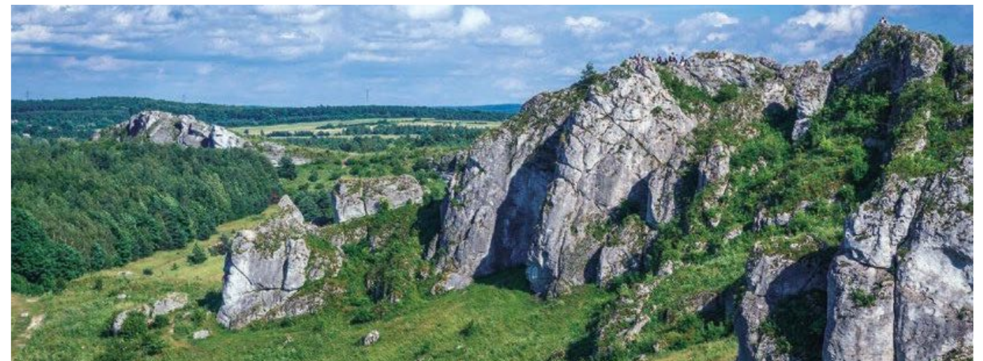
W jurze – jednym z okresów ery mezozoicznej – niemal cały obszar Polski był zalany przez morze. Ze szczątków żyjących w nim organizmów (z ich muszli i szkieletów) wytworzyły się pokłady wapieni jurajskich. Ich najokazalsze przykłady przetrwały na Wyżynie Krakowsko-Częstochowskiej, dlatego ten obszar bywa często nazywany Jurą.
