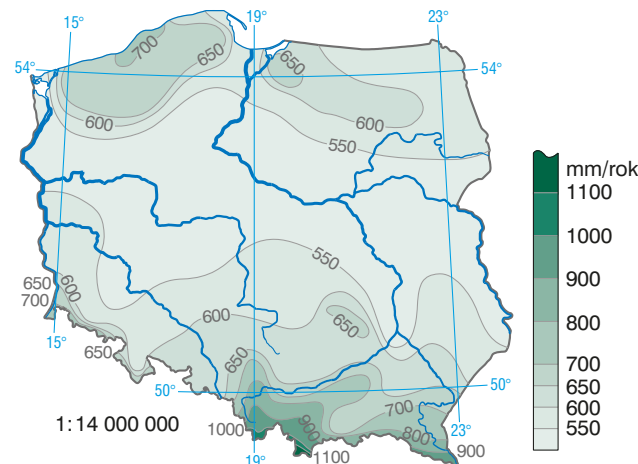
Roczne sumy opadów atmosferycznych.
