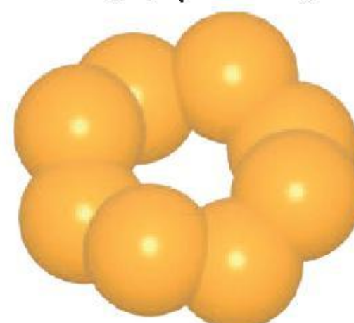
model cząsteczki siarki \text{S}_8
