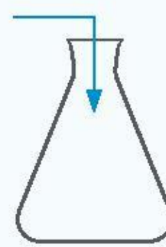
dodawanie substancji
