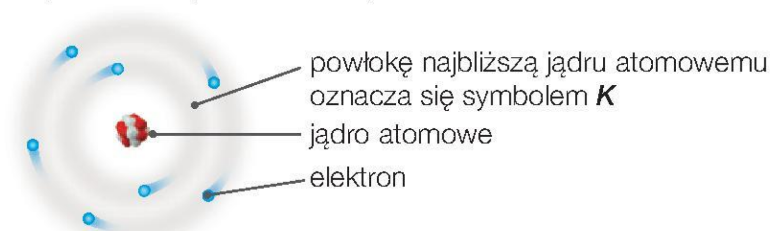
Rys. 13. Model atomu azotu.
