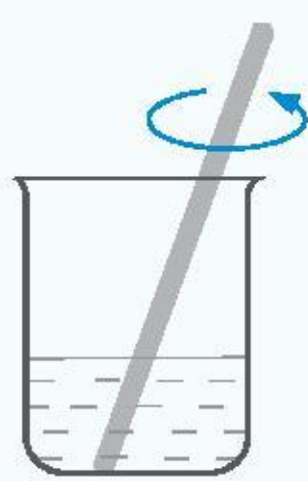
mieszanie
