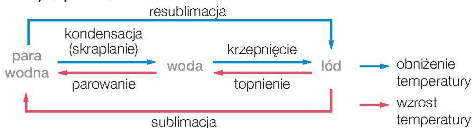
Rys. 22. Schemat zmian stanu skupienia wody.
