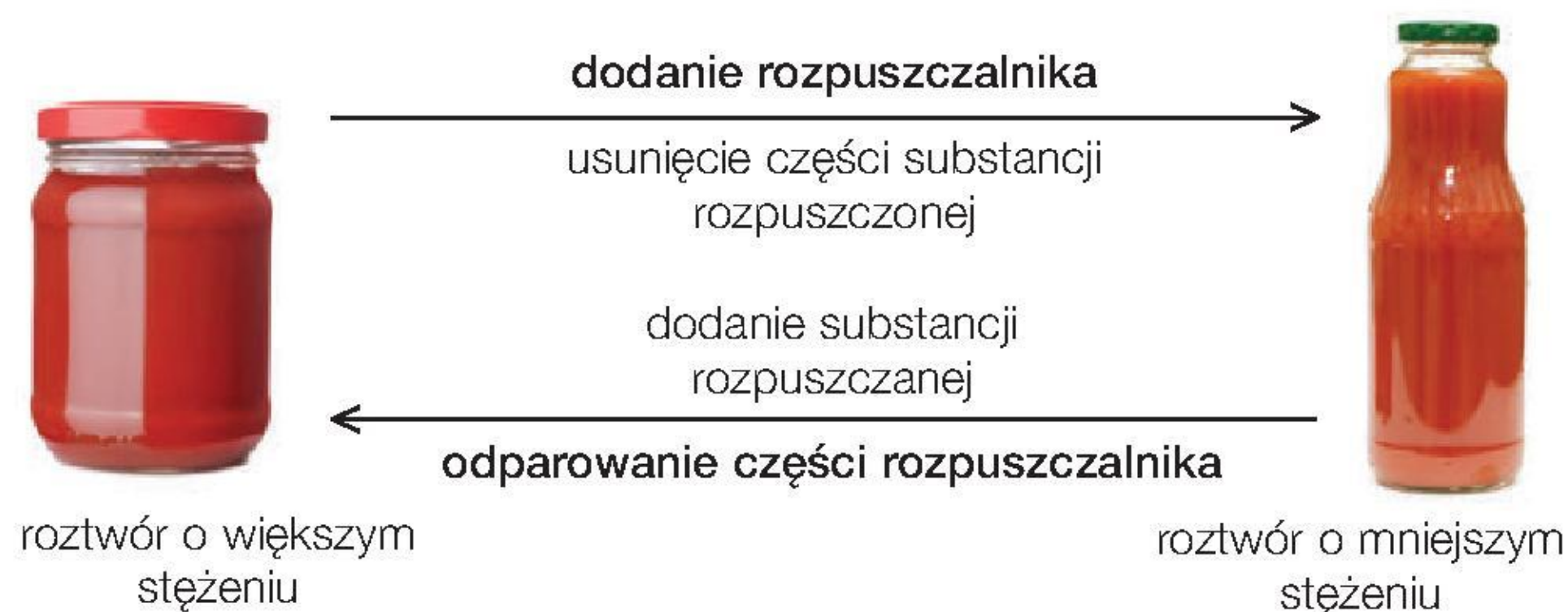
Fot. 121. Sposoby zmiany stężenia roztworu.
