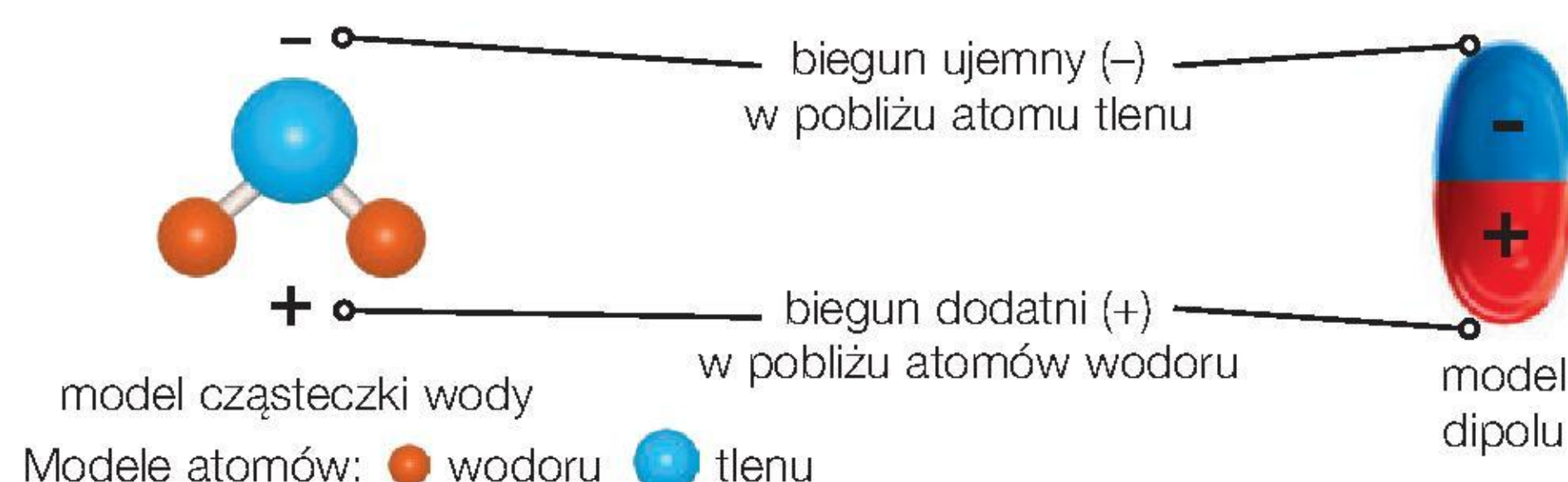
Rys. 23. Cząsteczka wody jest dipolem.
