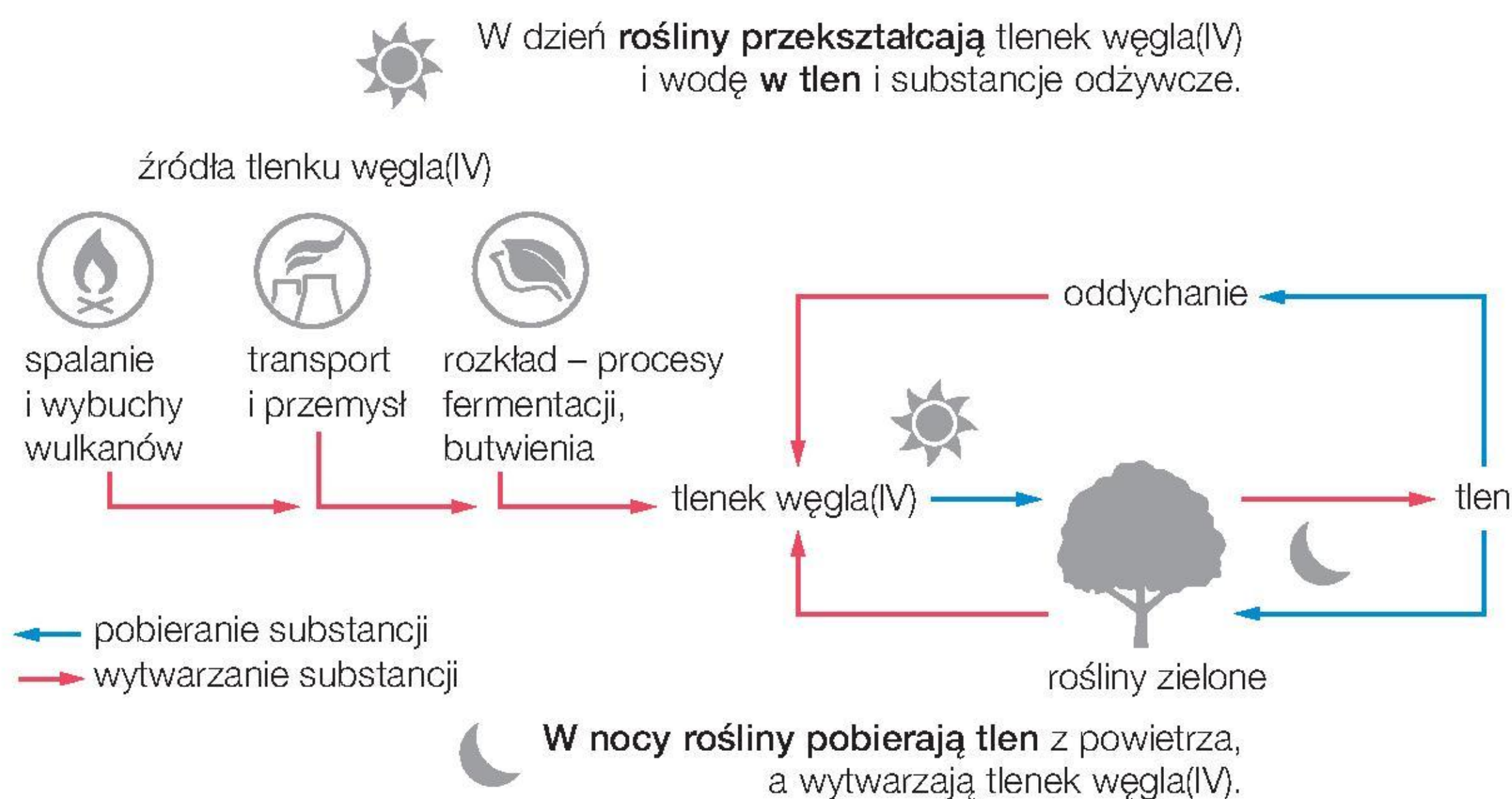
Rys. 9. Obieg tlenu i tlenku węgla(IV).
