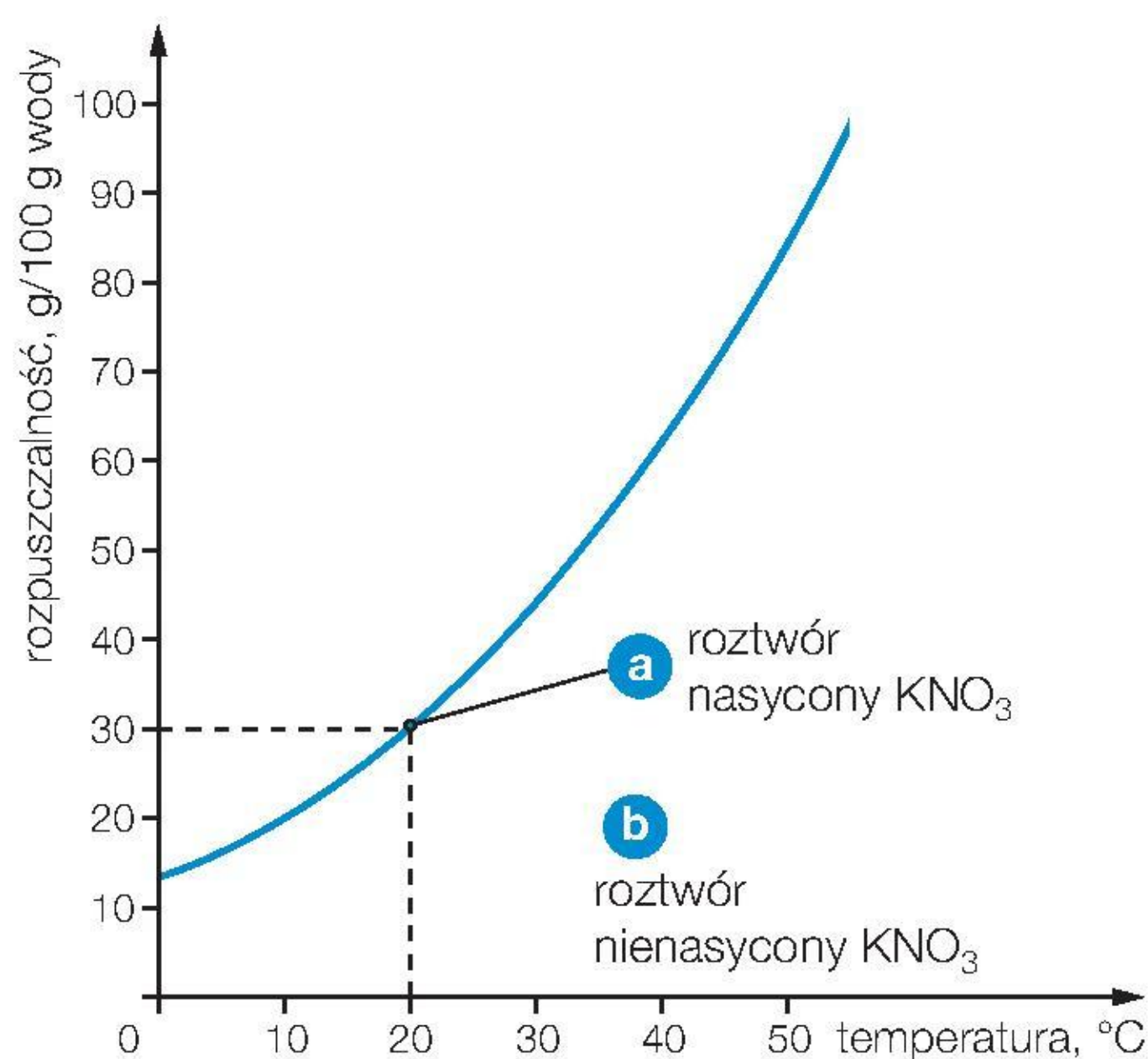
Rys. 27. Krzywa rozpuszczalności azotanu(V) potasu \text{KNO}_3 .
