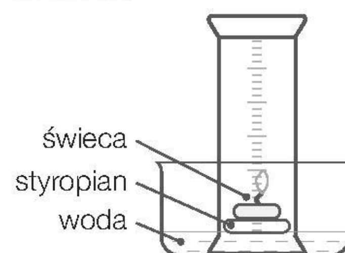
Schemat
