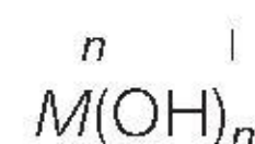
odczyn obojętny
