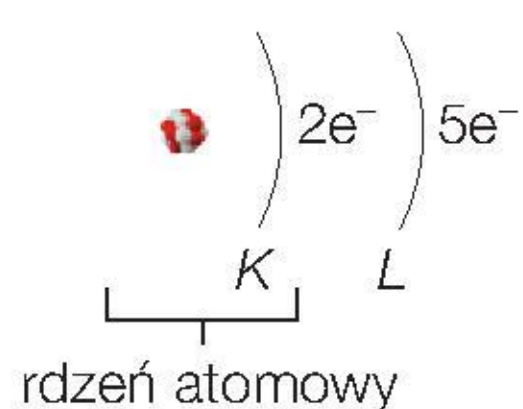
Rys. 15. Uproszczony model atomu azotu.
