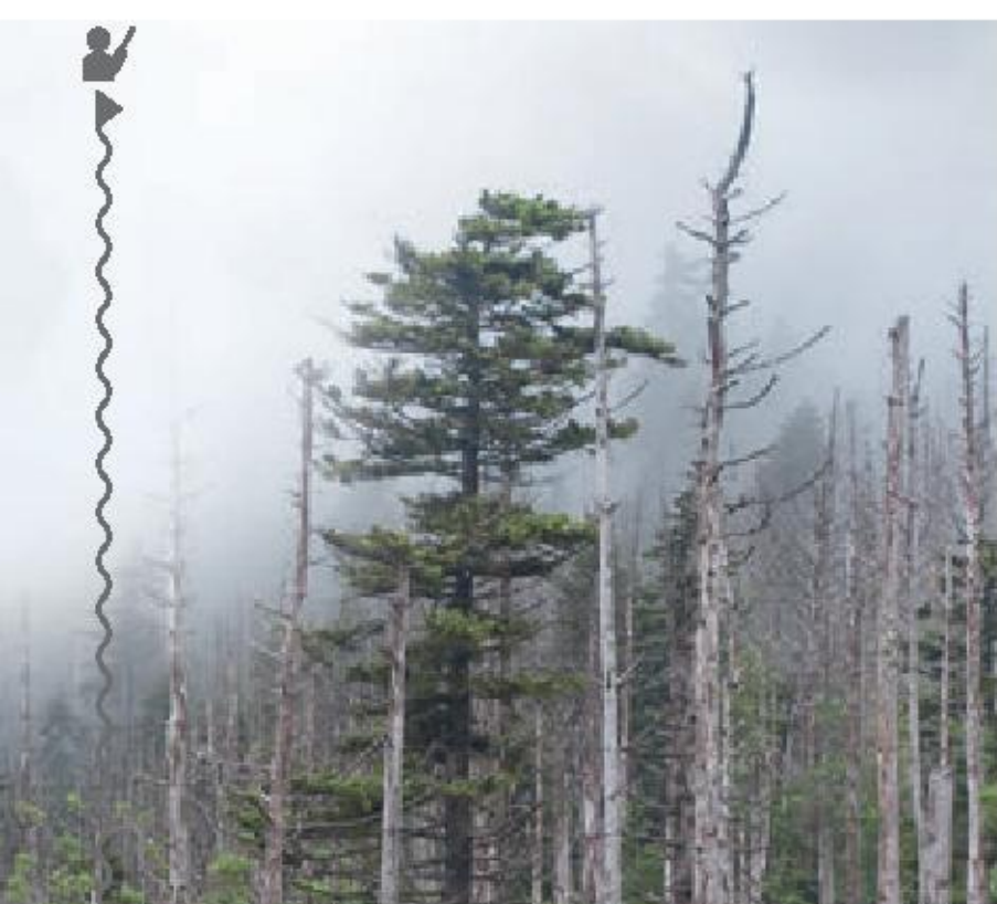
Fot. 59. Kwaśne opady niszczą tkanki roślin.
