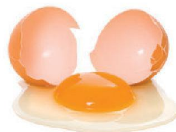
Fot. 79. Głównym składnikiem skorupy jaj jest związek jonowy – węglan wapnia.
