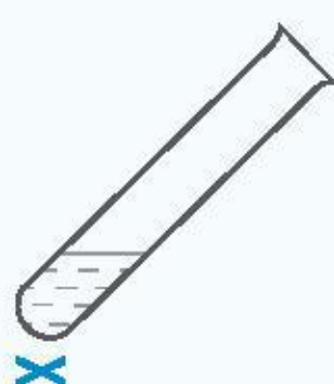
ogrzewanie
