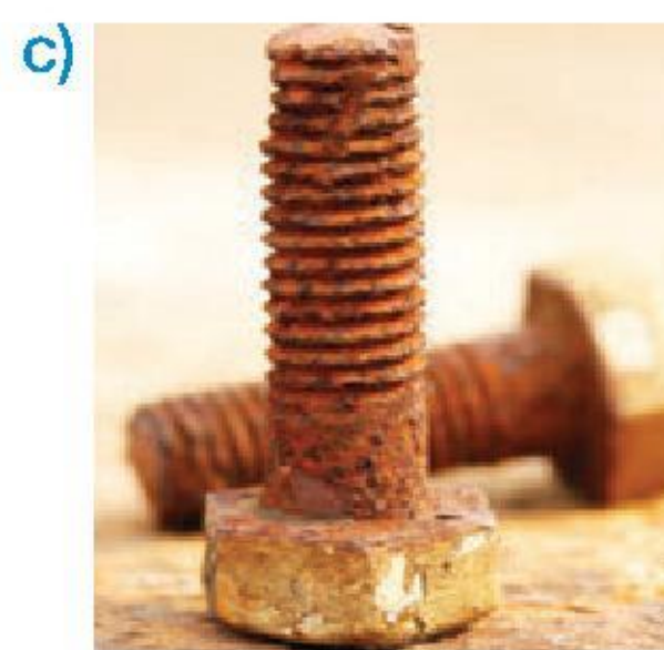
rdzewienie żelaza
