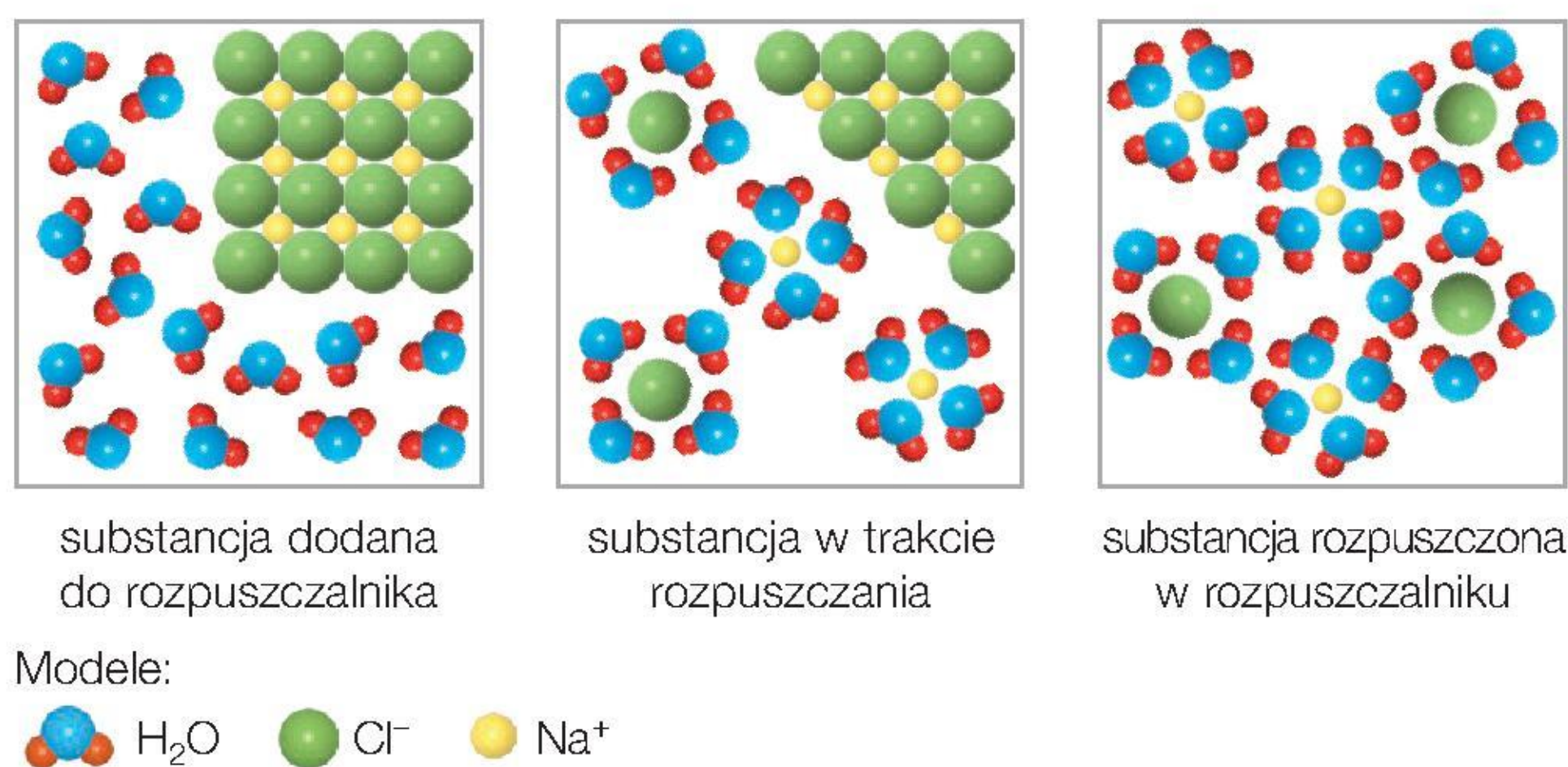
Rys. 26. Schemat rozpuszczania chlorku sodu w wodzie – polarne cząsteczki wody ustawiają się tak, aby biegun dodatni był jak najbliżej jonu Cl - , a biegun ujemny – jonu Na + .
