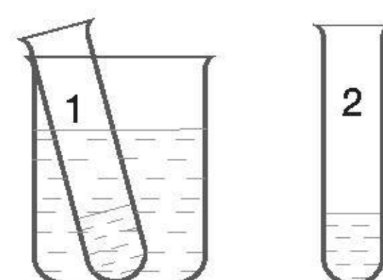
Schemat
