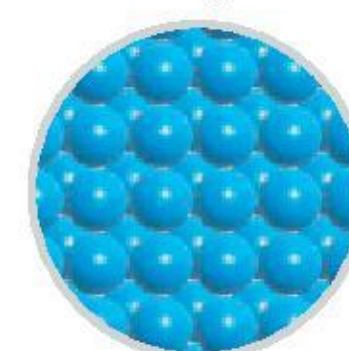
substancja stała
