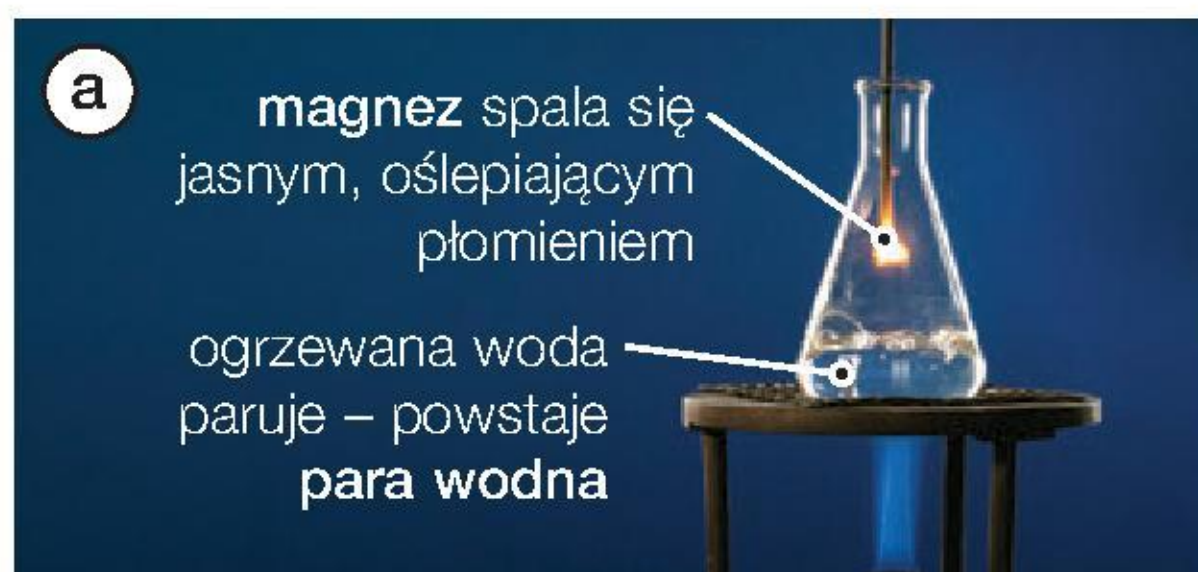
Fot. 57. Otrzymywanie wodoru w reakcji magnezu z parą wodną.
