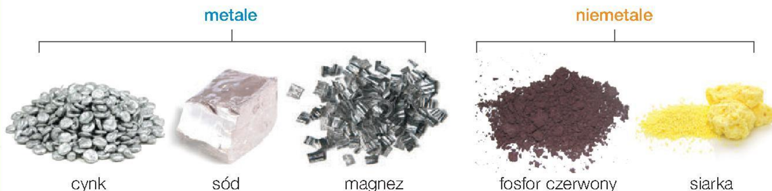
Fot. 28. Wybrane metale i niemetały.
