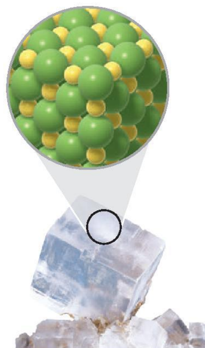
Fot. 78. Kryształ chlorku sodu.
