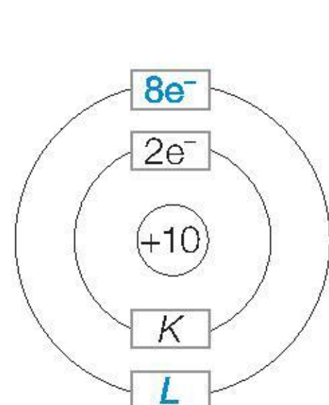
Rys. 18. Model atomu neonu.
