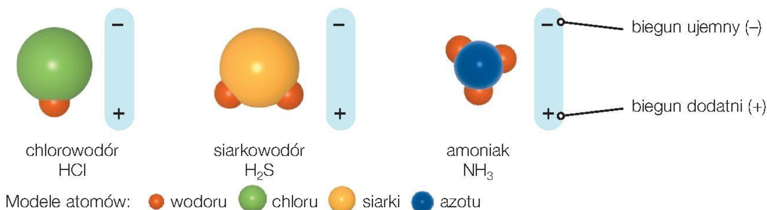
Rys. 25. Chlorowodór, siarkowodór i amoniak są dipolami.
