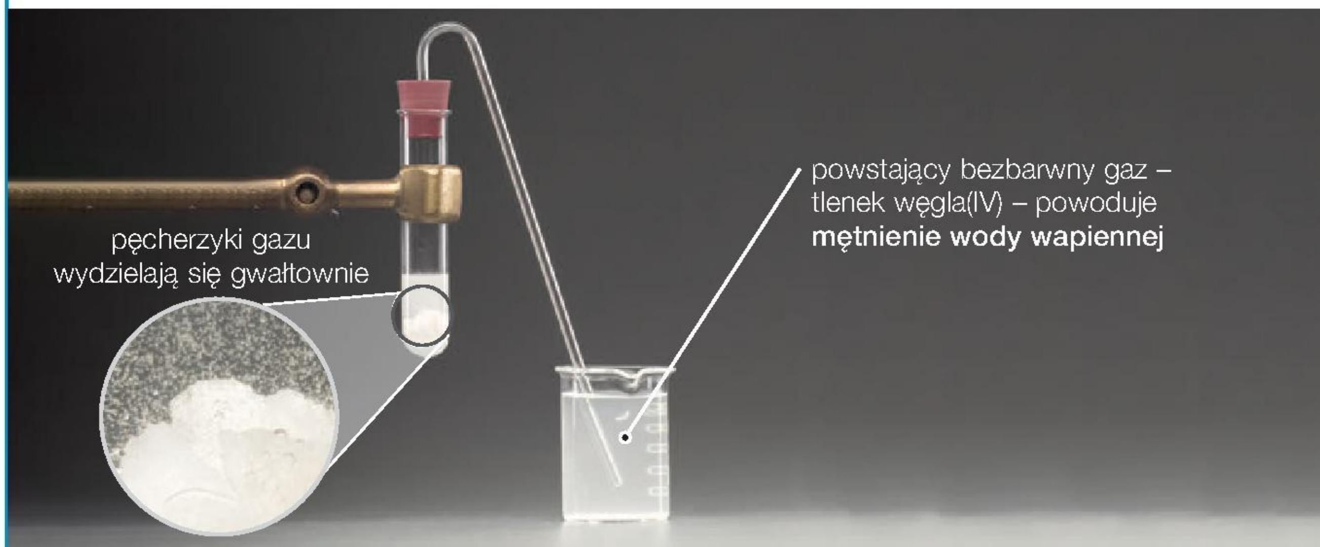
Fot. 50. Reakcja otrzymywania tlenku węgla(IV) przebiega gwałtownie.
