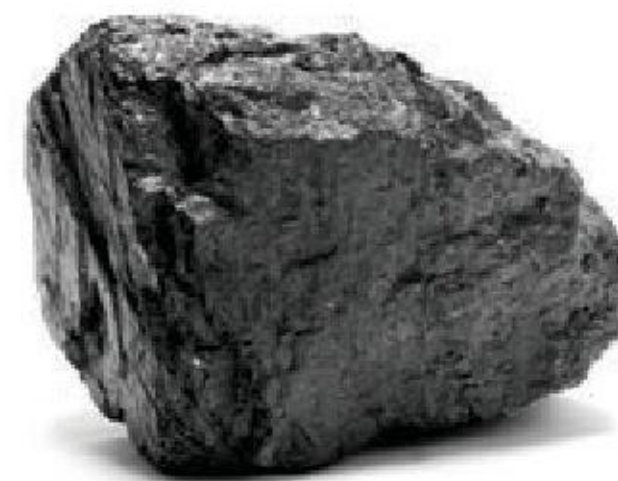
Fot. 23. Węgiel kamienny może zawierać do 92% czystego pierwiastka chemicznego.
