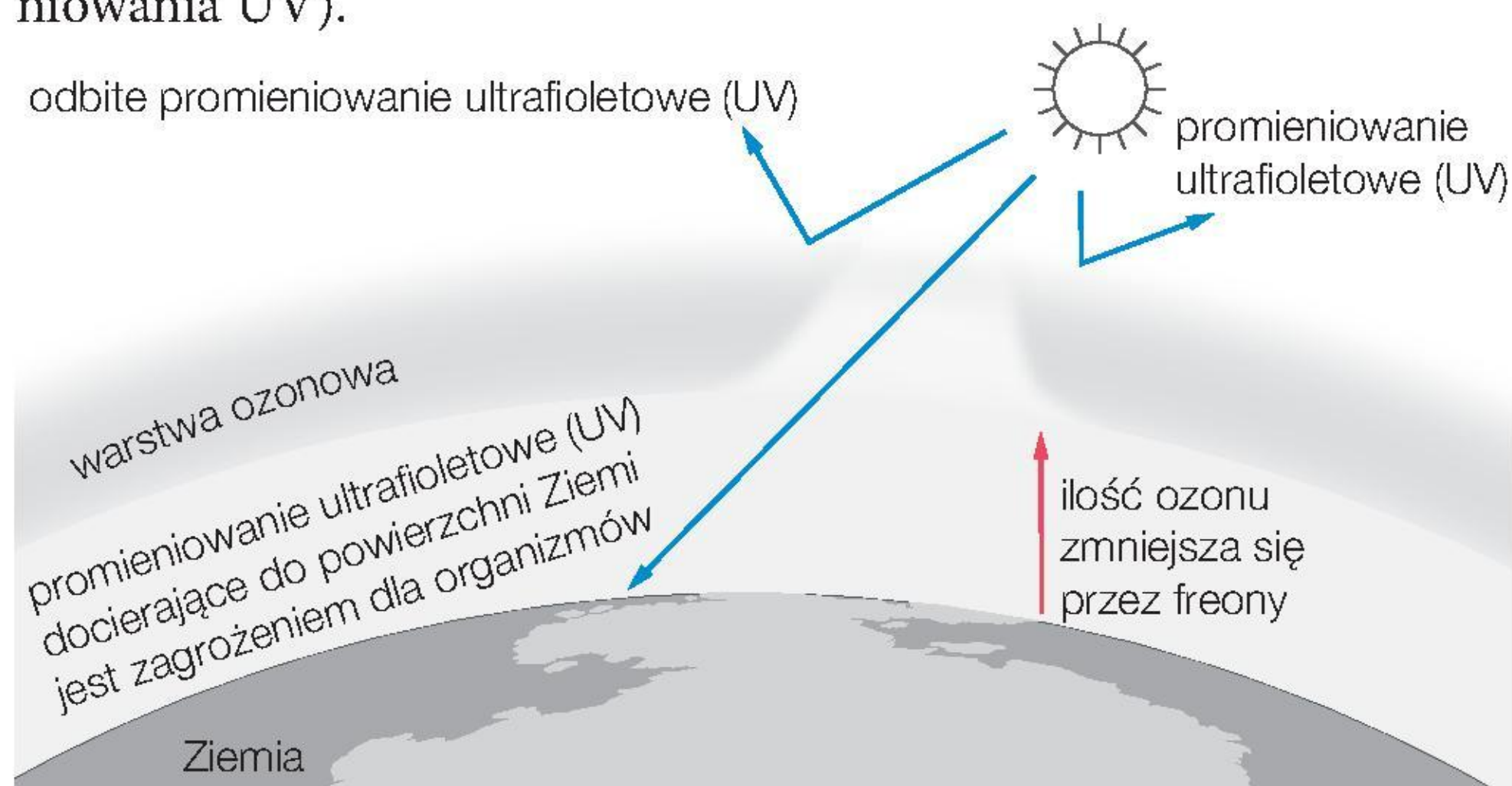
Rys. 10. Schemat powstawania dziury ozonowej.
