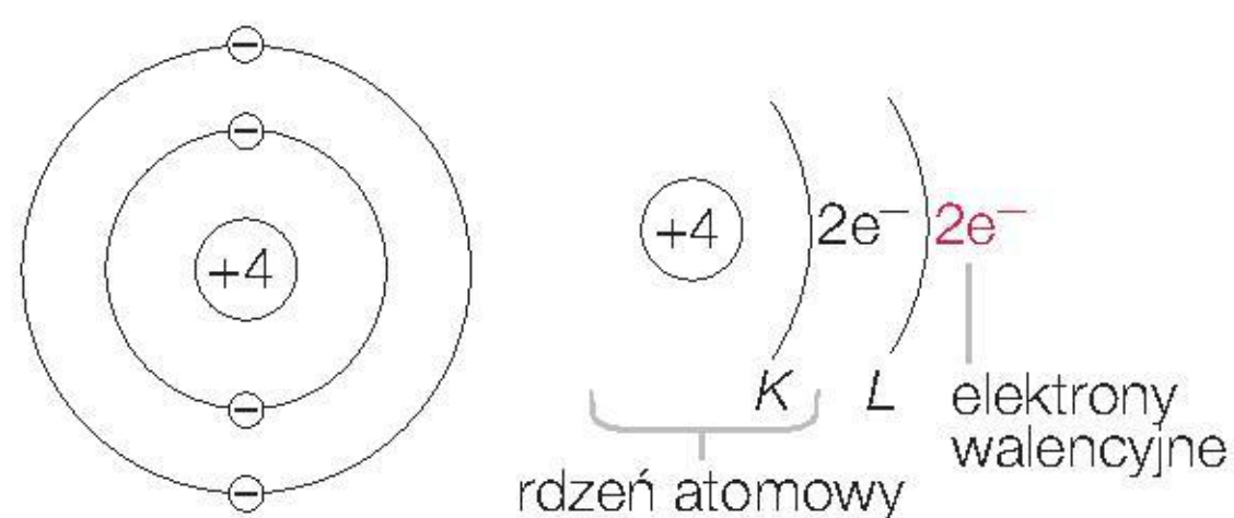
uproszczone modele atomu berylu
