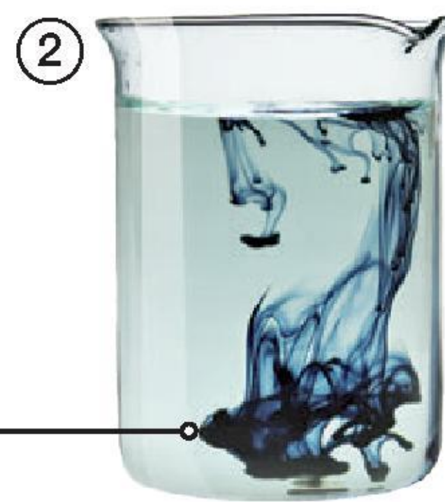
Fot. 64. Zjawisko dyfuzji – kryształy manganianu(VII) potasu (zlewka ①) i atrament (zlewka ②) wnikają między cząstki wody.
