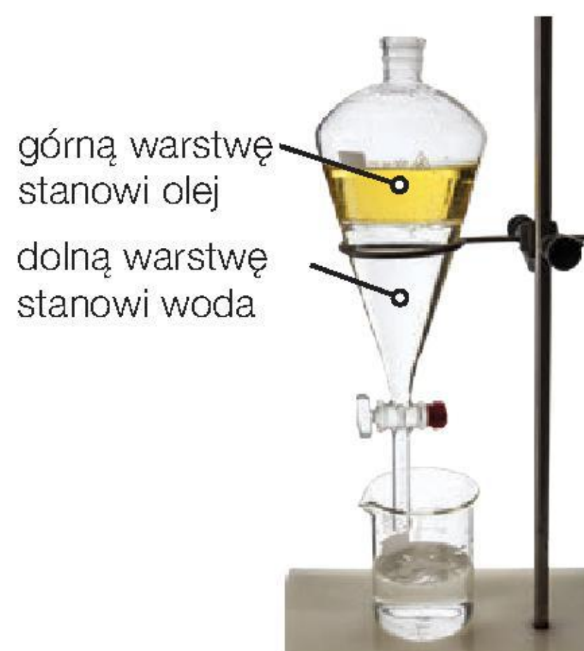
Fot. 18. Rozdzielanie za pomocą rozdzielacza.
