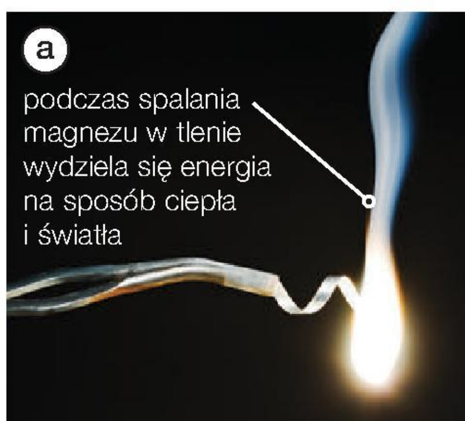
Fot. 61. Przykłady reakcji egzoenergetycznej (a) i endoenergetycznej (b).
