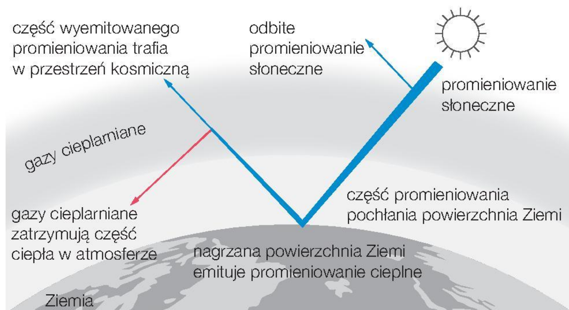
Rys. 12. Schemat powstawania efektu cieplarnianego.
