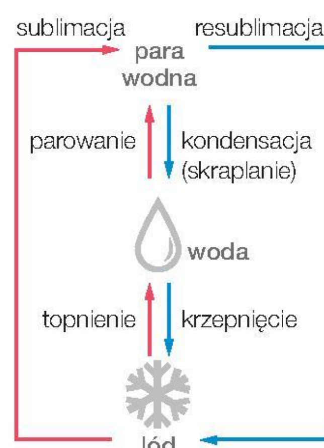
Rys. 8. Obieg wody w przyrodzie.
