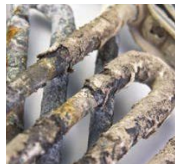
Fot. 62. Kamień kotłowy na grzałce.
