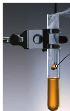
Fot. 48. Otrzymywanie kwasu fosforowego(V).
