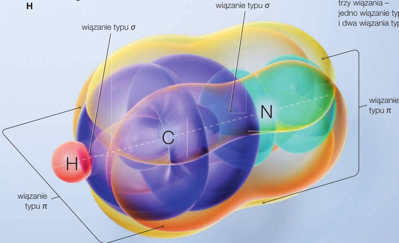
Model budowy cząsteczki HCN
