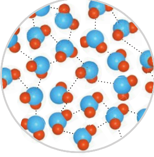
Rys. 38. Lód ma luźną strukturę, ponieważ jego wiązania wodorowe są dłuższe od tych występujących w wodzie w postaci ciekłej.
