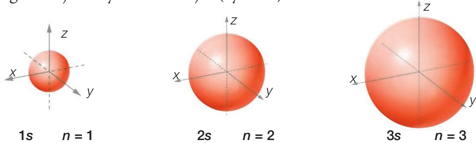
Rys. 15. Orbitale s mają kształt kuli, a ich promień są tym większe, im większa jest wartość n .
