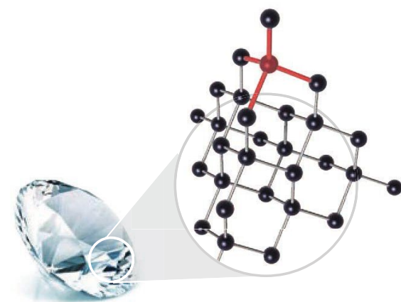
Fot. 19. W diamentie każdy atom węgla jest połączony wiązaniami kowalencyjnymi z czterema innymi atomami węgla.
