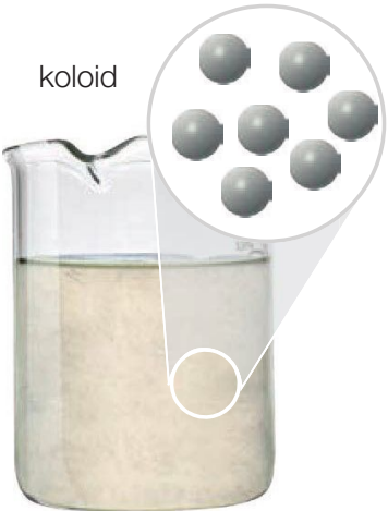
Fot. 77. Roztwory właściwe i koloidy różnią się wielkością cząstek substancji rozpuszczonej.
