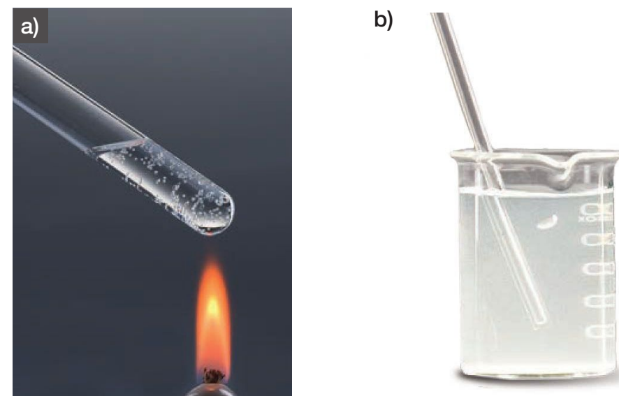
Fot. 84. W podwyższonej temperaturze z wody mineralnej wydziela się gaz – \text{CO}_2 – a). Można go zidentyfikować za pomocą wody wapiennej, która pod jego wpływem mętnieje – b).
