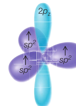
Rys. 47. W wyniku wymieszania 1 orbitalu s i 2 orbitali p powstają 3 orbitale zhybrydyzowane sp^2 .
