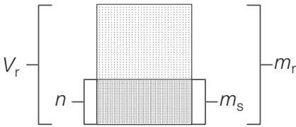
Rys. 74. Zależność między wielkościami opisującymi stężenia.
