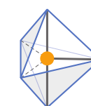
hybrydyzacja sp^3d – kształt bipyramidy trygonalnej
