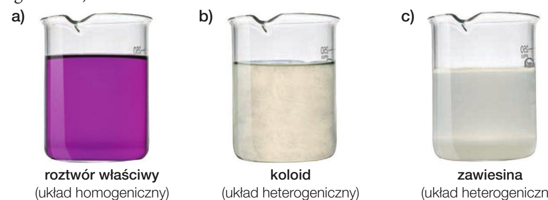
Fot. 74. Manganian(VII) potasu z wodą – a), białko jaja kurzego z wodą – b), mąka z wodą – c).
