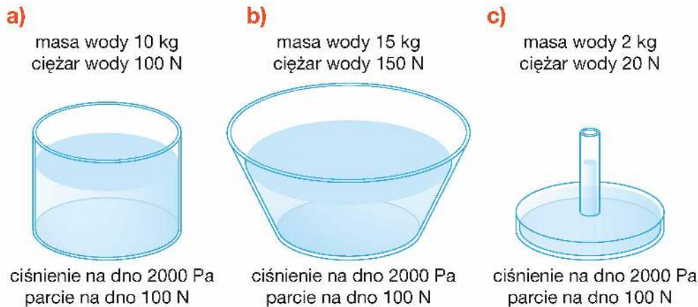
Rys. 7.16. Parcie na dno naczynia nie musi być równe ciężarowi cieczy
