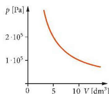
Rys. 8.10. Wykresy: a) przemiany izotermicznego sprężania gazu od objętości 10 \text{ dm}^3 do 5 \text{ dm}^3 , b) zależności p(V) w przemianie izotermicznej
