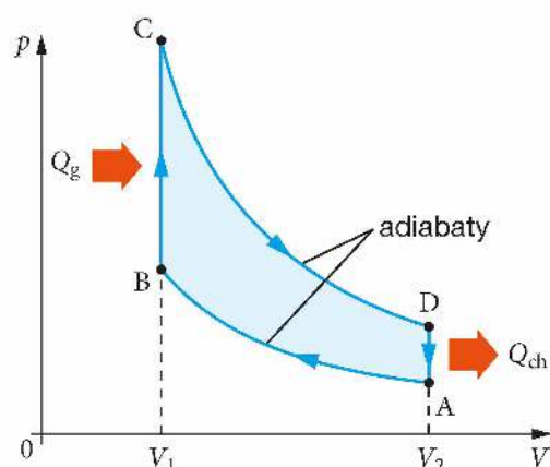
Rys. 8.32. Wykres cyklu Otta w układzie ( V, p )
