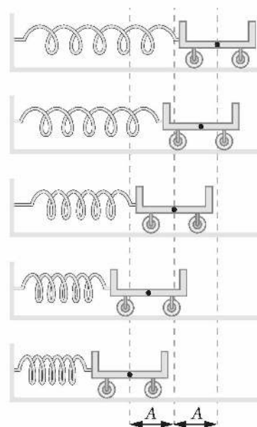
Rys. 9.31. Podczas ruchu w poziomie wagonika na sprężynie zachodzi przemiana energii kinetycznej w energię potencjalną sprężystości i z powrotem
