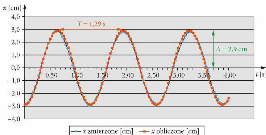
Rys. 9.20. Wykresy zależności wychylenia wahadła od czasu x(t) sporządzone na podstawie danych doświadczalnych (wykres niebieski) oraz wzoru opisującego ruch harmoniczny (wykres czerwony)
