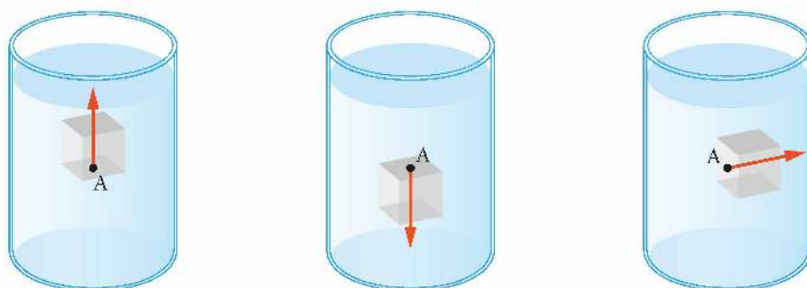
Rys. 7.6. Znajomość ciśnienia w punkcie A pozwala obliczyć wartość siły, jaka zadziała na ściankę umieszczonego w tym punkcie ciała o określonej wielkości, ale kierunek i zwrot tej siły zależą od tego, jak umieścimy ciało
