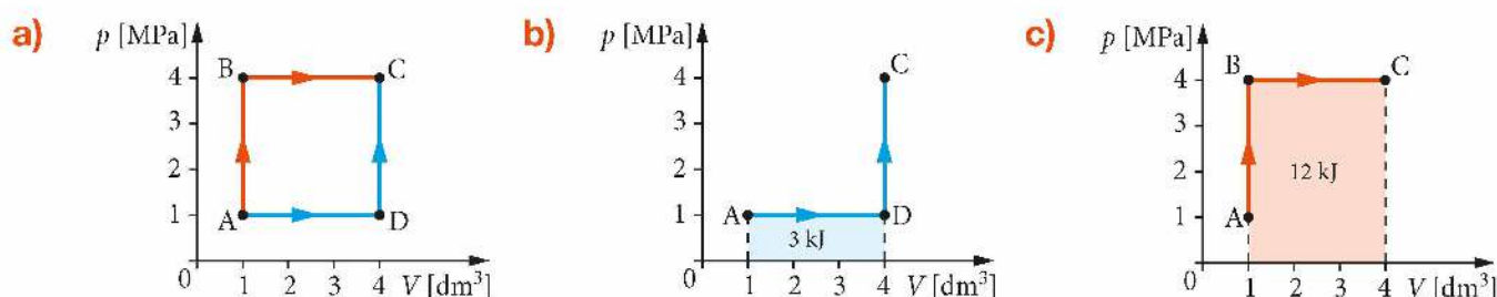
Rys. 8.21. a) porównanie dwóch przemian od stanu A do stanu C, b) obliczanie pracy w przemianie A–D–C, c) obliczanie pracy w przemianie A–B–C
