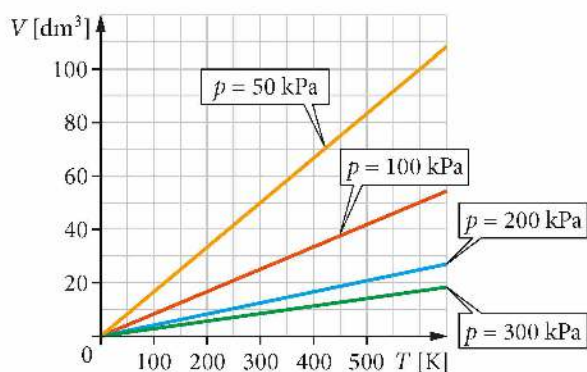
Rys. 8.4. Izobary – wykresy przedstawiające zależność objętości 1 mola gazu od temperatury w przemianie izobarycznej. Każdy z wykresów dotyczy innego ciśnienia
