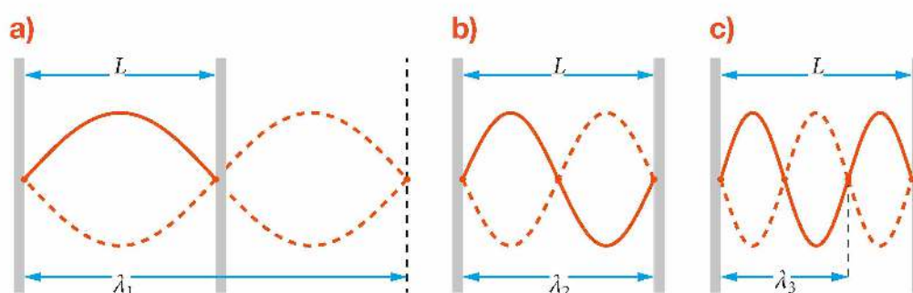
Rys. 10.49. Strunę można pobudzić do drgań tak, że: a) będzie miała węzły tylko na końcach – wtedy \lambda_1 = 2L , b) i c) powstaną kolejne składowe harmoniczne i fala będzie miała węzły nie tylko na końcach struny – wtedy \lambda_n = \frac{\lambda_1}{n}
