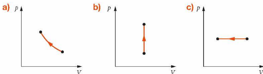
Rys. 8.11. Wykresy: a) izotermicznego sprężania, b) izochorycznego ogrzewania, c) izobarycznego chłodzenia
