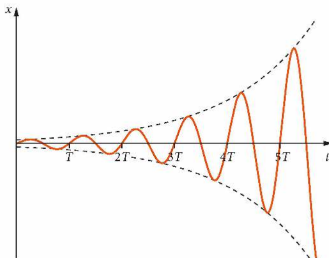
Rys. 9.38. W przypadku rezonansu amplituda drgań rośnie. Przy braku tłumienia rosłaby coraz bardziej
