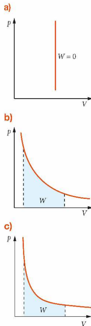
Rys. 8.20. Praca w przemianach gazowych: a) izochorycznej, b) izotermicznej, c) adiabatycznej
