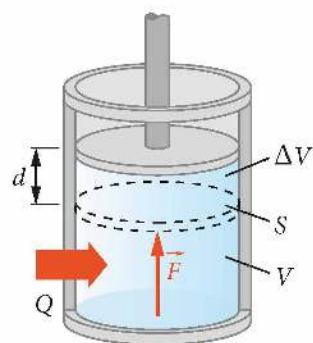
Rys. 8.18. Izobaryczne rozprężanie gazu, \Delta V = Sd
