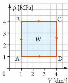
Rys. 8.23. Uzyskana praca jest równa polu wewnątrz figury
