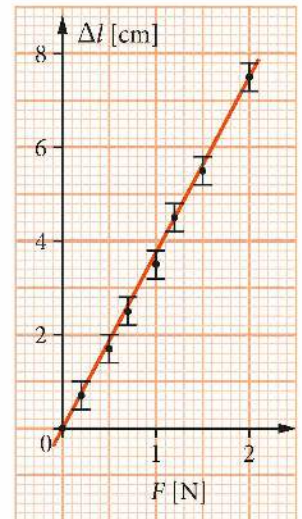
Rys. 9.21. Wykres zależności wydłużenia sprężyny od ciężaru obciążnika
