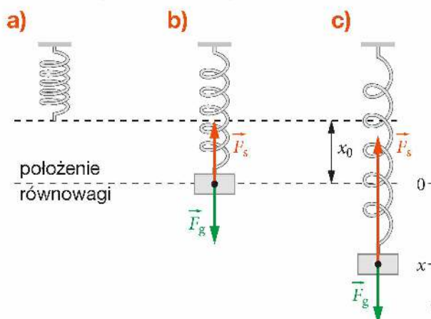
Rys. 9.19. Siły działające na ciało zawieszone na sprężynie
