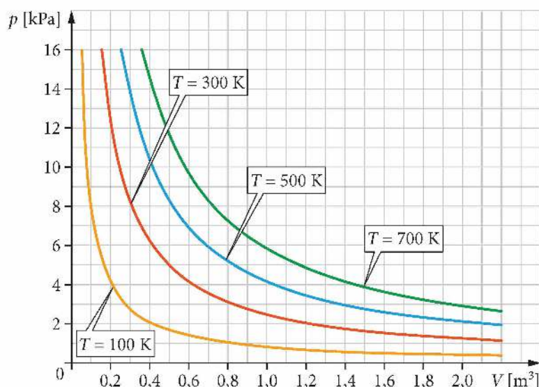
Rys. 8.3. Izotermy – wykresy przedstawiające zależność ciśnienia 1 mola gazu od objętości, do której został on sprężony, w przemianie izotermicznej. Każdy z wykresów odpowiada określonej temperaturze
