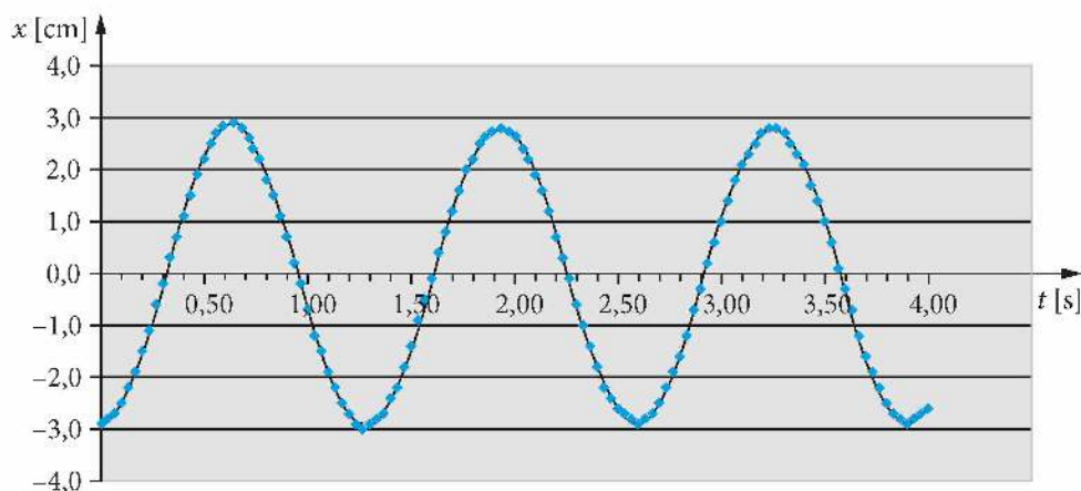
Rys. 9.3. Wykres zależności x(t) dla ciężarka na sprężynie – wyniki dośw. 18.
