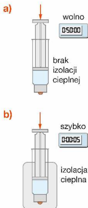
Rys. 8.14. Sprężanie gazu: a) izotermiczne, b) adiabatyczne
