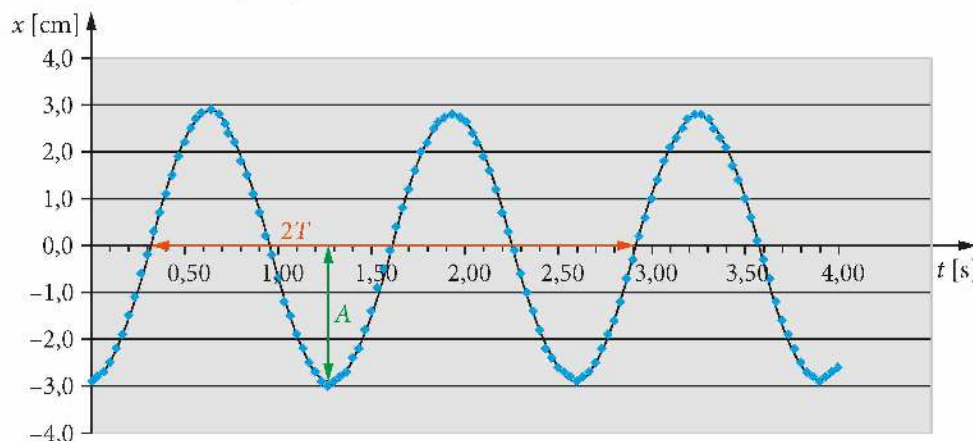
Rys. 9.4. Wykres drgań z zaznaczoną amplitudą i okresem drgań
