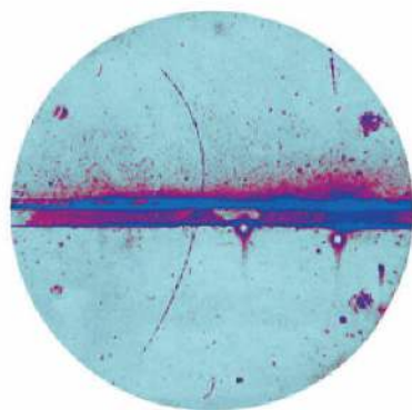
Rys. 7.53. Zdjęcie z komory mgłowej z 1932 r. – pierwszy dowód istnienia antymaterii
