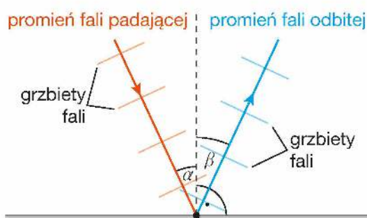
Rys. 10.28. Kąt odbicia \beta jest równy kątowi padania \alpha
