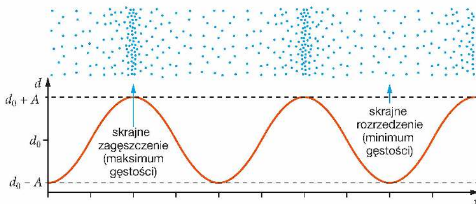
Rys. 10.20. Wykres zmian gęstości powietrza w zależności od odległości od źródła dźwięku dla czystego tonu w pewnej chwili. W miarę upływu czasu zagęszczenia i rozrzedzenia się przesuwają – fala się przemieszcza. W rzeczywistości zagęszczenia i rozrzedzenia cząsteczek są wielokrotnie mniejsze niż na naszych poglądowych rysunkach
