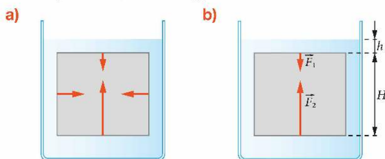
Rys. 7.28. Pochodzenie siły wyporu działającej na ciało całkowicie zanurzone w cieczy
