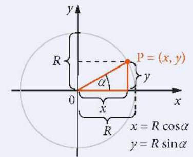
Rys. 9.6. Współrzędne punktu P , znajdującego się na okręgu o promieniu R , zależą od kąta \alpha
