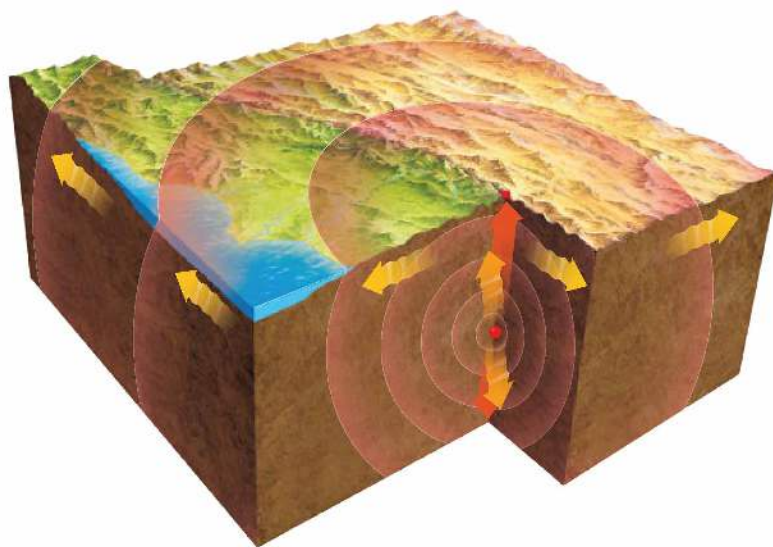
Rys. 10.11. Podłużna fala sejsmiczna porusza się z prędkością 4\text{--}8 \frac{\text{km}}{\text{s}} , a poprzeczna z prędkością 2\text{--}5 \frac{\text{km}}{\text{s}}
