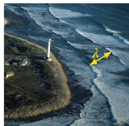
Rys. 10.12. Fale na morzu – zaznaczona długość fali
