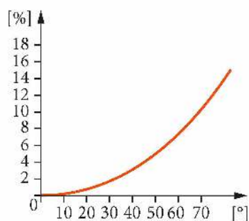
Rys. 9.30. Różnica (w procentach) między rzeczywistym okresem drgań wahadła a obliczonym ze wzoru (patrz opis w tekście)
