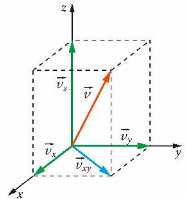
Rys. 8.8. Rozkład wektora prędkości na składowe v^2 = v_x^2 + v_y^2 + v_z^2 , v_{xy}^2 = v_x^2 + v_y^2
