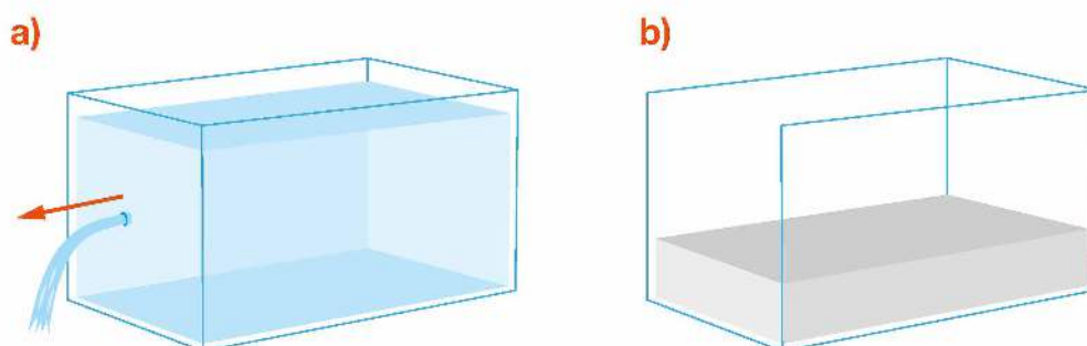
Rys. 7.3. a) woda naciska na ścianki, a te powstrzymują wodę przed wylaniem się z naczynia, b) ciało stałe nie oddziałuje ze ściankami – po usunięciu jednej ściany pozostaje na swoim miejscu
