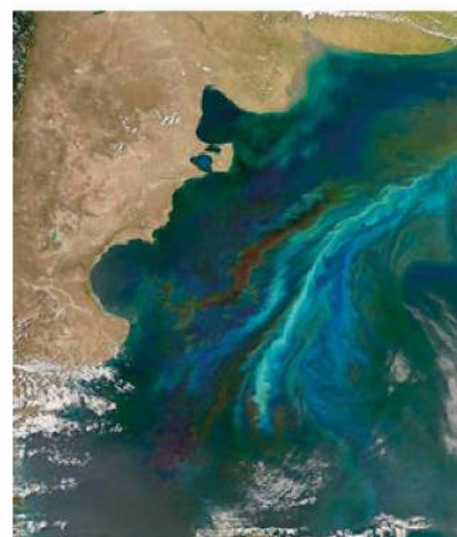
Rys. 7.60. Prądy morskie mają duży wpływ na klimat w wielu regionach Ziemi. Na zdjęciu prąd morski widoczny z satelity dzięki obecności fitoplanktonu
