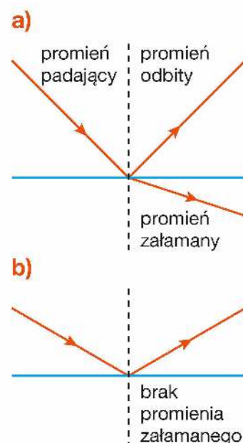
Rys. 10.33. Odbicie i załamanie fali (a) oraz jej całkowite odbicie dla dużego kąta padania (b)
