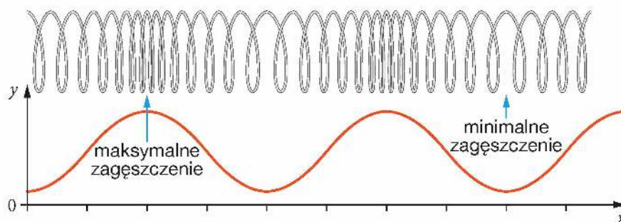
Rys. 10.16. Wykres fali podłużnej przedstawia zależność liczby zwojów na jednostkę długości ( y ) od współrzędnej ( x ) mierzonej zgodnie z kierunkiem osi, wzdłuż której rozchodzi się fala. Nie jest to obraz falującej sprężyny
