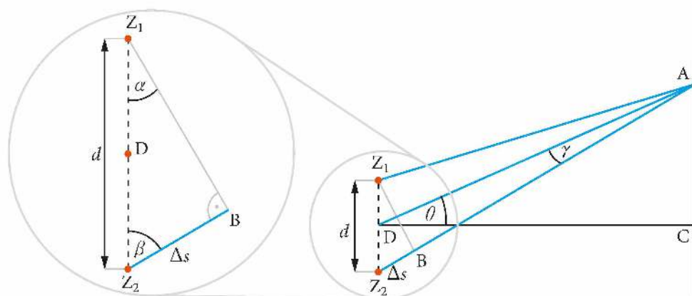
Rys. 10.40. Schemat ilustrujący wyprowadzenie wzoru na warunek wzmocnienia fali
