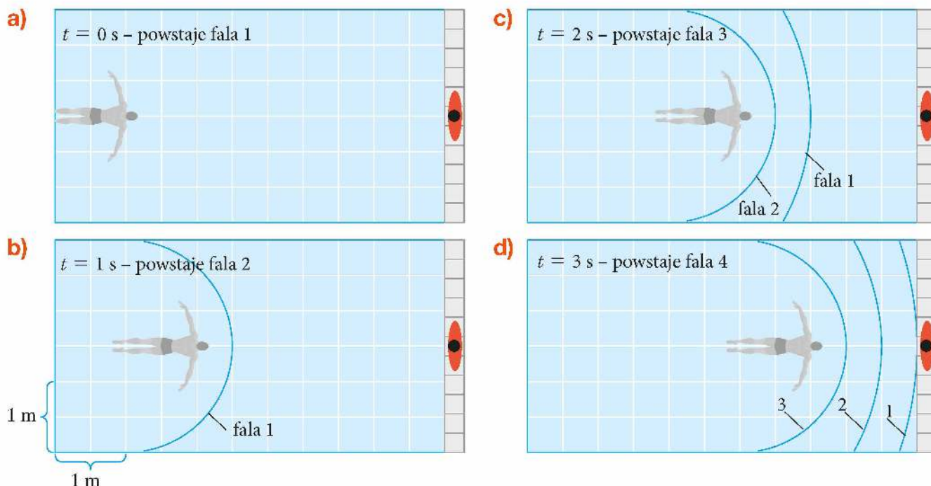
Rys. 10.55. Pływak i efekt Dopplera – źródło fali zbliża się do nieruchomego obserwatora. Dla uproszczenia zaznaczyliśmy falę tak, jakby rozchodziła się od głowy pływaka
