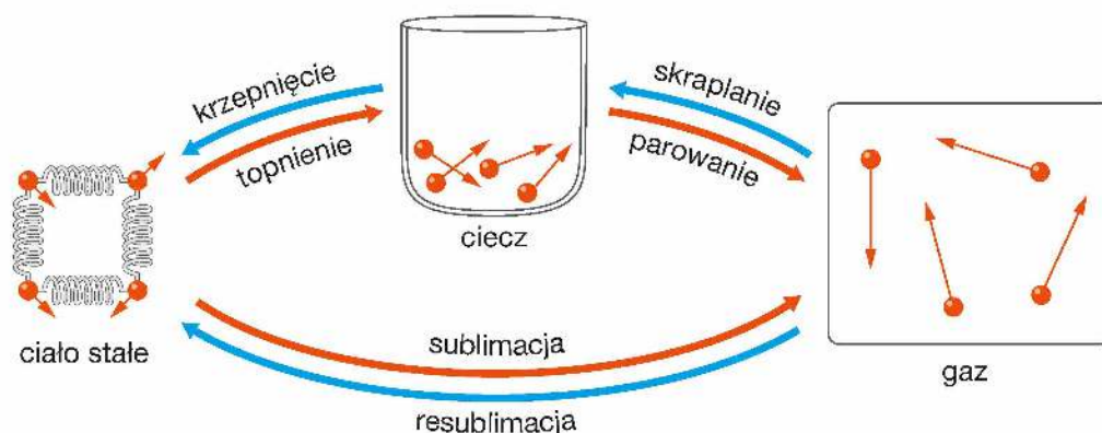
Rys. 7.47. Zmiany stanów skupienia (przemiany fazowe)
