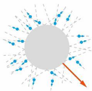
Rys. 7.39. Model zderzeń cząsteczek wody z ziarenkiem pyłku rośliny
