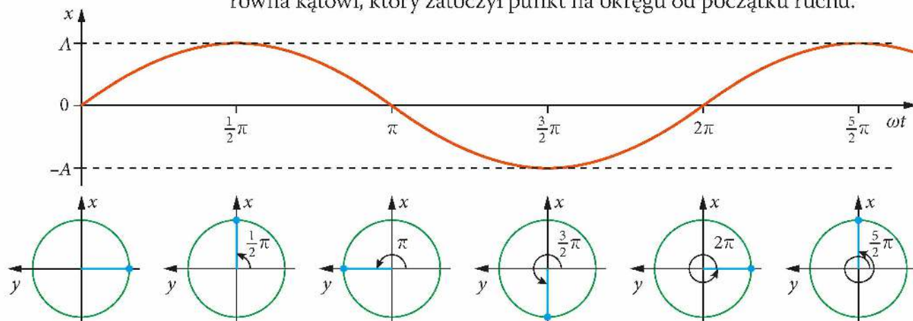
Rys. 9.14. Ruch punktu po okręgu a zmiany położenia jego rzutu. Układ współrzędnych, w którym narysowaliśmy okrąg, został obrócony tak, aby oś x była ustawiona pionowo, jak na wykresie powyżej
