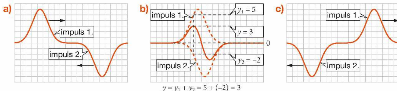
Rys. 10.35. Widok od góry impulsów rozchodzących się na sznurze a) przed spotkaniem, b) podczas ich spotkania, gdy obserwujemy superpozycję, c) po spotkaniu
