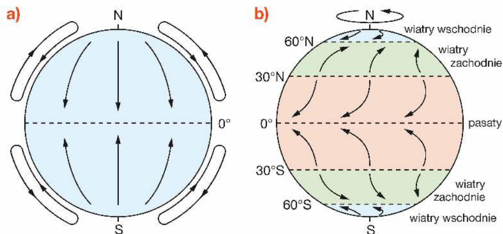
Rys. 7.61. Obieg powietrza wynikający z konwekcji, a) gdyby Ziemia się nie obracała, b) na obracającej się Ziemi
