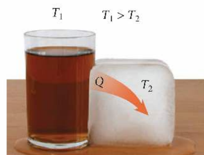
Rys. 7.41. Napój i lód mają różne temperatury. Różnica temperatur powoduje przepływ ciepła Q od napoju do lodu
