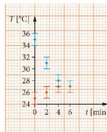
Rys. 7.42. Punkty pomiarowe wraz z niepewnością pomiaru T
