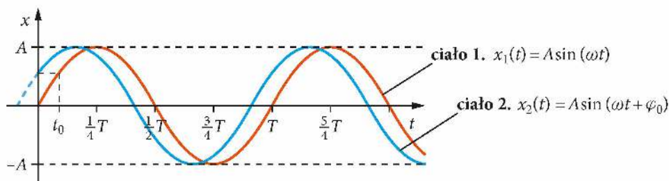
Rys. 9.16. Wykresy x(t) dla dwóch ciał poruszających się ruchem drgającym
