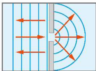
Rys. 10.43. Zachowanie się fali płaskiej padającej na przegrodę ze szczeliną w zależności od jej rozmiaru: a) gdy rozmiar szczeliny jest porównywalny z długością fali, fala ulega dyfrakcji – za otworem powstaje fala kolista, b) gdy rozmiar szczeliny jest dużo większy od długości fali, fala przechodzi na drugą stronę prawie niezaburzona
