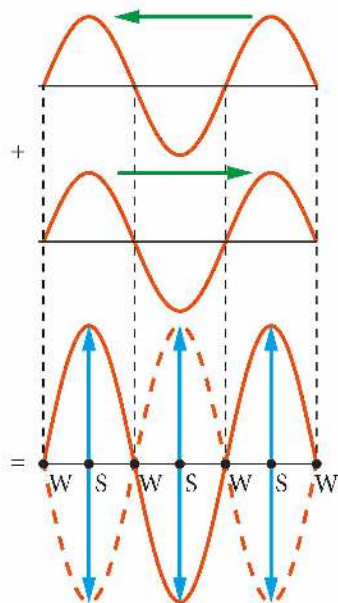
Rys. 10.47. Fala stojąca powstaje w wyniku nałożenia się dwóch fal biegnących w przeciwnie strony
