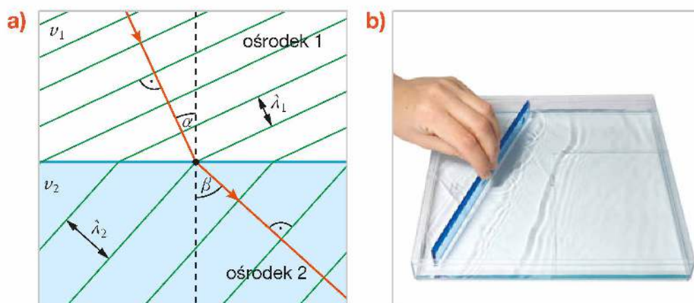
Rys. 10.29. a) Schematyczne przedstawienie przejścia fali z jednego ośrodka do drugiego, w którym fala rozchodzi się szybciej. Grzbiety fal tworzą ciągłe linie. b) Załamanie fali na granicy głębszej i płytszej wody (na dnie naczynia w prawym dolnym rogu ułożono prostokątną szklaną płytkę). Na wodzie o innej głębokości fala rozchodzi się z inną prędkością
