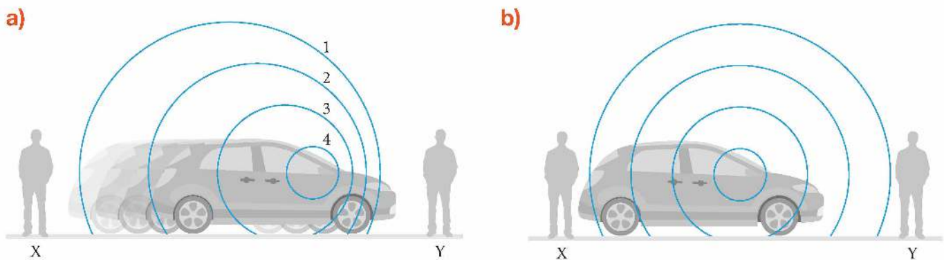
Rys. 10.56. Gdy źródło zbliża się do obserwatora, następuje przesunięcie w stronę częstotliwości wyższych, a gdy oddala się od niego – w stronę częstotliwości niższych (a). Jeśli źródło dźwięku jest względem obserwatora nieruchome, wtedy nie nastąpi przesunięcie w odbieranej częstotliwości fali (b)
