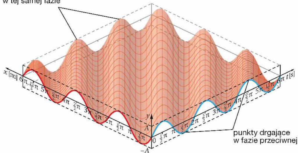
Rys. 10.15. Punkty drgające w zgodnej lub przeciwnej fazie na wykresie funkcji falowej
