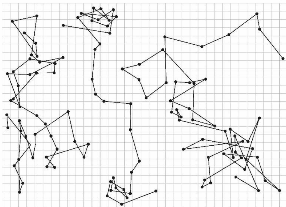
Rys. 7.38. Położenia cząstki pyłku w wodzie mierzone w równych odstępach czasu. Linia łącząca kolejne punkty nie jest torem ruchu pyłku, ułatwia jedynie odnalezienie jego kolejnego położenia. Zderzenia z cząsteczkami następują tak szybko, a przebyta między nimi droga jest tak mała, że rzeczywisty rysunek toru ruchu pyłku wyglądałby nie jak linia łamana, ale jak krzywa
