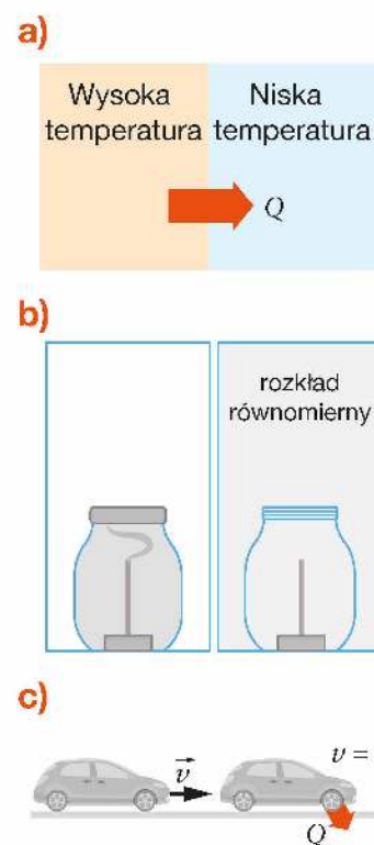
Rys. 8.35. Przykłady procesów nieodwracalnych: a) przepływ ciepła, b) rozprzestrzenianie się dymu po otwarciu słoika, c) zamiana energii mechanicznej w wewnętrzną (pracy w ciepło)
