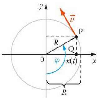
Rys. 9.10. Punkt Q porusza się po osi x ruchem drgającym opisanym wzorem x(t) = R \sin \varphi(t) , gdzie R – promień okręgu
