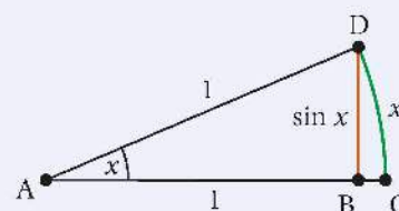
Rys. 9.28. Porównanie kąta i jego sinus
