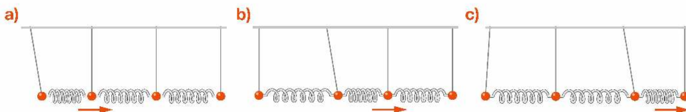
Rys. 10.6. Mechanizm powstawania fali podłużnej – kolejne etapy przemieszczania się impulsu falowego
