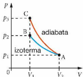
Rys. 8.15. Wykresy zależności p(V) dla przemian: izotermicznej (niebieski) i adiabatycznej (czerwony)
