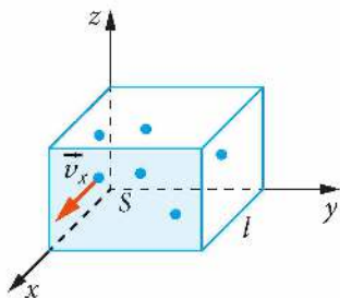
Rys. 8.7. Gaz w zamkniętym naczyniu
