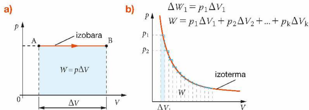
Rys. 8.19. Wykresy zależności p(V) a) dla przemiany izobarycznej, b) dla przemiany izotermicznej (można przybliżyć wykresem słupkowym)
