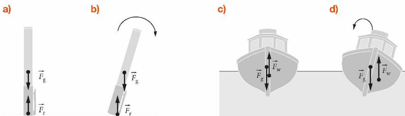
Rys. 7.33. W odróżnieniu od flamastra łódź nie wywraca się przy niewielkich wychyleniach, gdyż środek wyporu zmienia swoje położenie
