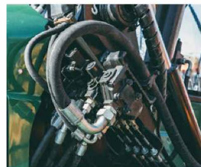
Rys. 7.10. Przewody systemu hydraulicznego w maszynie rolniczej
