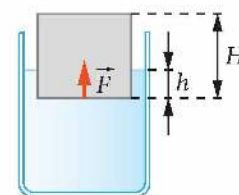
Rys. 7.29. W przypadku ciała pływającego po powierzchni cieczy siła wyporu to po prostu siła parcia na dolną powierzchnię ciała
