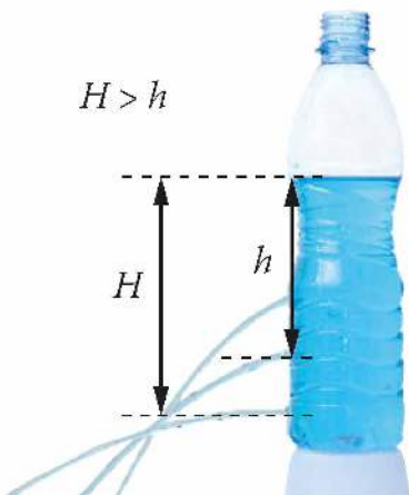
Rys. 7.15. Słupy cieczy nad środkowym i nad najniższym otworem
