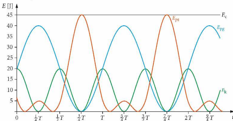
Rys. 9.36. Wykres przemian energii obciążnika zawieszonego na sprężynie dla x_0 = 1 m, A = 2 m, m = 1 kg, g = 10 \frac{\text{m}}{\text{s}^2} . Kolorami oznaczono zależność energii od czasu: zielonym – kinetycznej E_k(t) , niebieskim – potencjalnej grawitacji E_{pg}(t) , czerwonym – potencjalnej sprężystości E_{ps}(t) , czarnym – całkowitej E_c(t)
