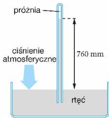
Rys. 7.24. Zasada działania barometru rtęciowego, 1000 \text{ hPa} \approx 760 \text{ mmHg}
