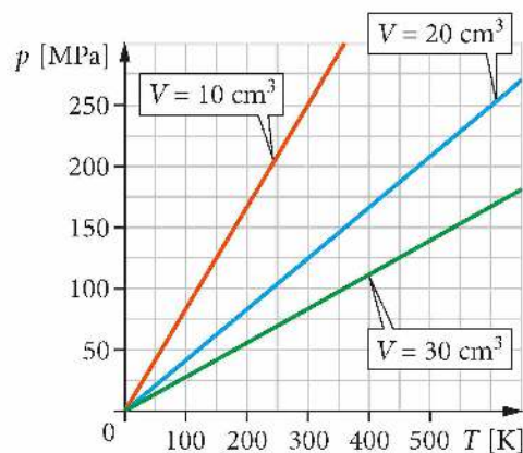
Rys. 8.5. Izochory – wykresy przedstawiające zależność ciśnienia 1 mola gazu od temperatury w przemianie izochorycznej. Każdy z wykresów dotyczy innej objętości
