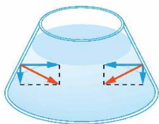
Rys. 7.19. Siły, którymi ścianki naczynia działają na wodę. Ich pionowa składowa powoduje dodatkowy nacisk wody na dno
