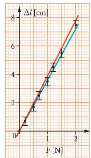
Rys. 9.22. Proste o największym (czerwona) i najmniejszym (niebieska) nachyleniu przechodzące przez punkty pomiarowe wraz z niepewnościami
