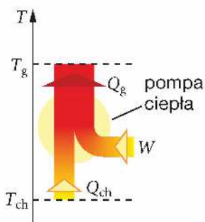
Rys. 8.28. Pompa ciepła działa odwrotnie niż silnik cieplny (por. rys. 8.25 s. 116)
