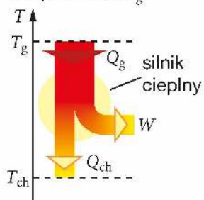
Rys. 8.25. Schemat silnika cieplnego
