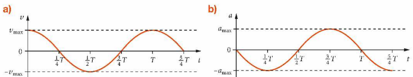
Rys. 9.13. Wykresy zależności a) prędkości od czasu, b) przyspieszenia od czasu dla ruchu drgającego
