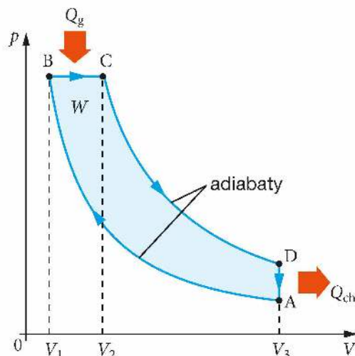
Rys. 8.34. Cykl w silniku Diesla
