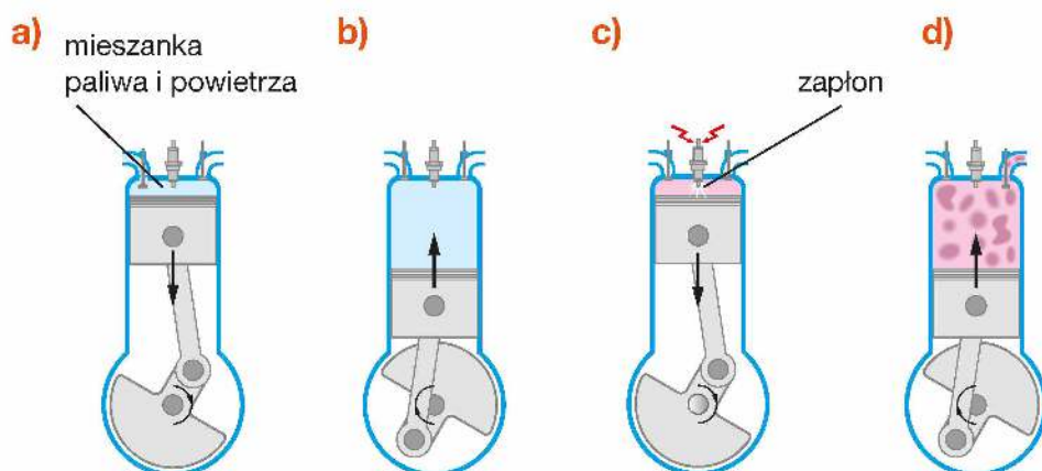
Rys. 8.31. Schemat działania benzynowego silnika czterosuwowego: a) suw ssania, b) suw sprężania, c) suw pracy, d) suw wydechu
