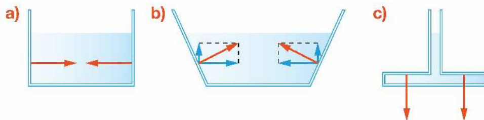
Rys. 7.18. Siły, którymi ścianki różnych naczyń działają na wodę. Jeżeli ścianki nie są pionowe, to siły te mają pionową składową
