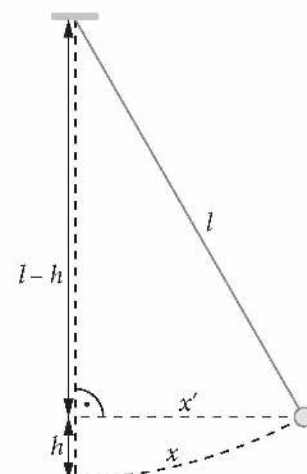
Rys. 9.34. Sposób obliczania wysokości, na jakiej znajduje się ciężarek wahadła
