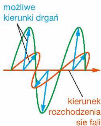
Rys. 10.5. Istnieje nieskończenie wiele kierunków prostopadłych do kierunku rozchodzenia się fali. Drgania w czasie rozchodzenia się fali poprzecznej mogą zachodzić w każdym z nich
