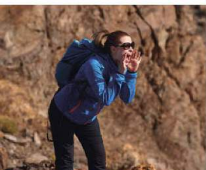
Rys. 10.27. Odbicie fali dźwiękowej dociera do nas jako echo
