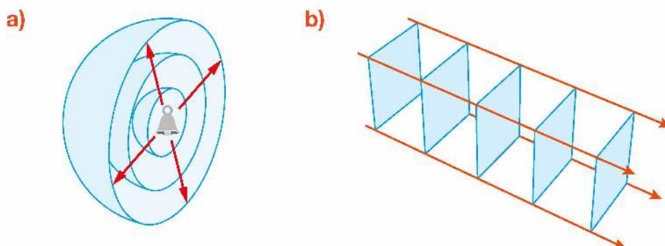
Rys. 10.25. Promienie i powierzchnie falowe a) kulistej fali dźwiękowej, b) fali płaskiej w przestrzeni
