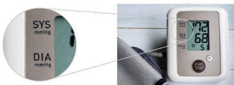
Rys. 7.25. Ciśnienie krwi mierzymy w mmHg
