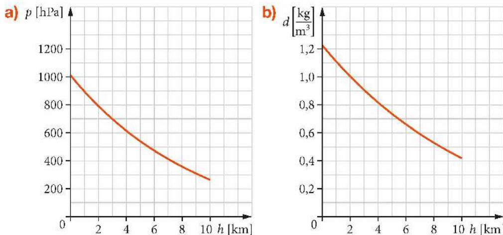
Rys. 7.21. Zależność a) ciśnienia atmosferycznego, b) gęstości powietrza od wysokości n.p.m.
