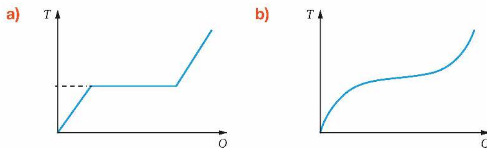
Rys. 7.49. Zmiany temperatury ciała w zależności od ilości dostarczonego ciepła dla a) kryształu, b) ciała bezpostaciowego
