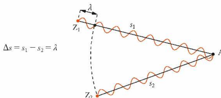
Rys. 10.38. Gdy drogi przebyte przez dwie fale różnią się o \lambda , fale spotykają się w tej samej fazie i się wzmacniają
