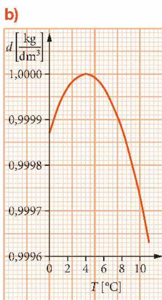
Rys. 7.58. a) objętość 1 kg wody w zależności od temperatury, b) gęstość wody w zależności od temperatury
