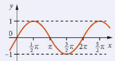
Rys. 9.8. Wykres funkcji y = \sin x
