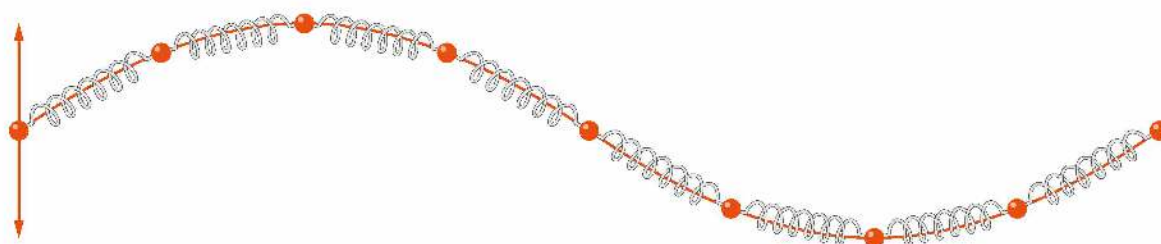
Rys. 10.4. Fala harmoniczna (widok z góry)
