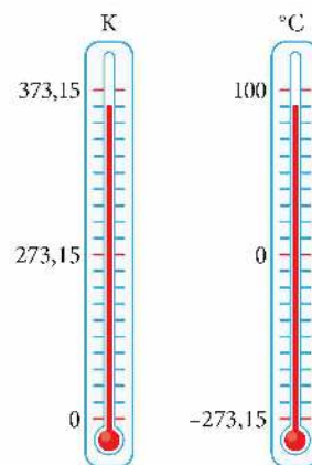
Rys. 7.34. Porównanie skal temperatur: Kelvina i Celsjusza
