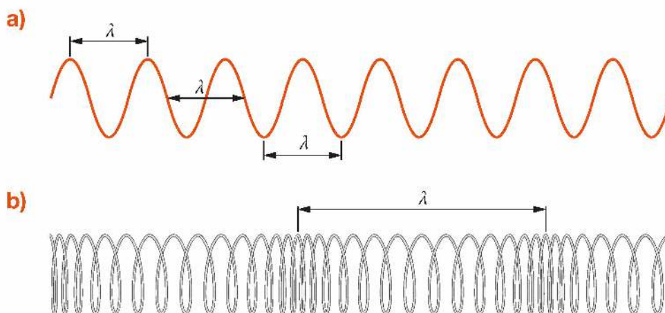
Rys. 10.13. Długość fali to odległość między sąsiednimi punktami, które drgają w tej samej fazie, np.: a) między dwoma sąsiednimi grzbietami, b) między dwoma kolejnymi zagęszczeniami zwojów
