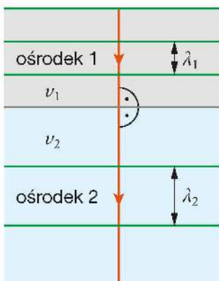
Rys. 10.32. Fala padająca prostopadle na granicę ośrodków
