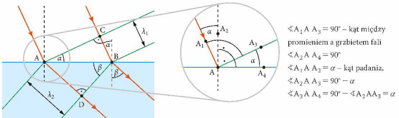
Rys. 10.31. Uzasadnienie prawa załamania
