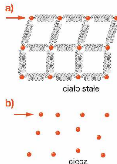
Rys. 10.10. Warstwy atomów oddziałują ze sobą w ciele stałym (a), ale nie w cieczy (b)
