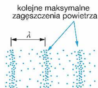
Rys. 10.19. Długość fali dźwiękowej
