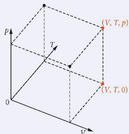
Rys. 8.12. Układ współrzędnych do rysowania wykresu funkcji dwóch zmiennych
