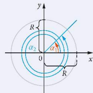
Rys. 9.7. Jeśli kąt jest większy od 2\pi , to przyjmujemy, że ramię kąta obróciło się o kąt pełny (być może wielokrotnie) i jeszcze o pewien kąt mniejszy od kąta pełnego
