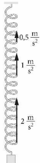
Rys. 9.24. Różne zwoje sprężyny poruszają się z różnymi przyspieszeniami
