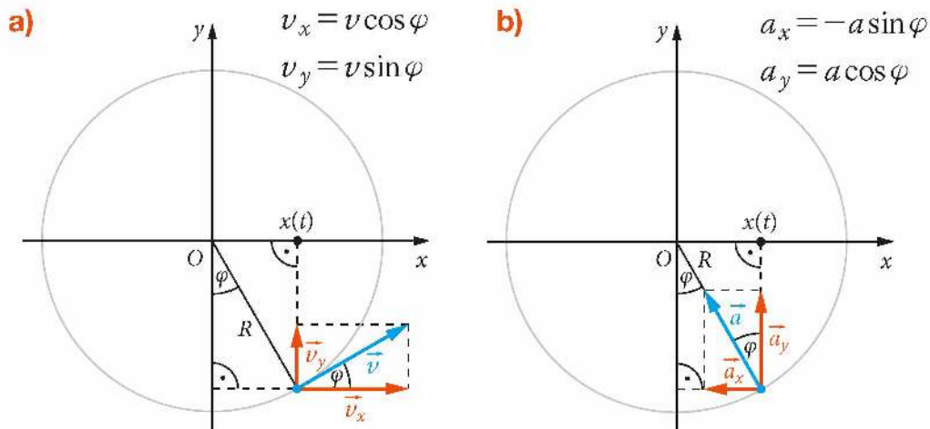
Rys. 9.12. Rozkład na składowe a) wektora prędkości liniowej, b) wektora przyspieszenia dośrodkowego w ruchu po okręgu
