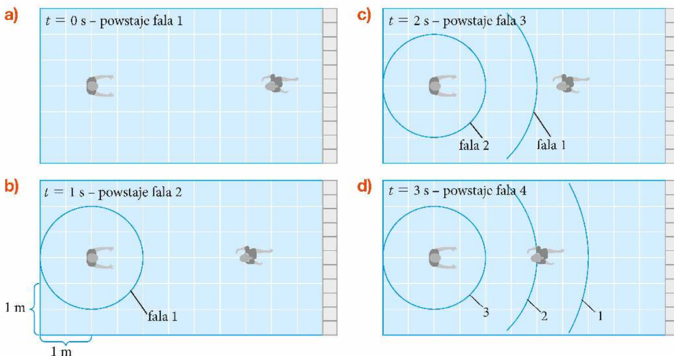
Rys. 10.59. Fala na wodzie i efekt Dopplera – obserwator zbliża się do nieruchomego źródła fali
