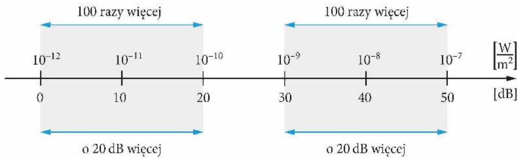
Rys. 10.61. Skala natężenia dźwięku
