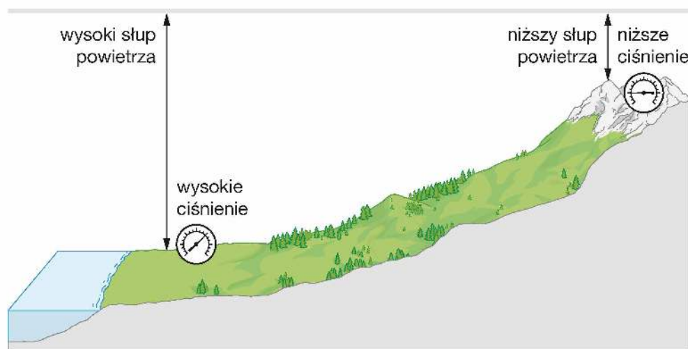
Rys. 7.20. W górach znajduje się nad nami niższy słup powietrza. Uwaga. Górna granica atmosfery została zaznaczona umownie
