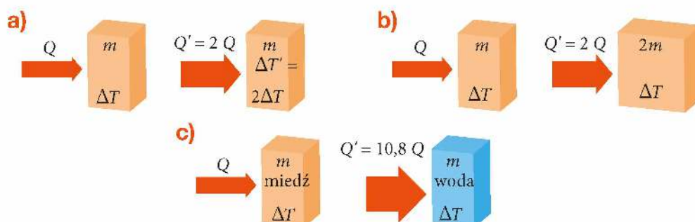
Rys. 7.43. Ilość ciepła potrzebna do zmiany temperatury zależy od: a) wielkości zmiany temperatury, b) ilości substancji, c) jej rodzaju
