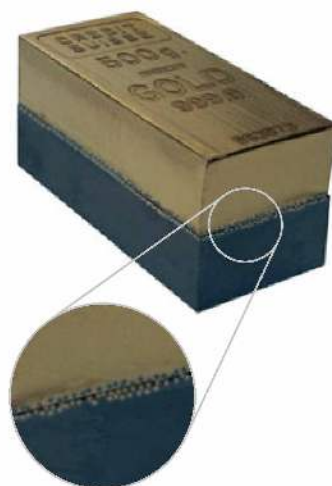
Rys. 7.37. Dyfuzja zachodzi także w ciałach stałych. W ciągu kilku lat część atomów złota przemieściła się do ołowiu i na odwrót
