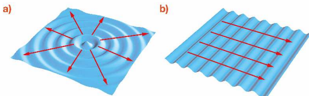
Rys. 10.24. Promienie fal na wodzie: a) kolistych, b) płaskich
