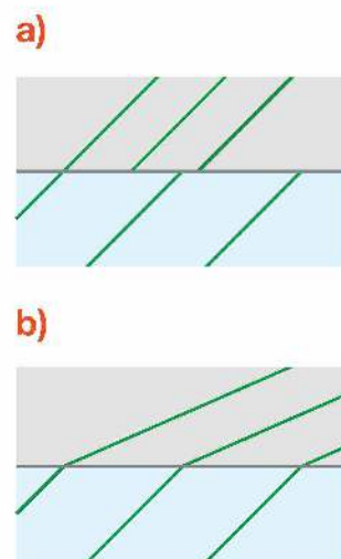
Rys. 10.30. Gdyby długość fali miała się zwiększyć bez zmiany kierunku, grzbiety fal musiałyby ulec przerwowaniu (a), ale grzbiety fal tworzą linie ciągłe (b)
