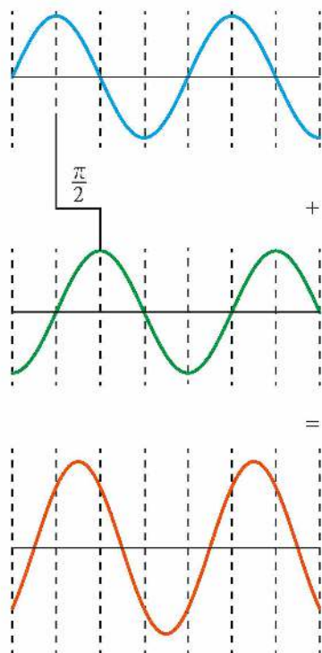
Rys. 10.37. Gdy dwie fale o tej samej amplitudzie, lecz przesunięte w fazie o \frac{\pi}{2} dochodzą do tego samego miejsca, mamy do czynienia z częściowym wzmocnieniem. Oznacza to, że amplituda fali wypadkowej jest większa od amplitudy każdej z fal składowych, ale mniejsza od sumy ich amplitud
