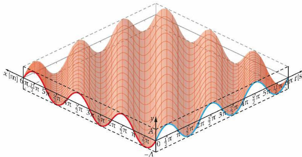
Rys. 10.14. Wykres funkcji falowej jako funkcji dwóch zmiennych y(x, t)
