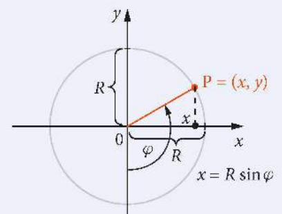
Rys. 9.9. Jeśli kąt mierzymy od osi y , to x = R \sin \varphi
