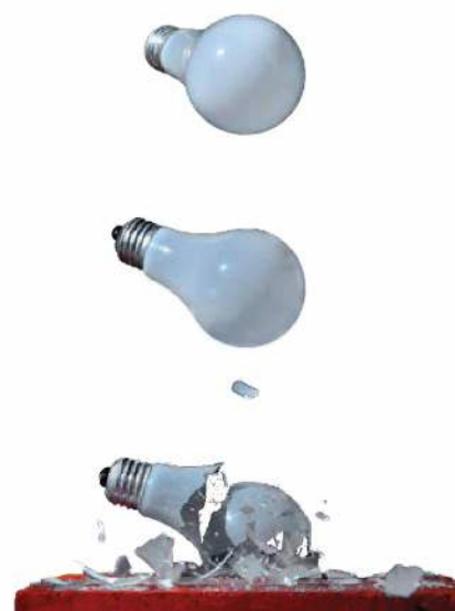
Rys. 8.37. Gdy widzimy tłukący się przedmiot, zawsze wiemy, jaka jest kolejność zdarzeń
