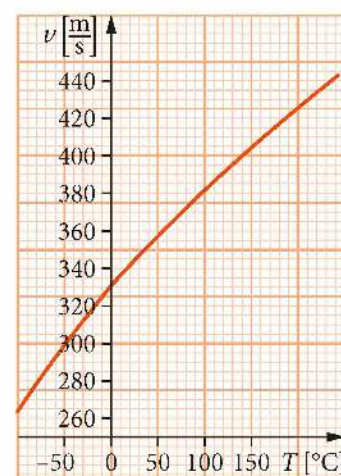
Rys. 10.22. Prędkość dźwięku w powietrzu zależy od temperatury powietrza
