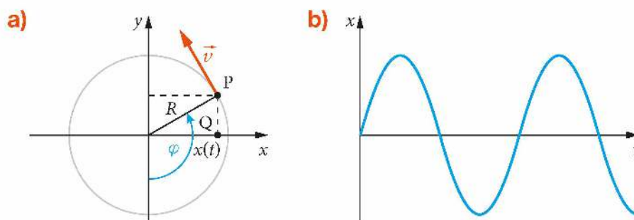
Rys. 9.5. a) punkt P porusza się po okręgu, a jego rzut Q porusza się po osi x ruchem drgającym, b) wykres ruchu punktu Q w funkcji czasu jest sinusoida
